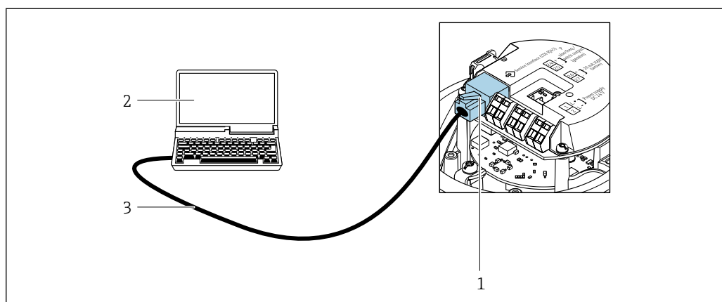
14 Подключение для кода заказа «Выход», опция В «4-20 мА HART, импульсный/частотный/релейный выход»
