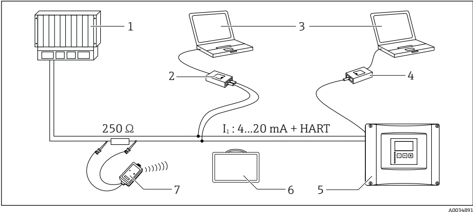
图 9 HART 系统集成
