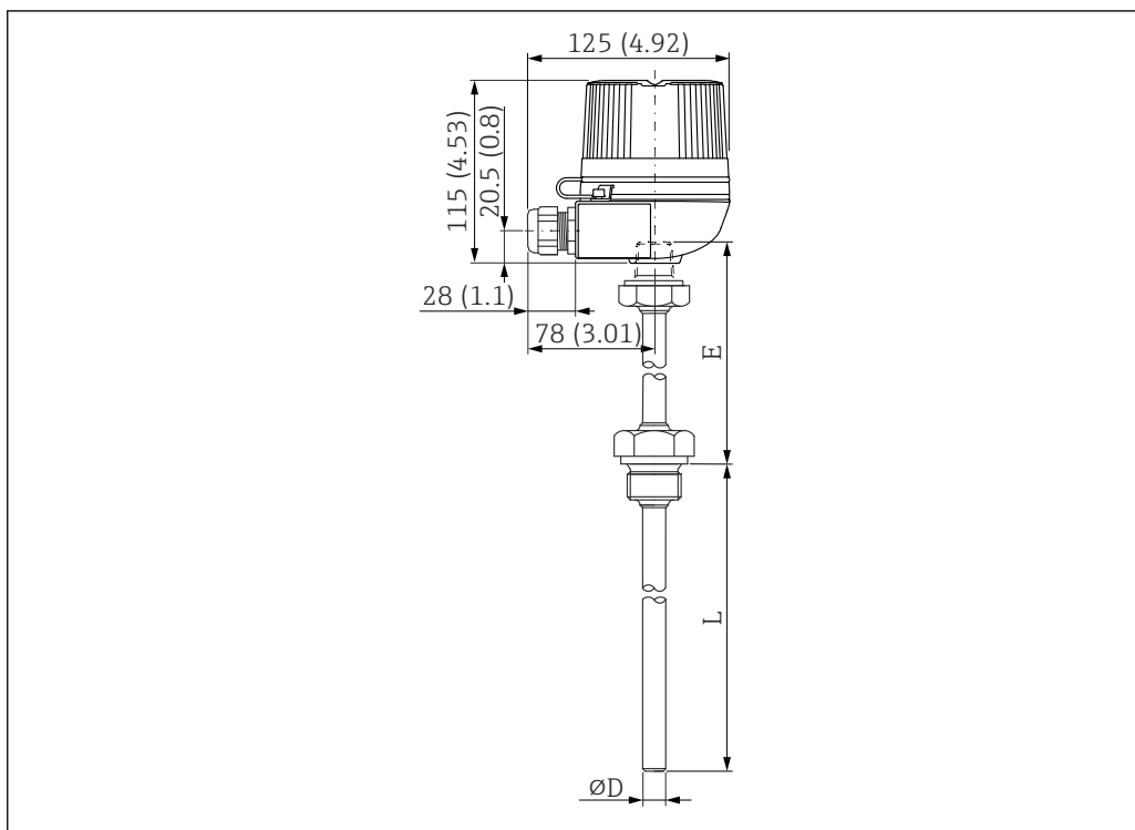
77 Struttura di Omnigrad S TR61; dimensioni: mm (in)
