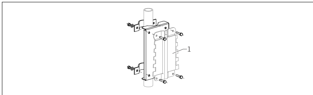
73 Piastra di montaggio della custodia da campo in polycarbonato
