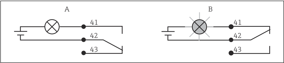
11 Empfohlene Fail-Safe-Schaltung für den Alarmkontakt
