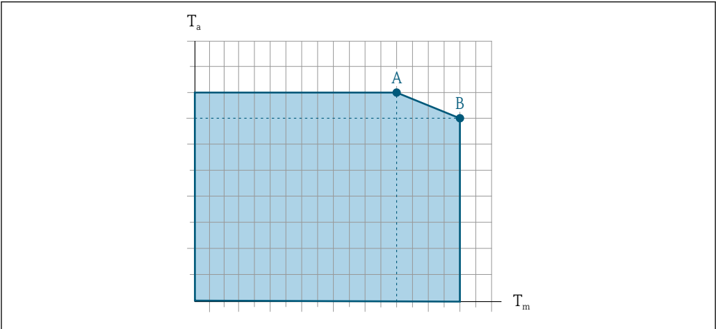
41 Пример зависимости, значения приведены в таблице. T_a Температура окружающей среды T_m Температура технологической среды A Максимально допустимая температура среды T_m при T_{a\,max} = 60\,^{\circ}\text{C} (140 °F); более высокие значения температуры технологической среды T_m требуют снижения температуры окружающей среды T_a B Максимально допустимая температура окружающей среды T_a при максимальной установленной температуре среды T_m для сенсора
