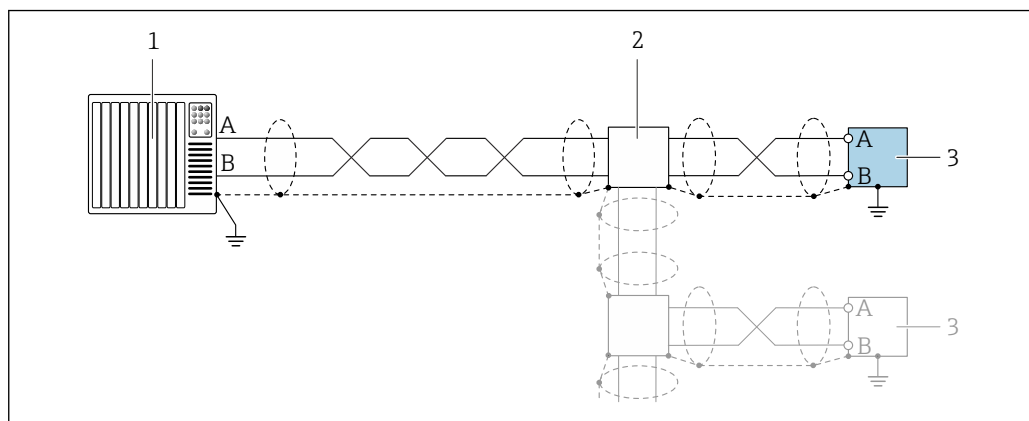
25 Пример подключения для Modbus RS485
