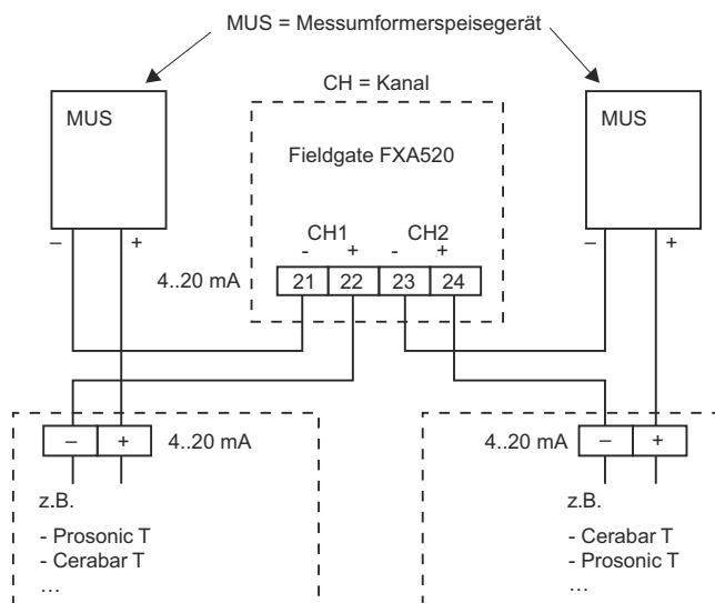
Abb. 4-12: Verdrahtung von 4...20 mA-Geräten
