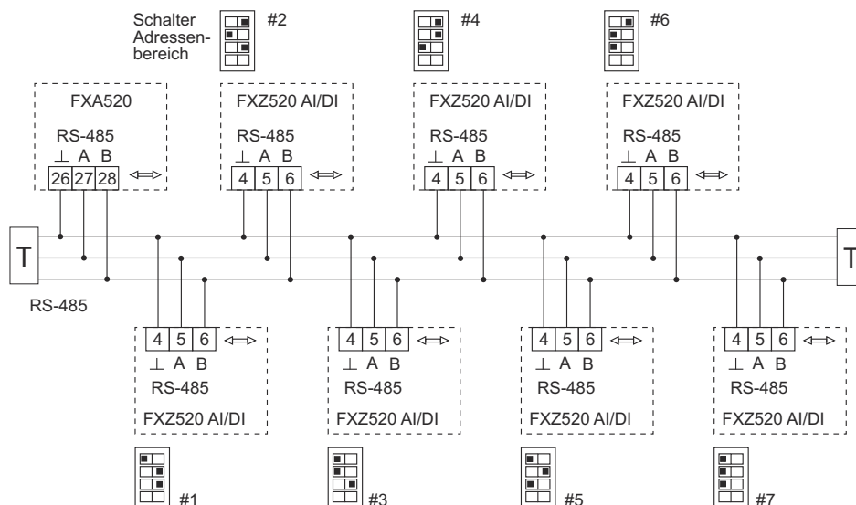
Abb. 4-13: Verdrahtung des RS 485-Busses: Jedes FXZ520 muss über eine eigene Adressbereichseinstellung verfügen
