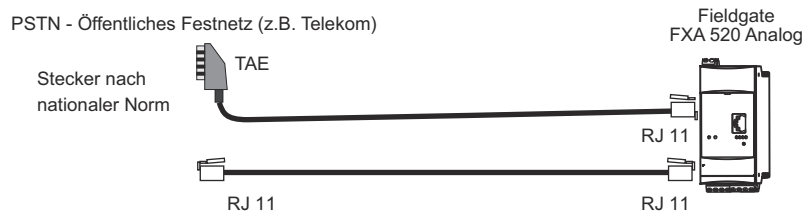
Abb. 4-14: Anschluss von Fieldgate ans leitungsvermittelte Telefonnetz
