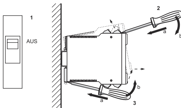
Abb. 4-4: Fieldgate von Hüttschiene lösen
