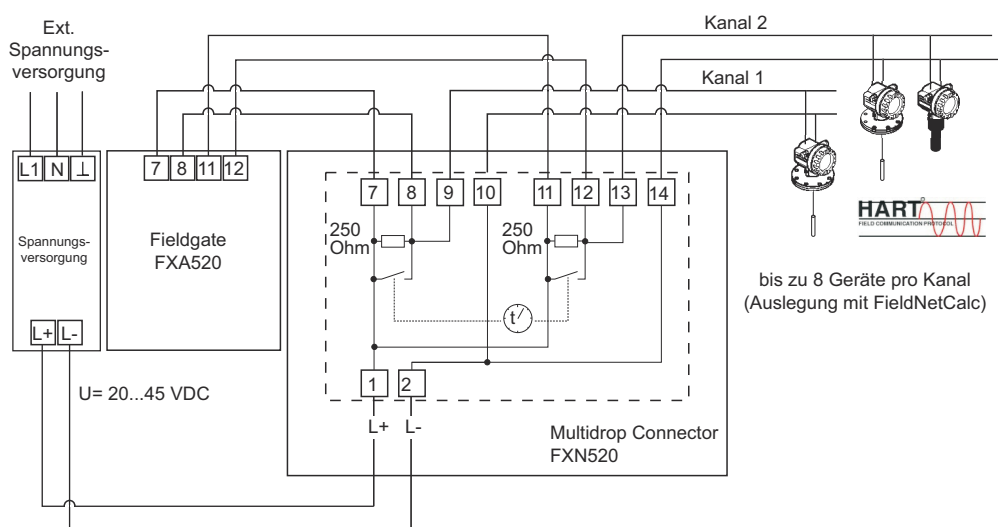
Abb. 4-9: Verdrahtung für HART-Multidrop mit FXN520
