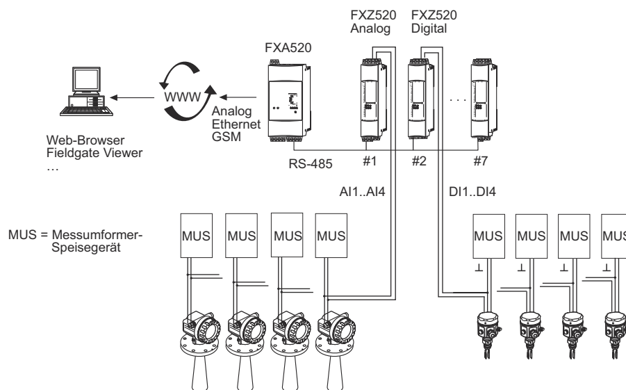
Abb. 3-11: Systemaufbau für FXZ520-Analog- und Digital-Eingangsmodule
