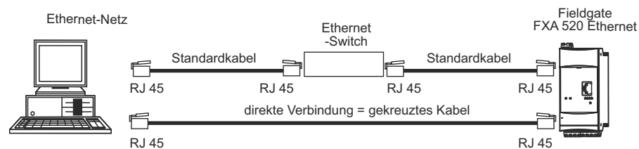
Abb. 4-15: Anschluss des Fieldgates an ein Ethernet-Netz
