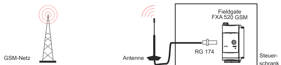
Abb. 4-16: Anschluss des Fieldgates an ein GSM-Netz
