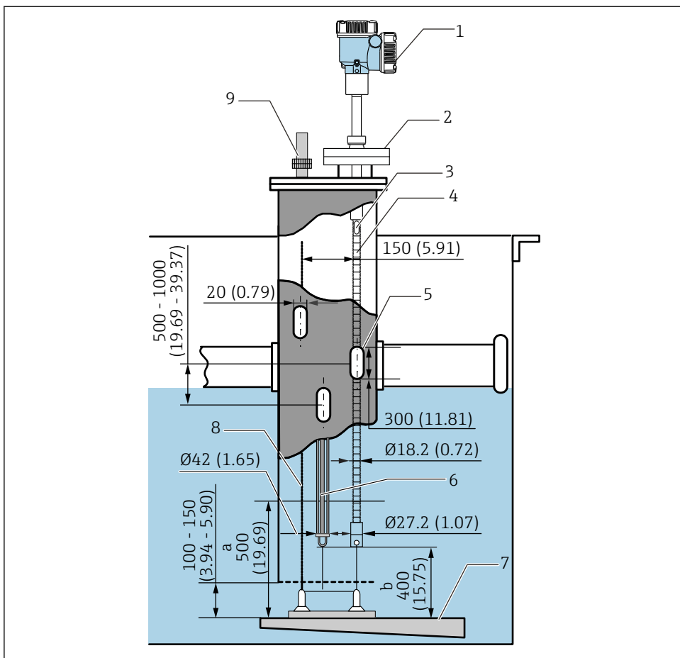
29 Método de anclaje superior. Unidad de medida mm (in)
