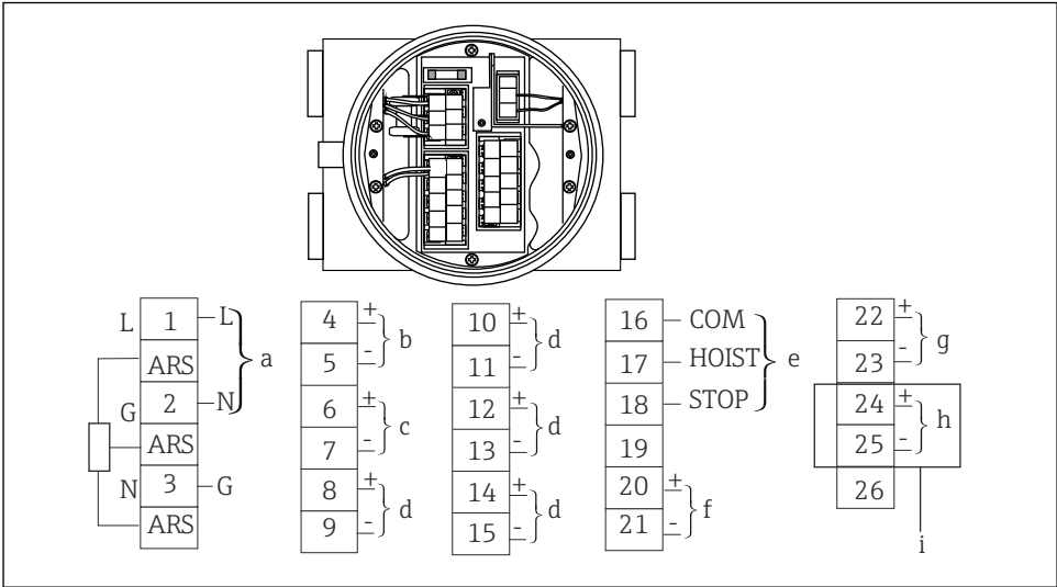
37 Terminal del NMS5
