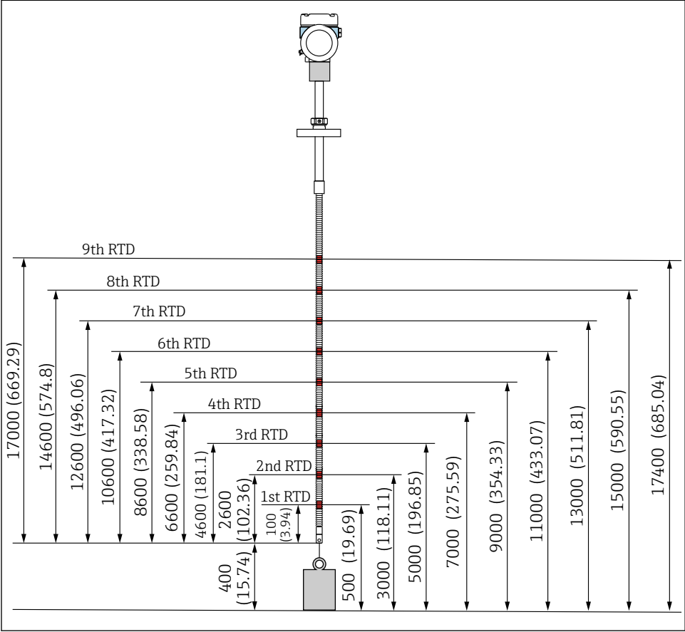
11 Posición del elemento. Unidad de medida mm (in)
