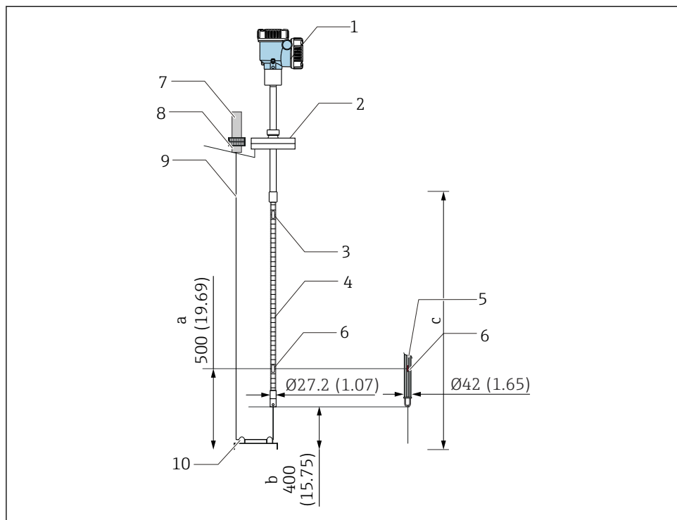
24 Método de anclaje superior. Unidad de medida mm (in)
