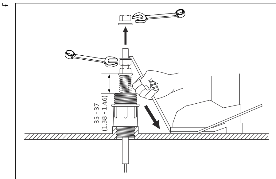
26 Instalación con anclaje superior 2. Unidad de medida mm (in)
