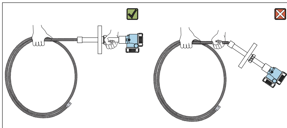
15 Desembalaje del NMT81
