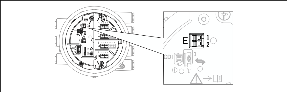
36 Terminal del NMS8x para el NMT81
