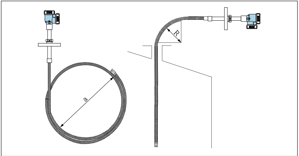
17 Instalación y enrollado de una sonda de temperatura
