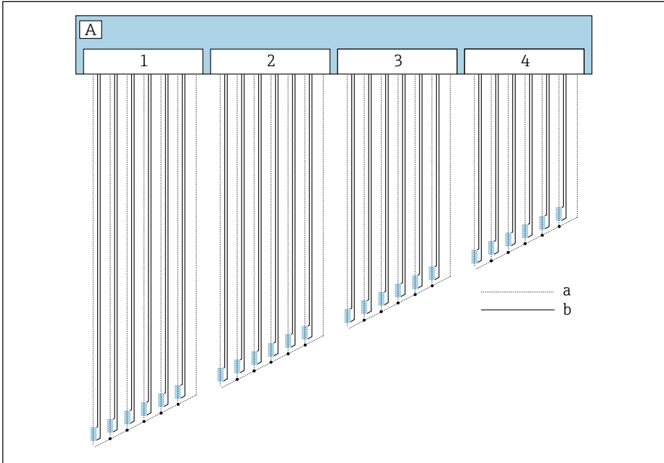
35 Esquema de conexión a cuatro hilos
