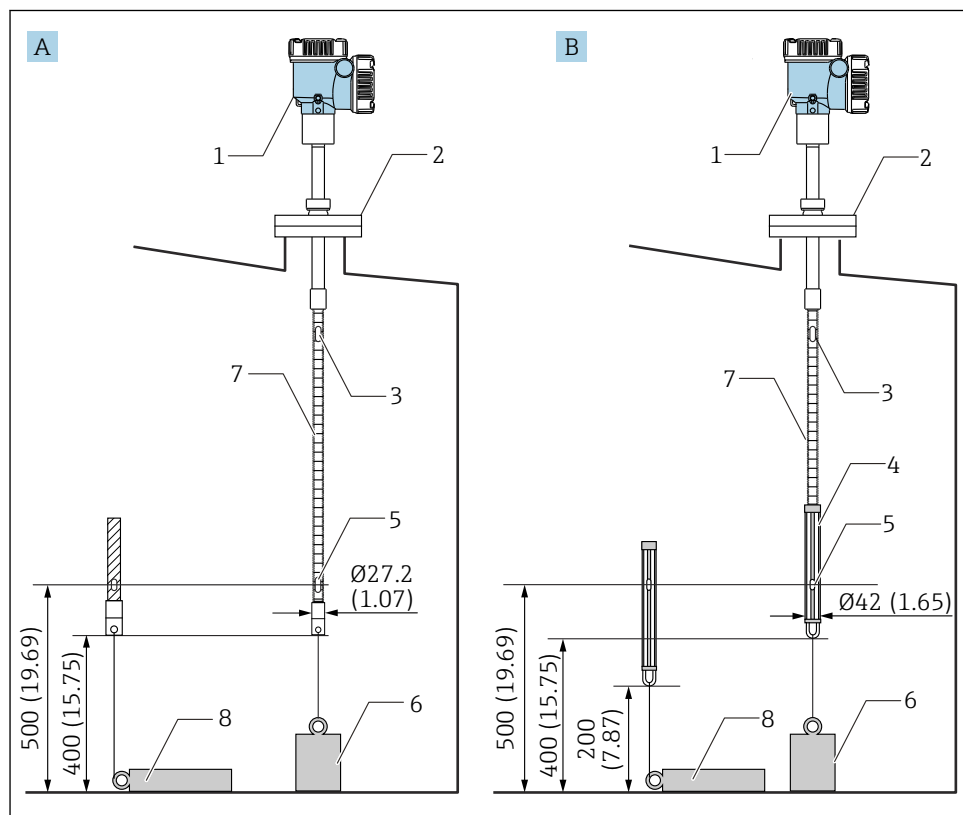
28 Método de contrapeso de anclaje. Unidad de medida mm (in)
