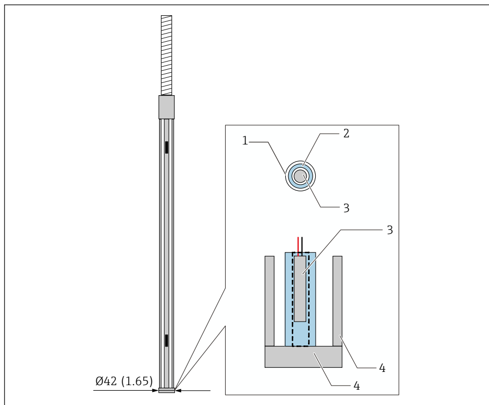
12 Diseño de la sonda de fondo de agua. Unidad de medida mm (in)
