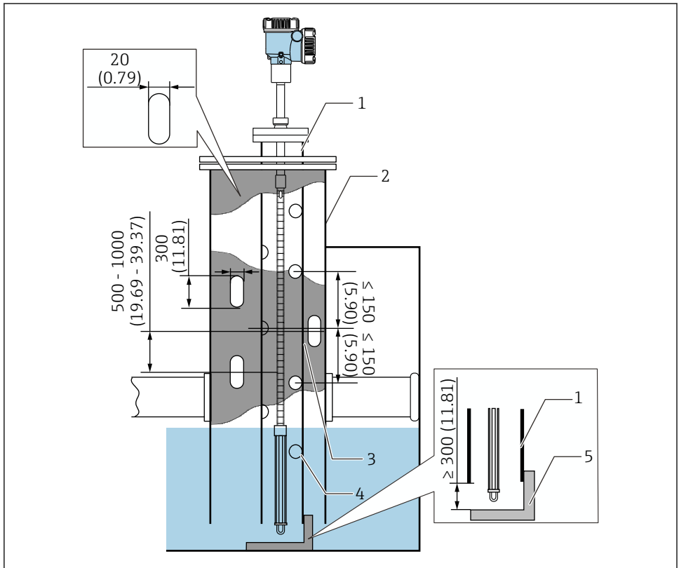
30 Método de tubo tranquilizador. Unidad de medida mm (in)
