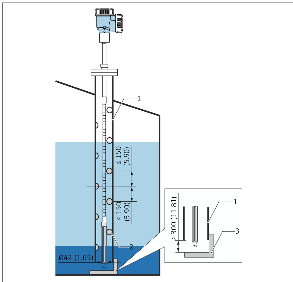
27 Tubo tranquilizador. Unidad de medida mm (in)
