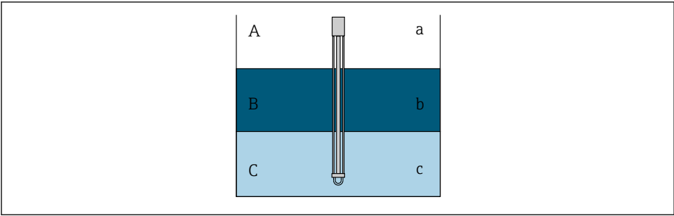
13 Medición de nivel de agua en tres capas
