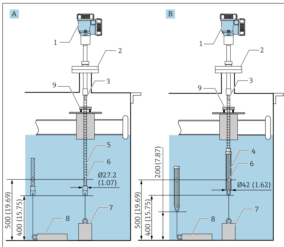
31 Método de anillo de guía y contrapeso de anclaje. Unidad de medida mm (in)
