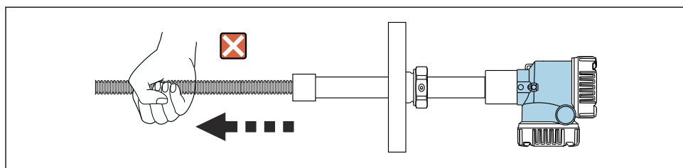
16 Manipulación de la sonda de temperatura
