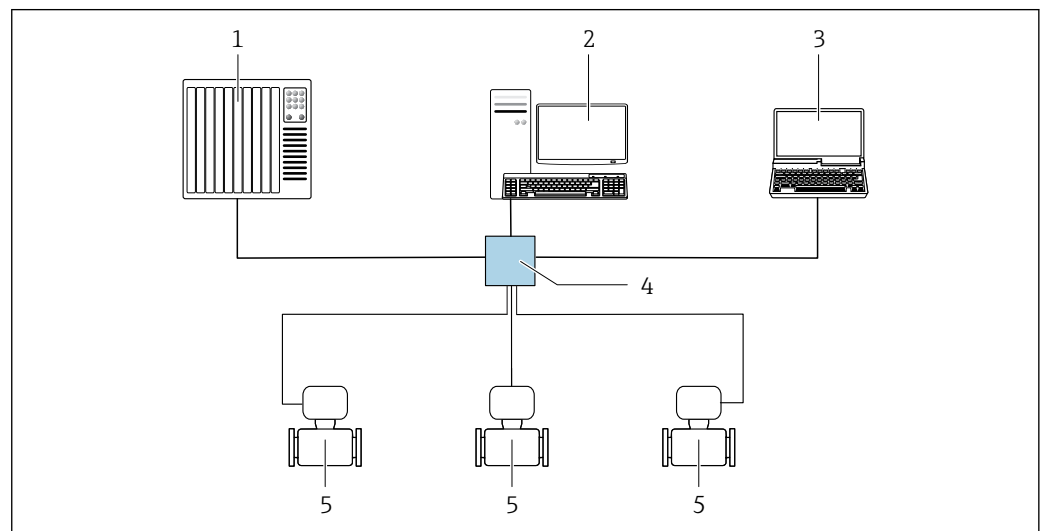
16 Options pour la configuration à distance via le réseau EtherNet/IP : topologie en étoile
