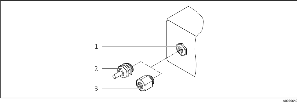
図 43 可能な電線口/ケーブルグラント 1 めねじ M20 × 1.5 2 ケーブルグラント M20 × 1.5 3 電線口用アダプタ (めねじ G ½" または NPT ½")
