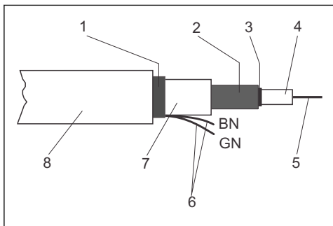
12 Structuur van kabel CMK
