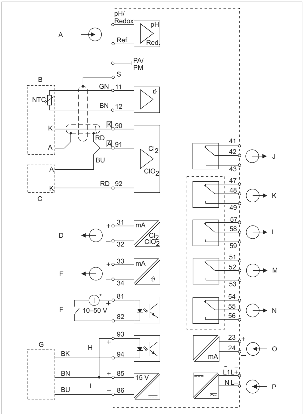
7 Elektrische aansluiting van de transmitter (versie 1)
