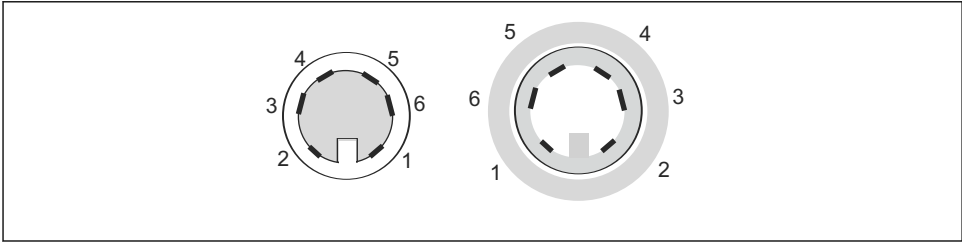
10 TOP68-aansluiting, pinbezetting van connector en koppeling (gezien vanaf contactzijde)
