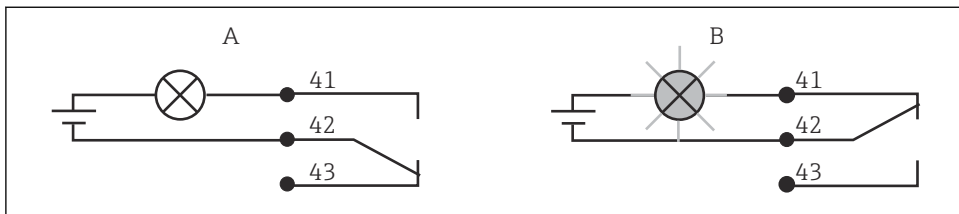
14 Aanbevolen fail-safe schakeling voor het alarmcontact
