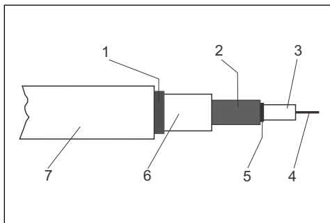
13 Structuur van kabel CYK71
