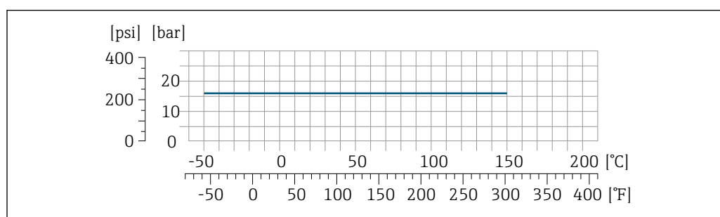
22 Con materiale connessione titanio grado 2
