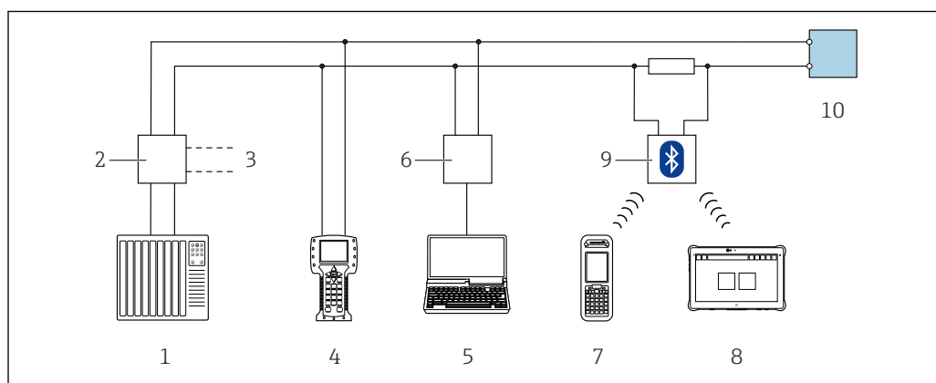
38 Opzioni per funzionamento a distanza mediante protocollo HART (passivo)
