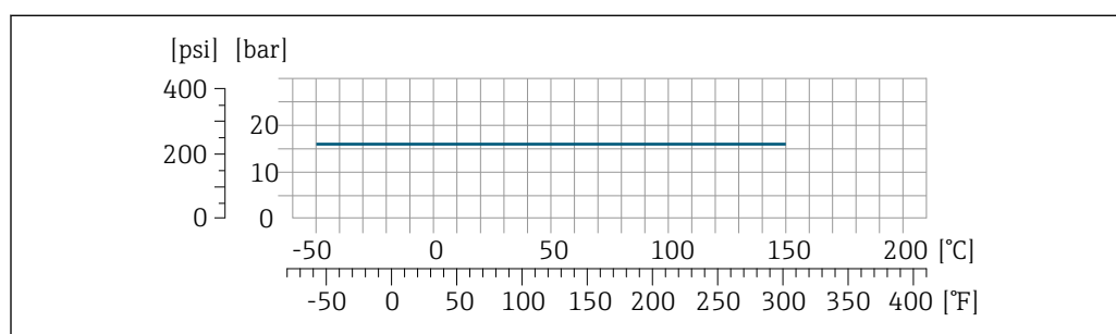
23 Con materiale connessione titanio grado 2
