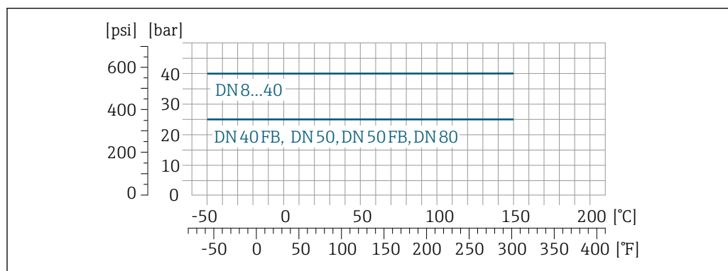
21 Con materiale connessione titanio grado 2
