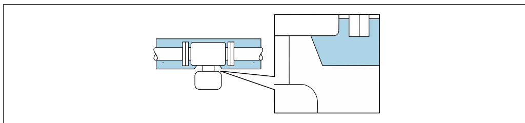
24 Coibentazione con collo esteso a vista
