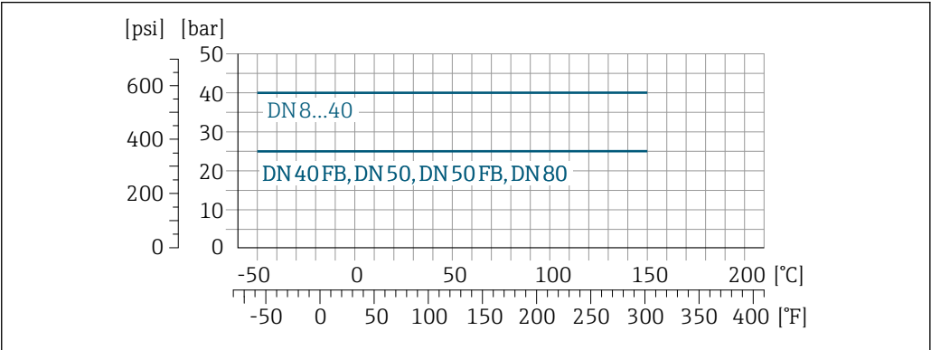
20 Con materiale connessione titanio grado 2
