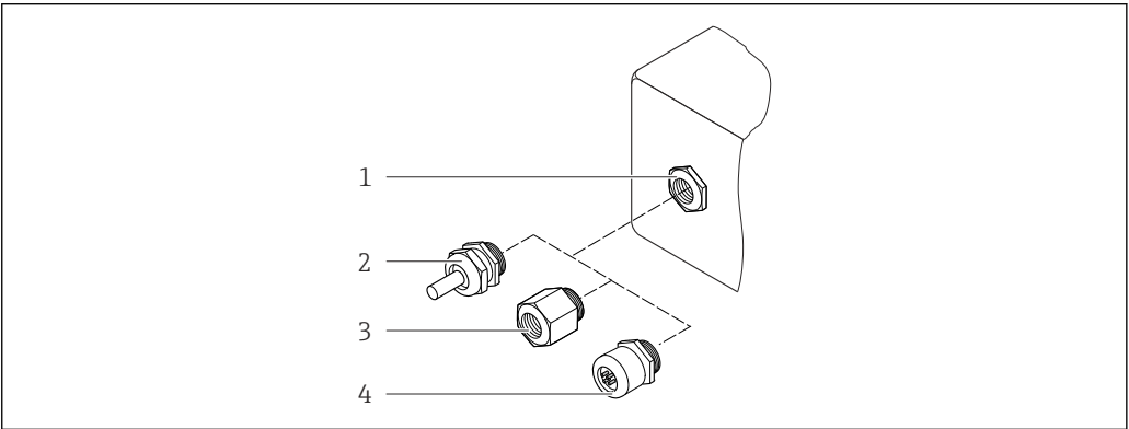
34 Possibilità di ingressi cavo/pressacavi
