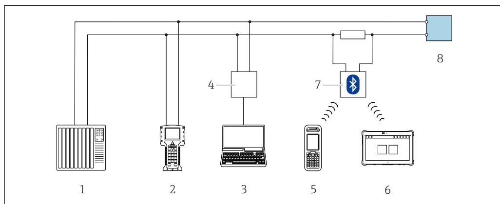
37 Opzioni per funzionamento a distanza mediante protocollo HART (attivo)
