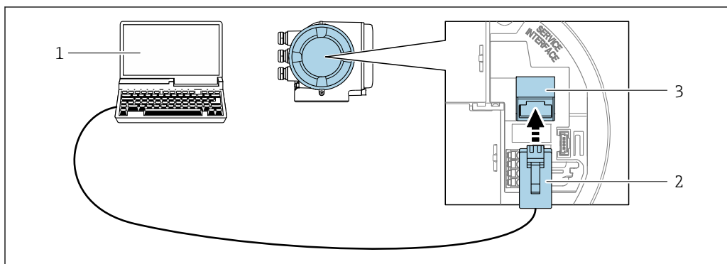
49 Connessione mediante interfaccia service (CDI-RJ45)
