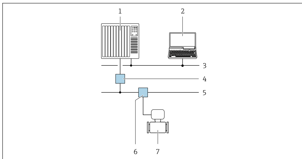
25 Варианты дистанционного управления по сети PROFIBUS PA
