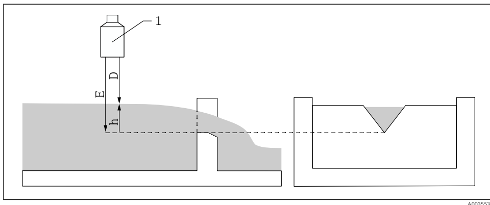
11 Étalonnage "vide" pour déversoirs
