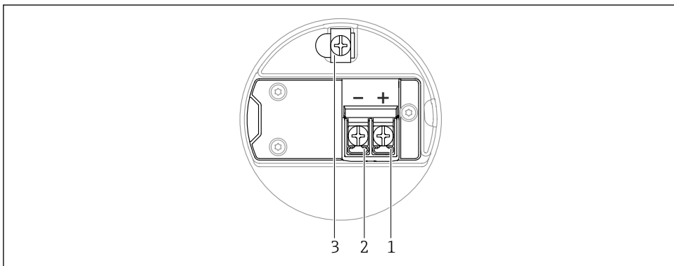
图 1 接线腔中的接线端子和接地端
