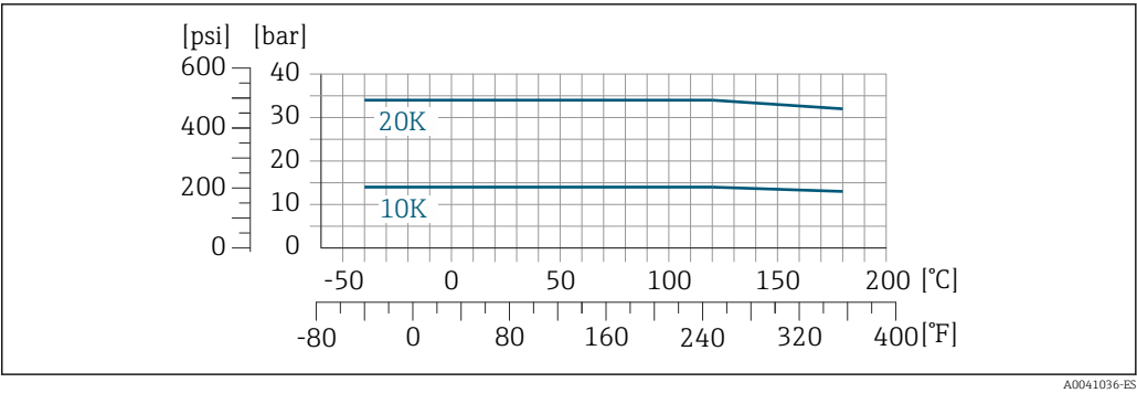
20 Material de la conexión bridada: acero inoxidable, múltiples certificaciones, 1.4404/F316/F316L
