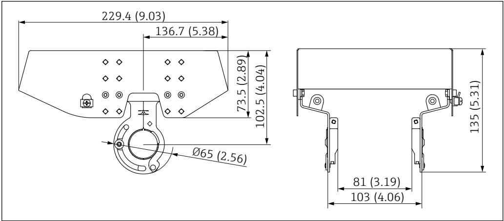
38 Capot de protection climatique. Unité de mesure mm (in)
