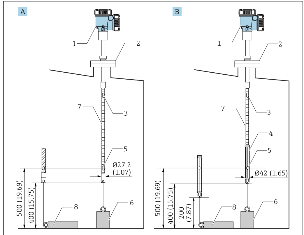
20 Méthode du poids d'ancrage. Unité de mesure mm (in)
