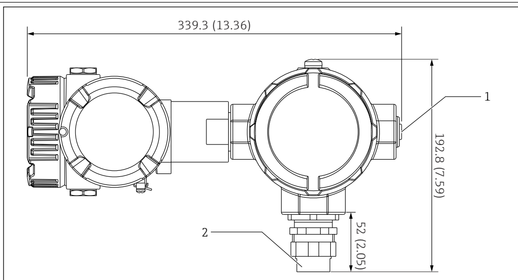
27 Option 1 : Convertisseur (raccord universel G3/4 (NPT 3/4) standard). Unité de mesure mm (in)
