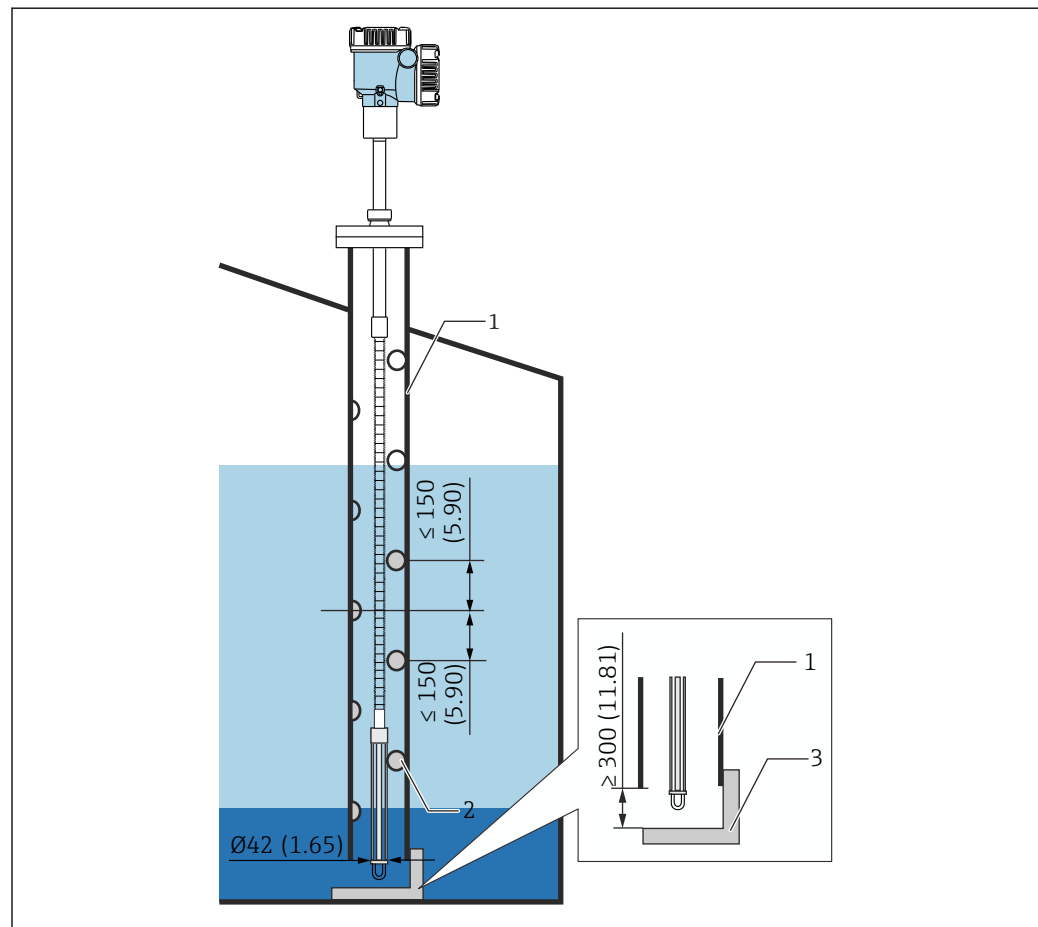
15 Tube de mesure. Unité de mesure mm (in)
