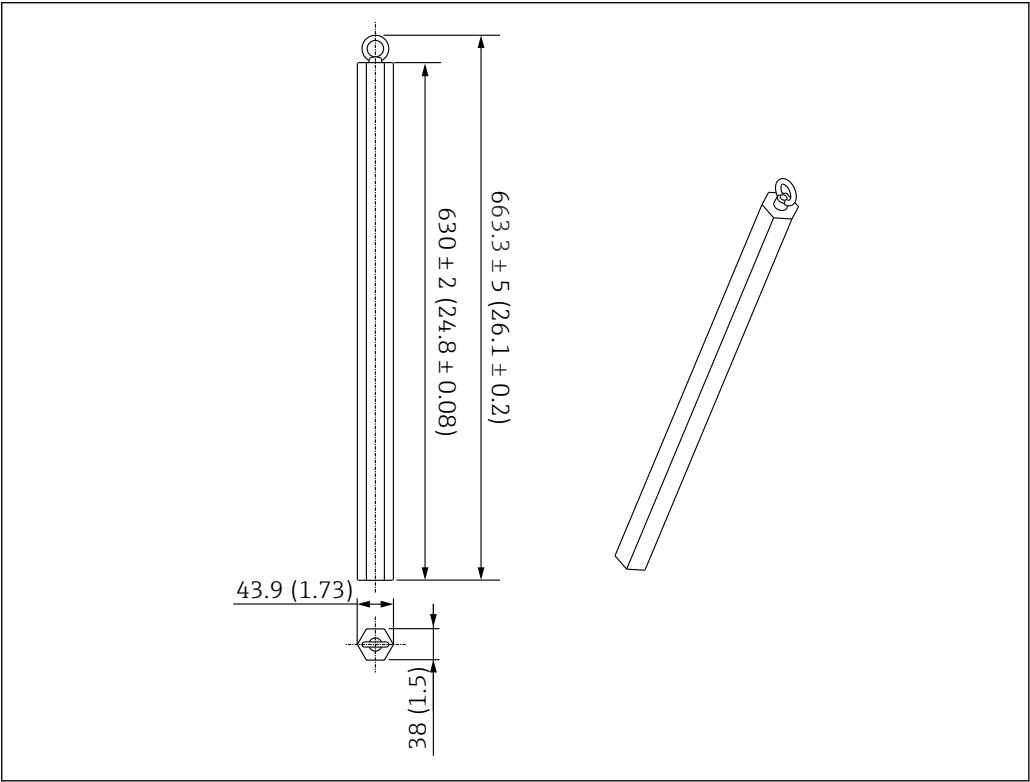
40 Accessoire de montage. Unité de mesure mm (in)
