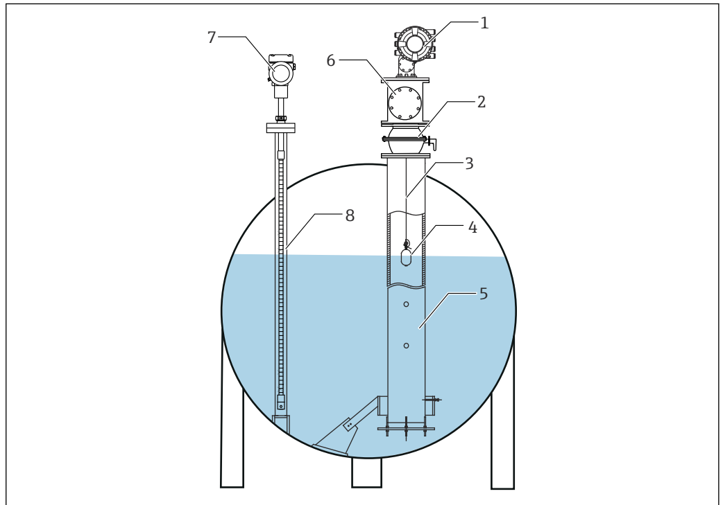
24 Protecteur pour une cuve sous pression
