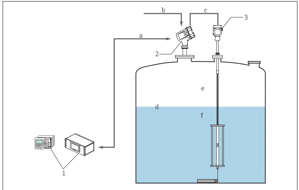
3 Combinaison NMT81 Ex ia et NMR8x
