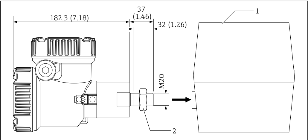
28 Option 2 : Convertisseur (Varec 1700, raccord fileté M20). Unité de mesure mm (in)
