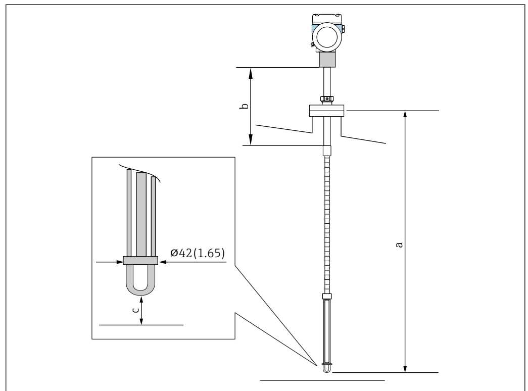
14 Montage recommandé. Unité de mesure mm (in)
