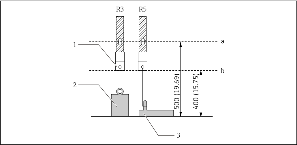
16 Accessoire de montage 1 (convertisseur + sonde de température). Unité de mesure mm (in)
