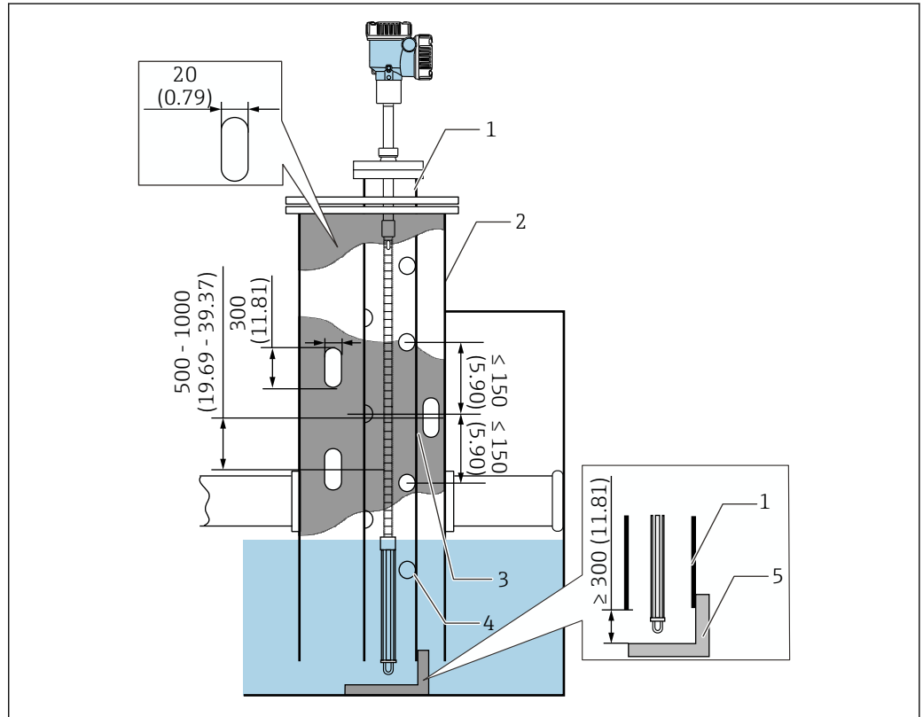
22 Méthode du tube de mesure. Unité de mesure mm (in)
