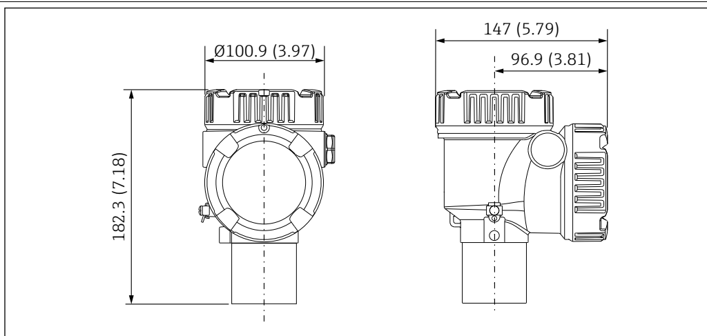
26 Convertisseur standard. Unité de mesure mm (in)
