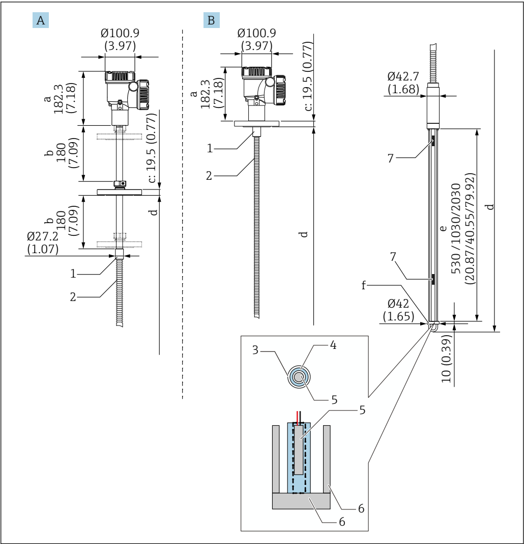
30 Convertisseur + sonde de température + sonde de fond d'eau. Unité de mesure mm (in)
