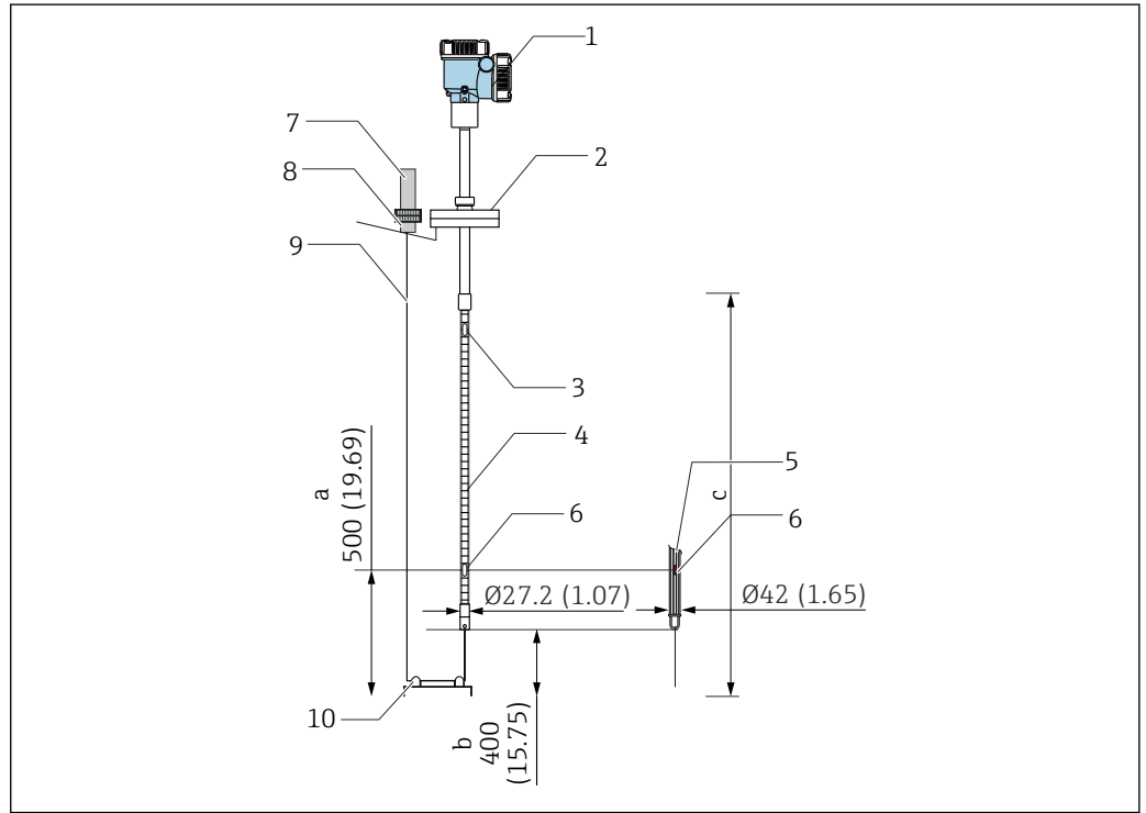
18 Méthode de l'ancrage supérieur. Unité de mesure mm (in)
