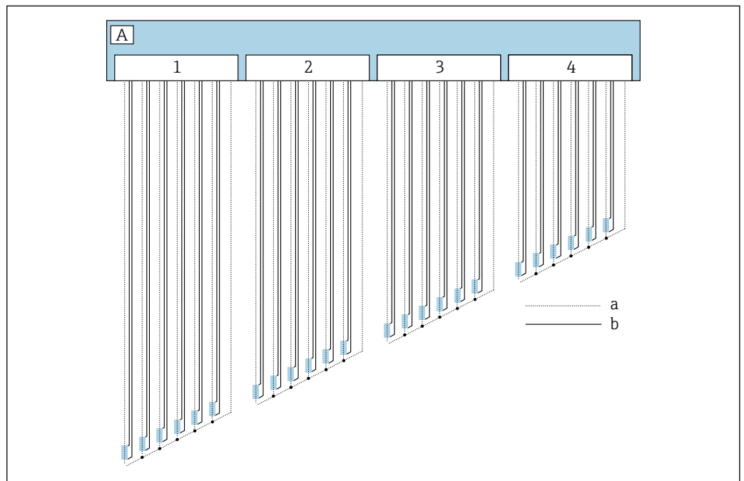
6 Schéma de raccordement à 4 fils
