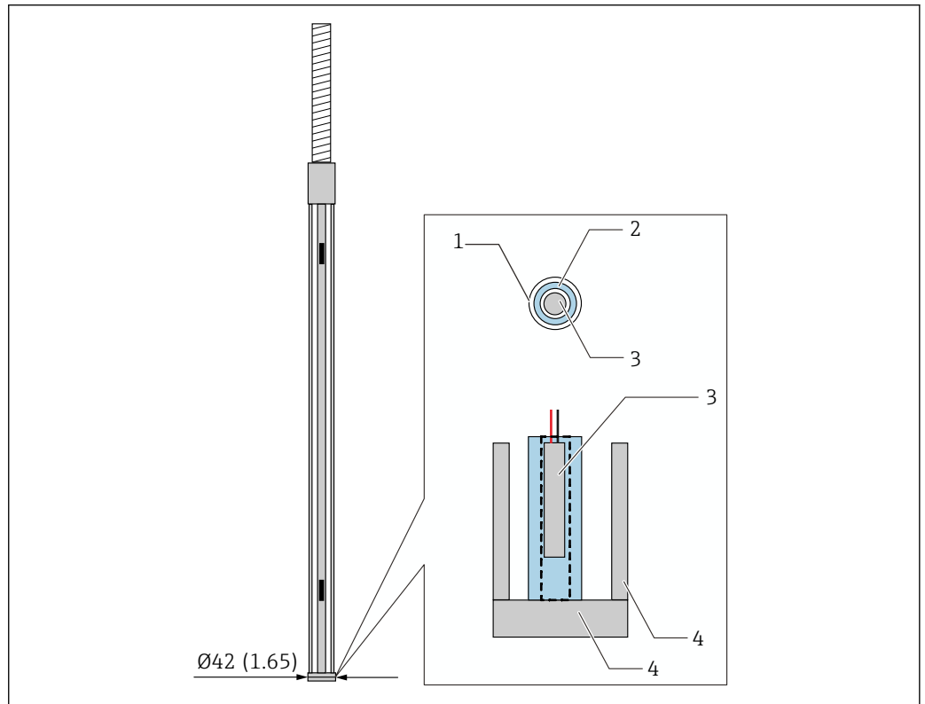
33 Construction de la sonde WB. Unité de mesure mm (in)
