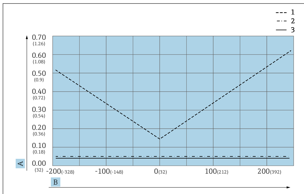
11 Précision totale, gammes de température haute et basse, unité de température en degré °C (°F)
