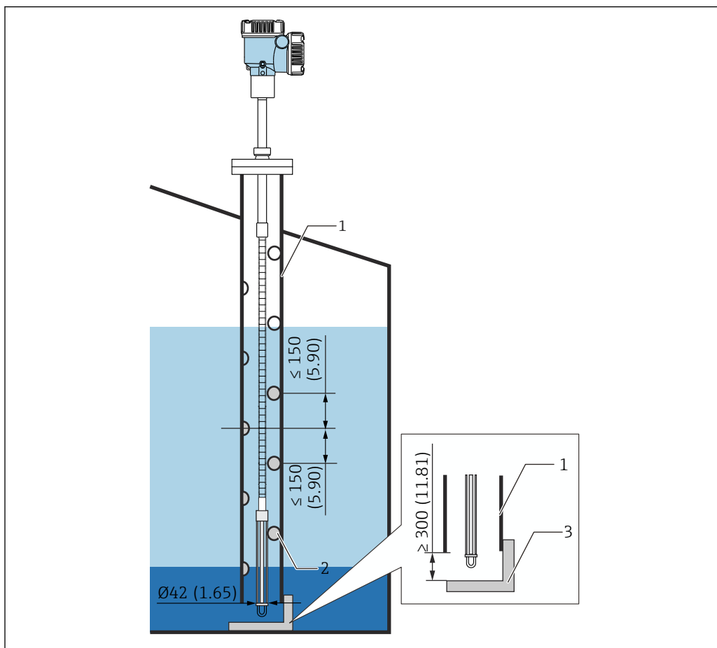
19 Tube de mesure. Unité de mesure mm (in)
