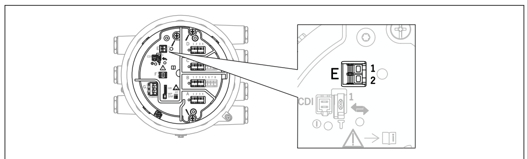
7 Bornes du NMS8x pour le NMT81
