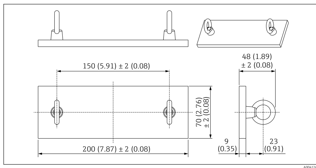
42 Crochet. Unité de mesure mm (in)
