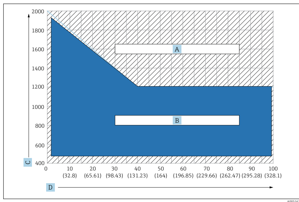
41 Tableau de sélection du poids d'ancrage, C : Unité de densité [kg/m³], D : Unité de longueur m / (ft)
