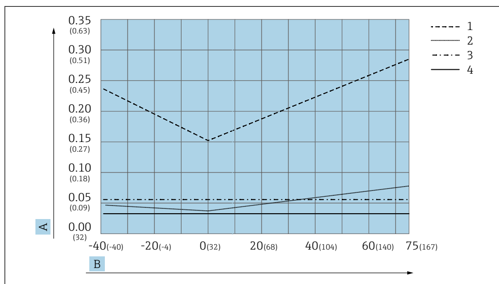
10 Précision totale, gammes de température standard, unité de température en degré °C (°F)
