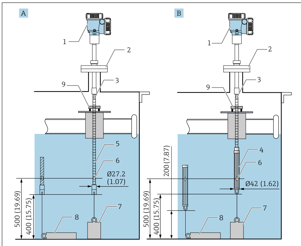
23 Méthode de la bague de guidage et du poids d'ancrage. Unité de mesure mm (in)
