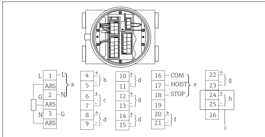
8 Bornes du NMS5
