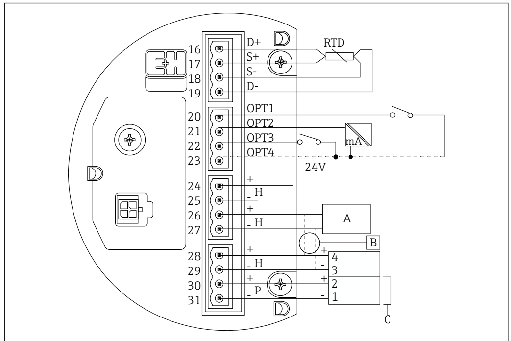
9 Bornes (à sécurité intrinsèque) du NRF590
