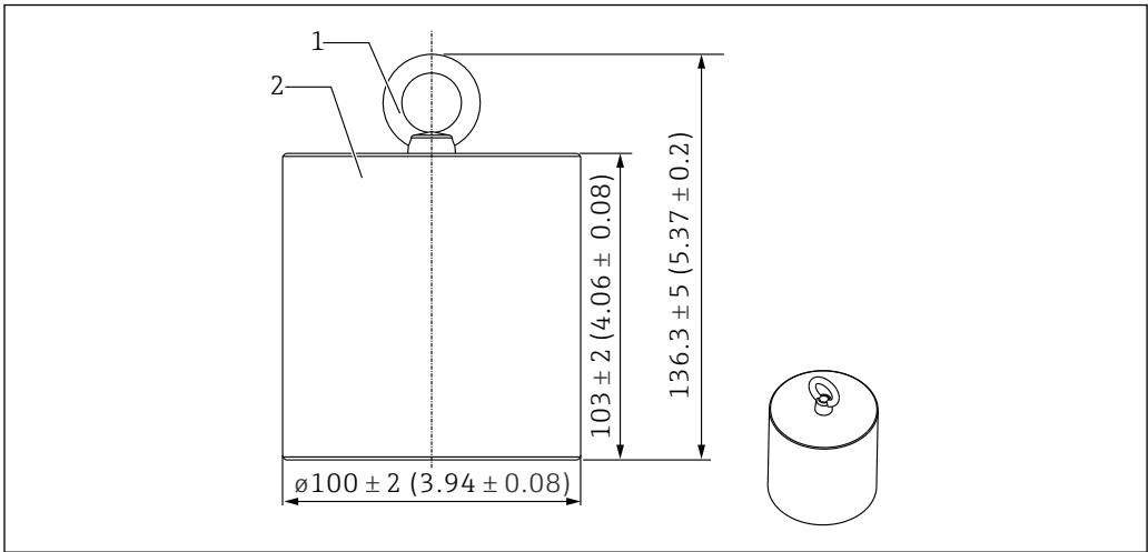
39 Accessoire de montage. Unité de mesure mm (in)
