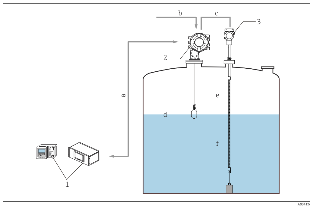
2 Construction du système NMS8x et NMT81
