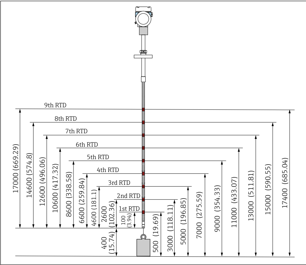
13 Position d'élément. Unité de mesure mm (in)
