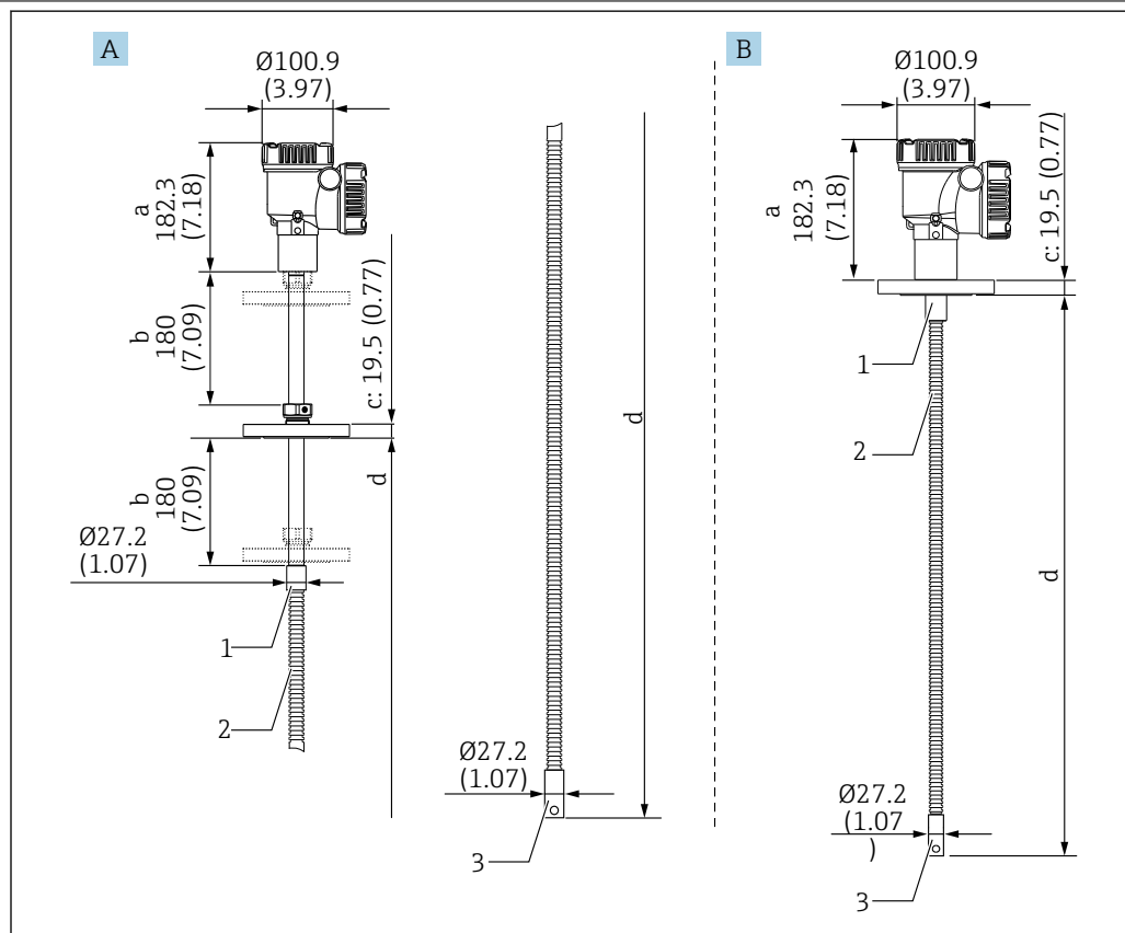
29 Convertisseur + sonde de température moyenne. Unité de mesure mm (in)
