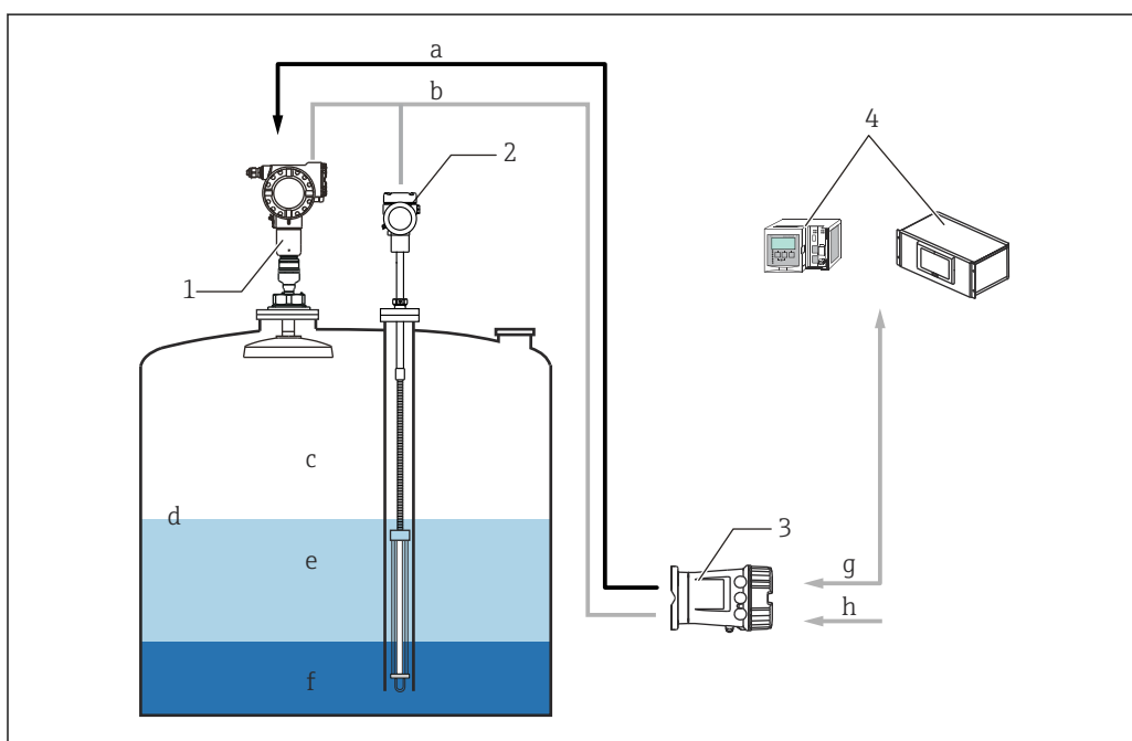
4 Combinaison NMT81 Ex ia et NRF Ex d [ia]
