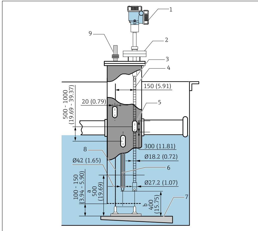
21 Méthode de l'ancrage supérieur. Unité de mesure mm (in)
