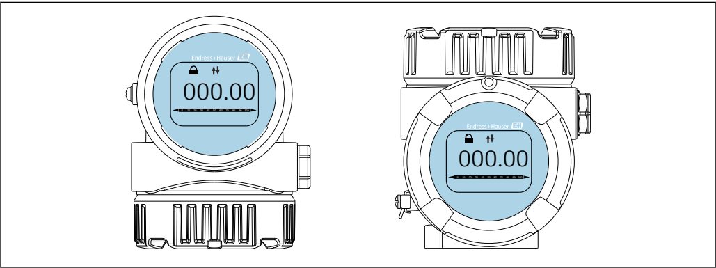
37 Position de l'afficheur : dessus (à gauche) ou côté (à droite)
