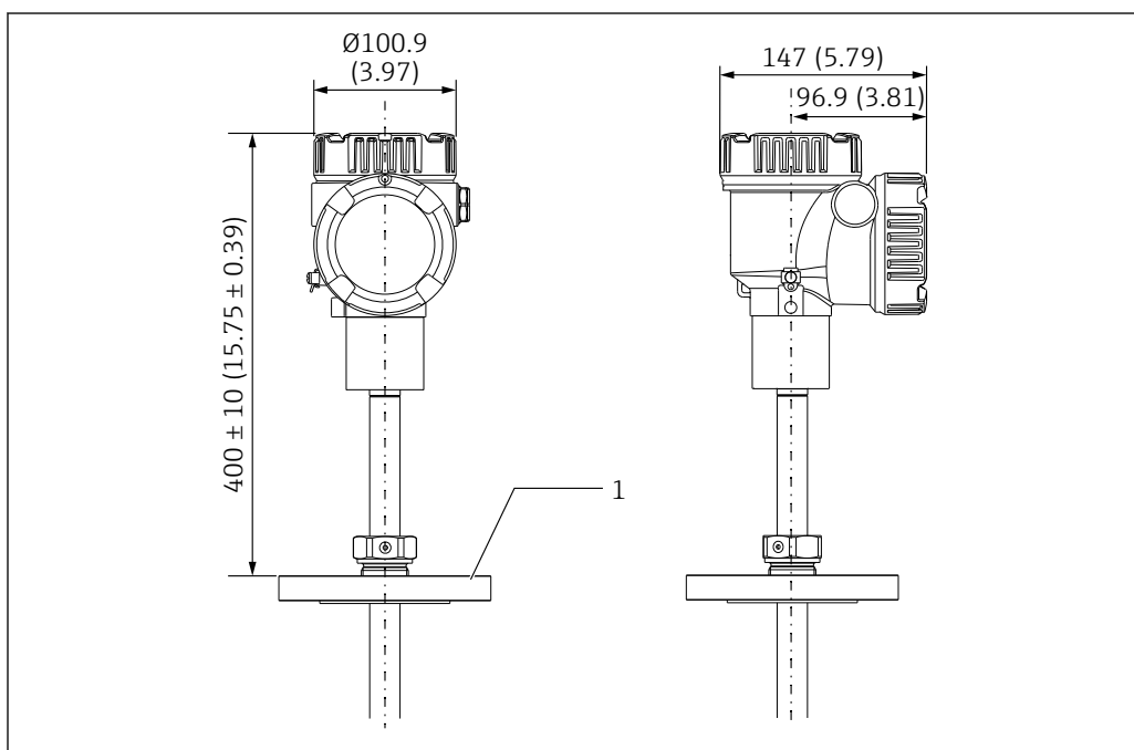
32 Bride coulissante. Unité de mesure mm (in)
