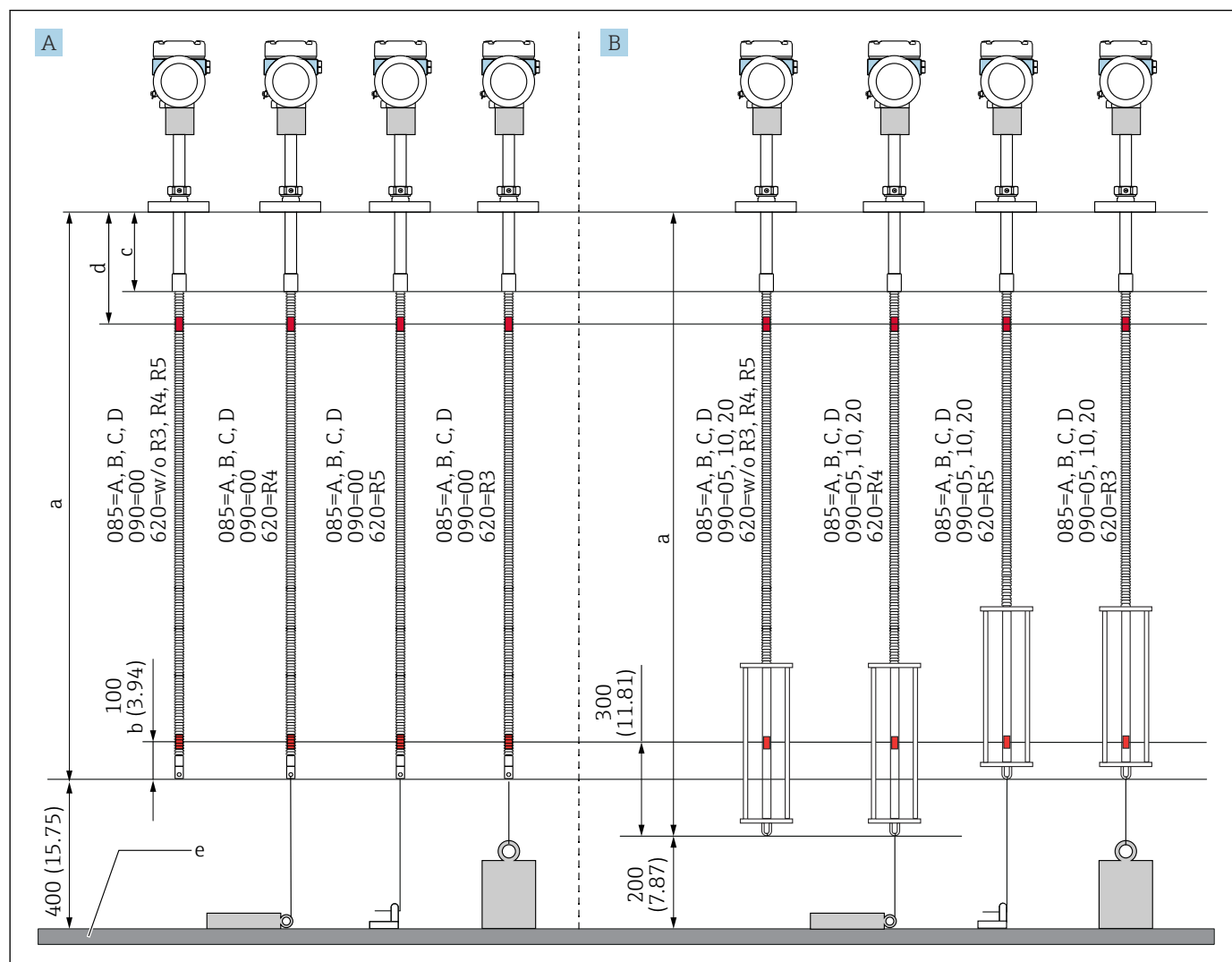
12 Position de l'élément n° 1 du NMT81 selon la méthode de montage. Unité de mesure mm (in)
