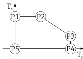
■ 15 Kunststoffgehäuse; Prozesstemperatur 0 \dots +80 \text{ °C} ( +32 \dots +176 \text{ °F} ) bei CSA C/US Zulassung
