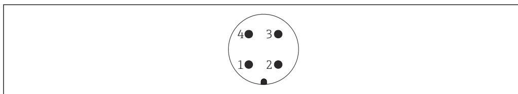
7 Sicht auf die Steckverbindung am Gerät
