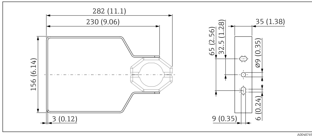
67 Abmessungen; Montagebügel ausrichtbar FMR6xB. Maßeinheit mm (in)
