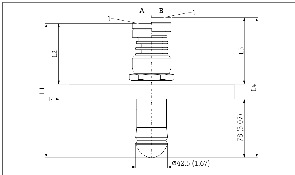
52 Abmessungen Drip-off Antenne 50 mm (2 in), Prozessanschluss UNI-Flansch. Maßeinheit mm (in)
