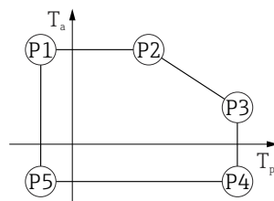
27 Gehäuse Aluminium, beschichtet; Prozesstemperatur -40 \dots +200 \text{ }^{\circ}\text{C} ( -40 \dots +392 \text{ }^{\circ}\text{F} )
