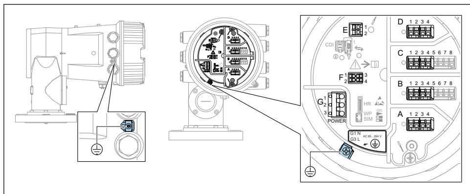
8 Priključni prostor (tipičen primer) in ozemljitvene sponke
