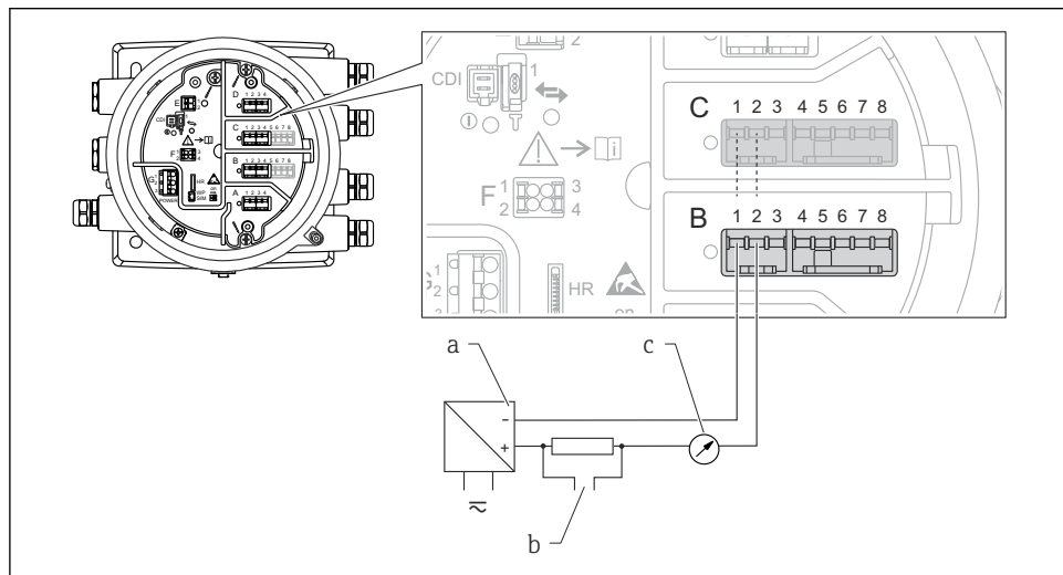
12 Pasivna uporaba analognega vhodno/izhodnega modula v izhodnem načinu
