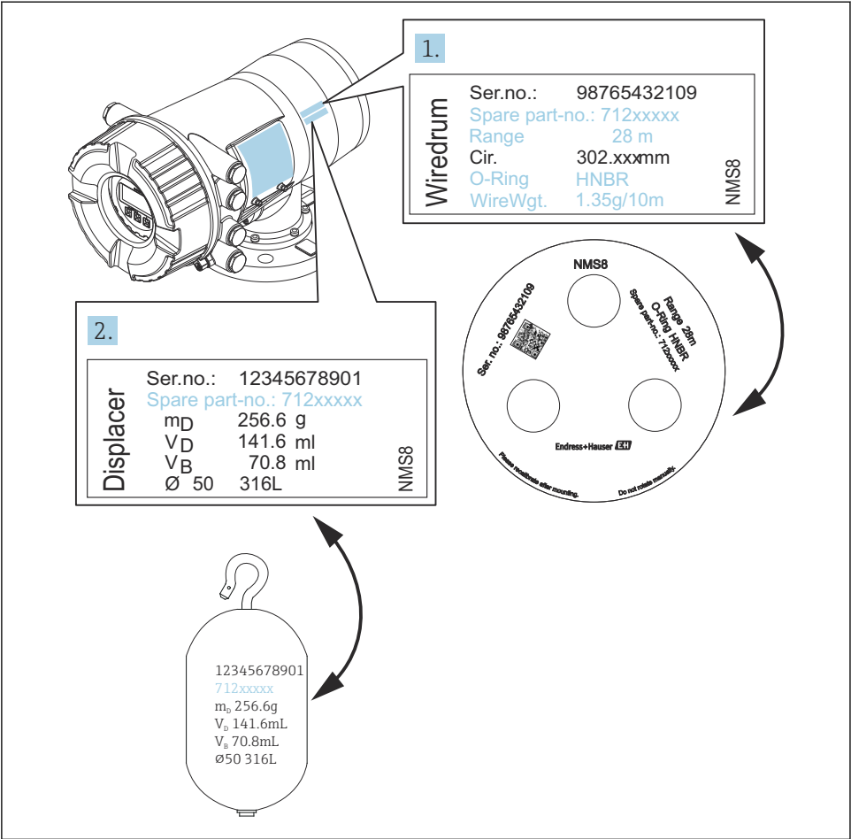
4 Verifikacija izpodrivnika in merilnega bobna
