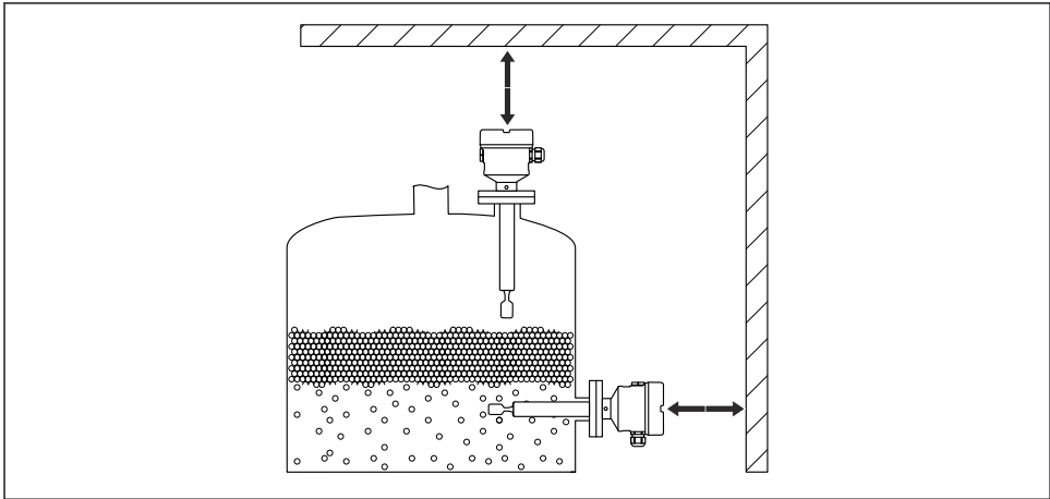
9 Abstand außerhalb des Tanks berücksichtigen
