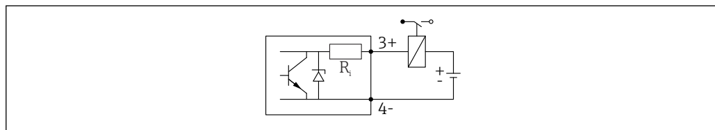
14 Conexión de un relé
