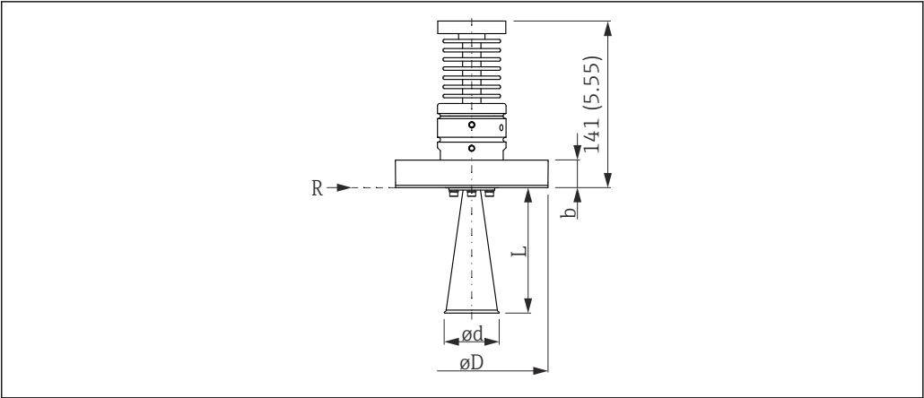
32 Dimensiones de la antena, versión T < 450\text{ }^{\circ}\text{C} (842 °F). Unidad de medida mm (in)
