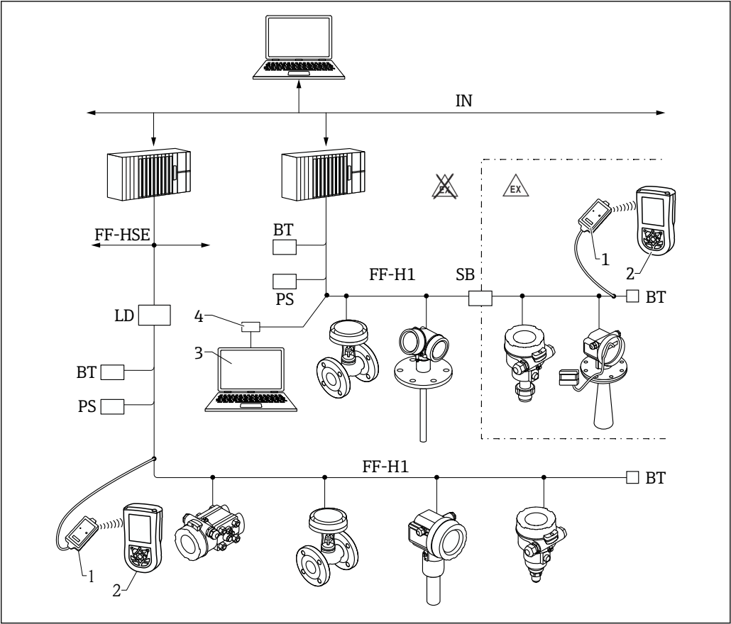
41 Arquitectura del sistema Fieldbus FOUNDATION con componentes asociados
