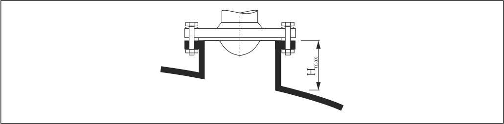
22 Altura de la tubuladura para una antena de bocina, soporte para montaje enrasado (FMR52)
