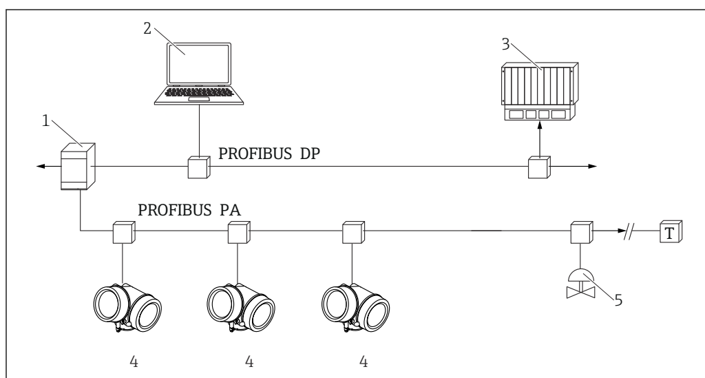
40 Opciones para la configuración a distancia mediante el protocolo de red PROFIBUS PA
