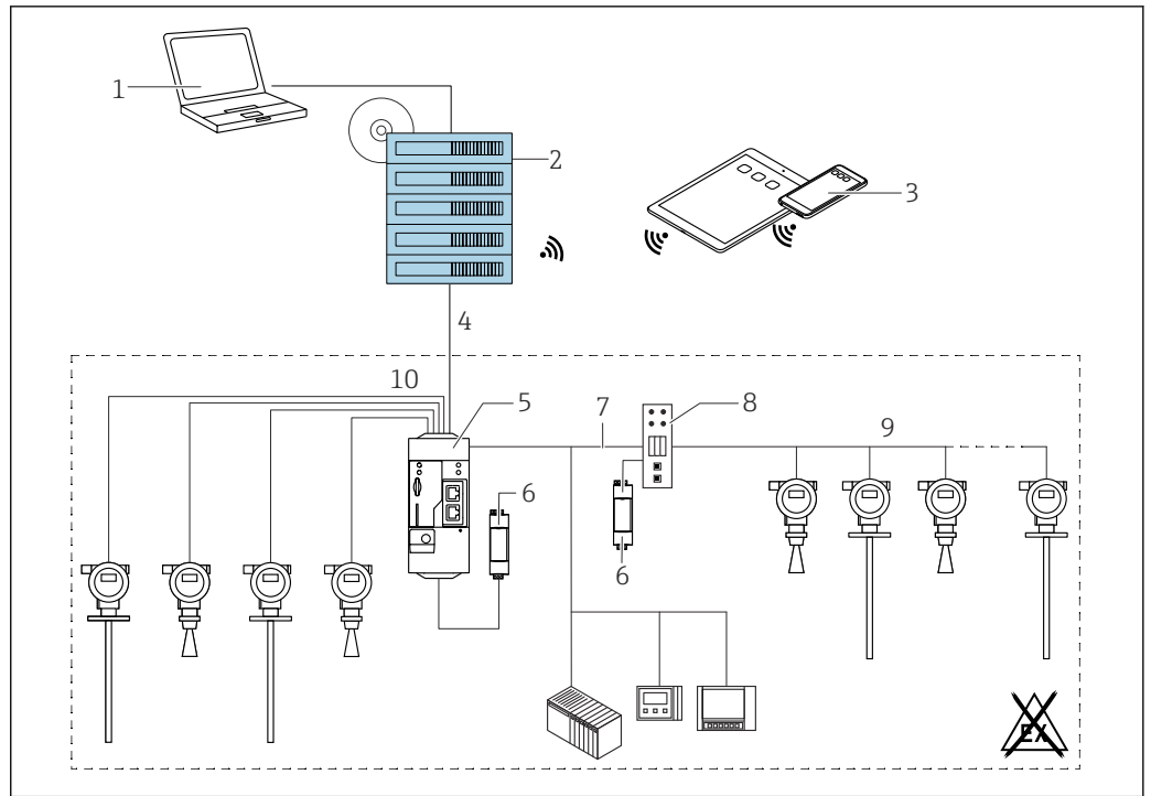
44 Ejemplo de plataforma para la gestión de inventario con SupplyCare Enterprise SCE30B
