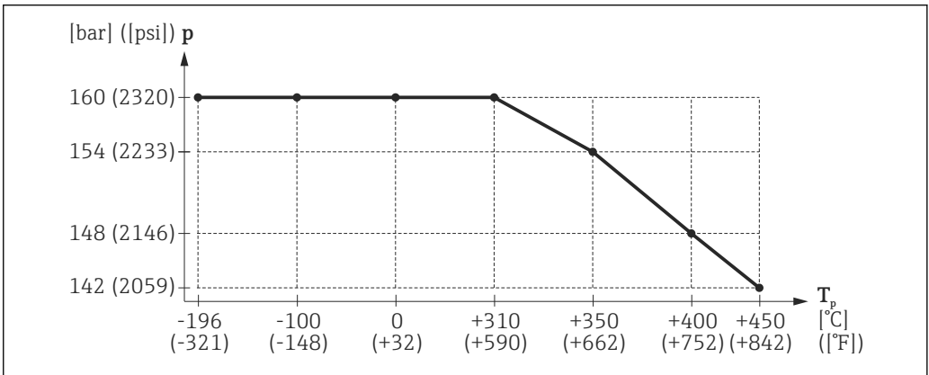
25 FMR51: rango admisible para temperatura de proceso y presión de proceso de la versión HT (característica 090 "Junta", versión D2)
