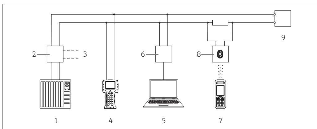
39 Opciones para la configuración a distancia mediante protocolo HART
