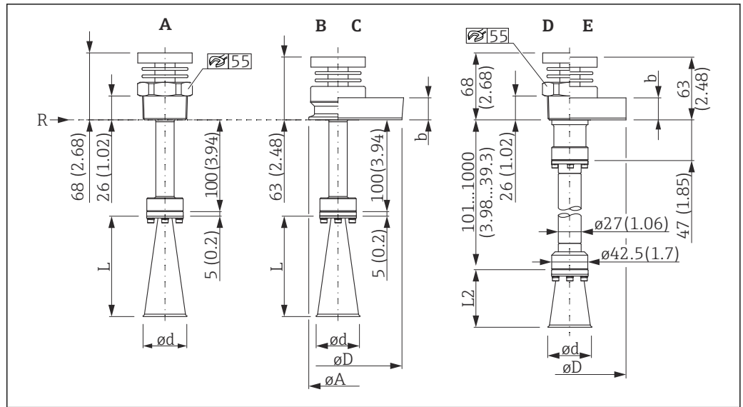
30 Dimensiones de la antena, versión con extensión. Unidad de medida mm (in)
