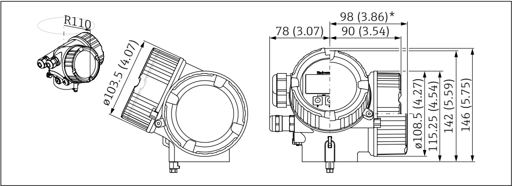
26 Caja GT18 (316L). Unidad de medida mm (in)
