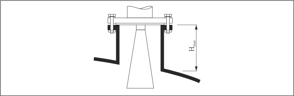
21 Altura de la tubuladura para una antena de bocina (FMR51)
