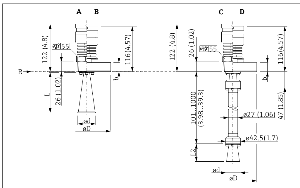
31 Dimensiones de la antena, versión T < 250\text{ °C} (482 °F). Unidad de medida mm (in)
