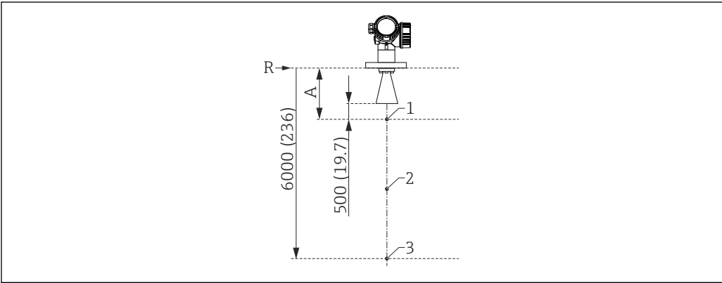
46 Puntos del protocolo de linealización de 3 puntos; unidad física: mm (in)
