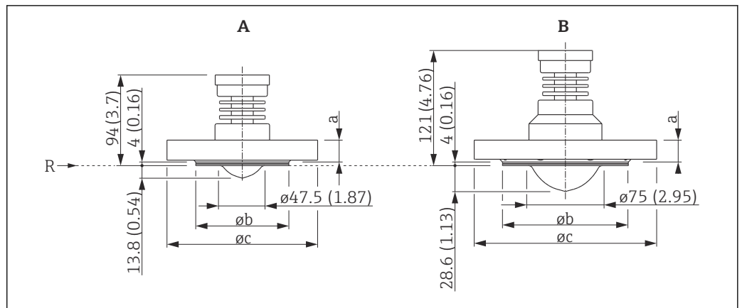
35 Dimensiones del equipo con brida. Unidad de medida mm (in)
