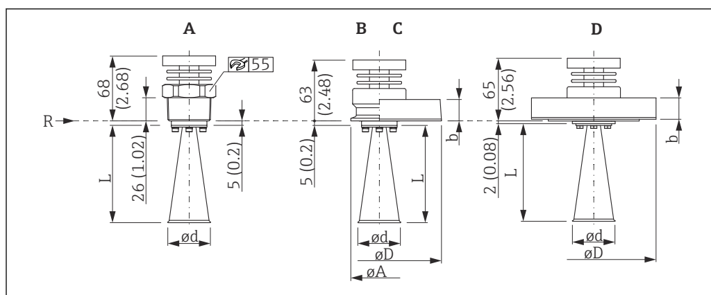
29 Dimensiones de la antena, versión sin extensión. Unidad de medida mm (in)
