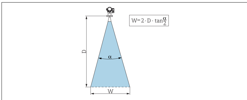
20 Relación entre el ángulo de abertura del haz \alpha , la distancia D y el ancho del haz W
