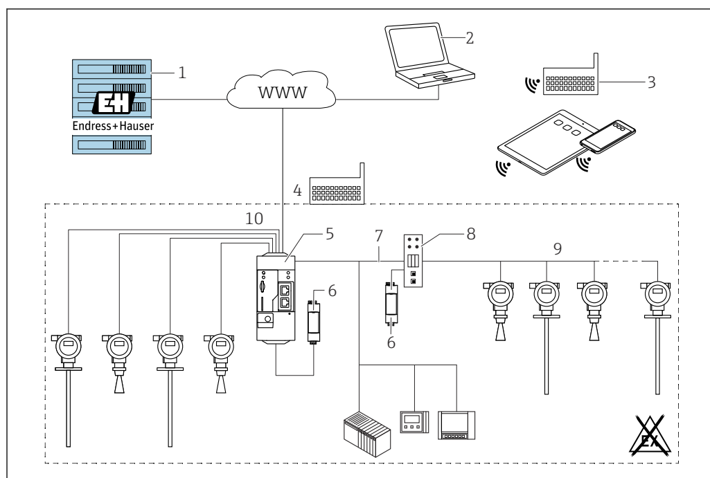
45 Ejemplo de plataforma para la gestión de inventario con SupplyCare Hosting SCH30
