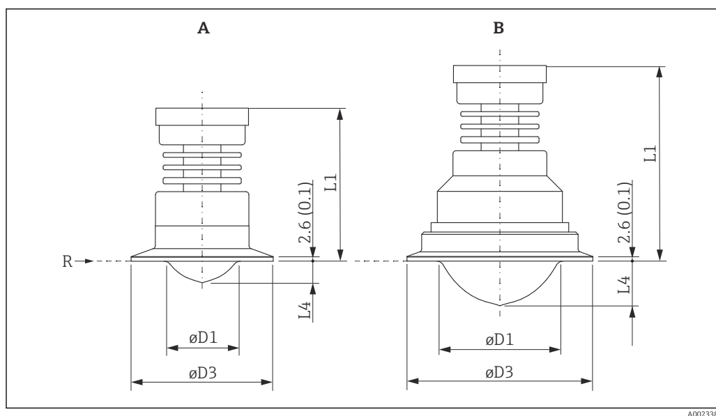
34 Dimensiones del equipo con conexión Tri-Clamp. Unidad de medida mm (in)
