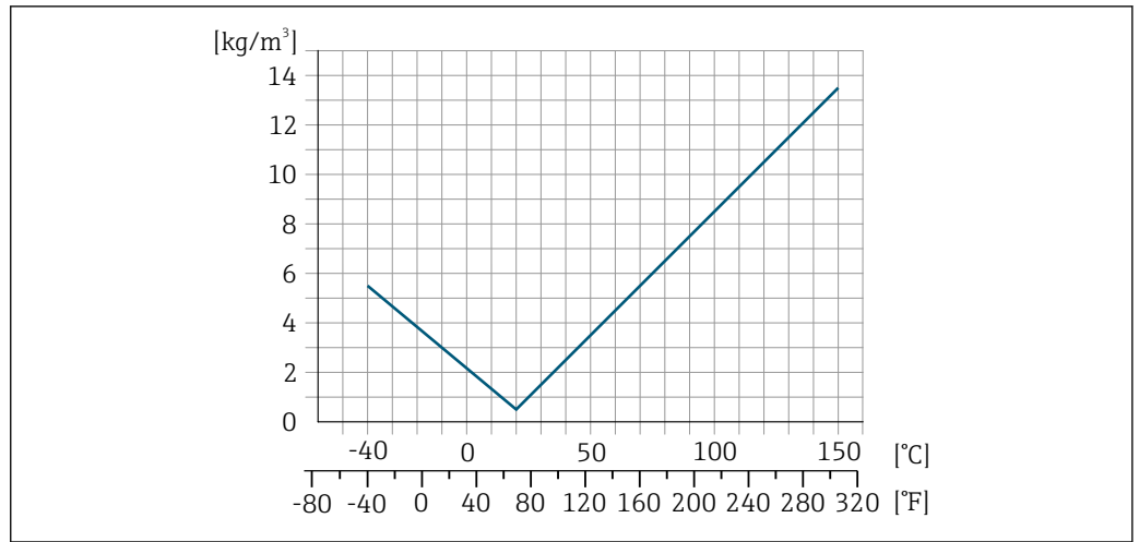
18 Felddichtejustierung, Beispiel bei +20 °C (+68 °F)
