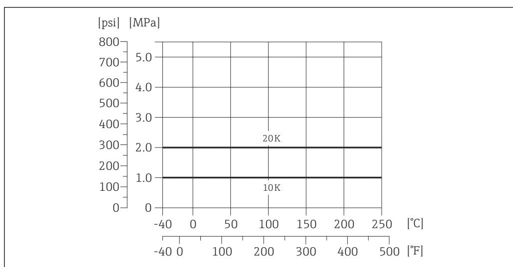
図 22 プロセス接続材質：鋳造アロイ CX2MW (アロイ C22/ 2.4602 と同等)
