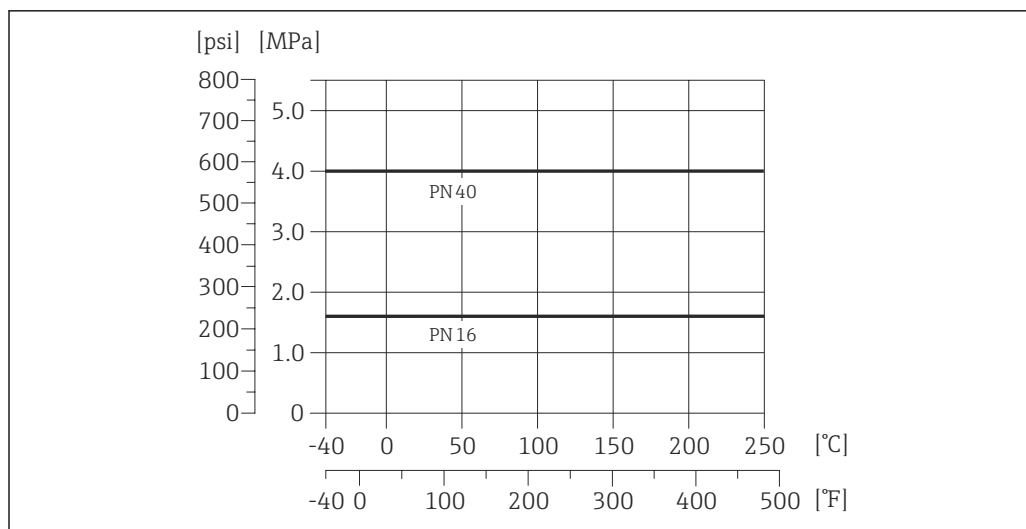
図 18 プロセス接続材質：鋳造アロイ CX2MW（アロイ C22/ 2.4602 と同等）
