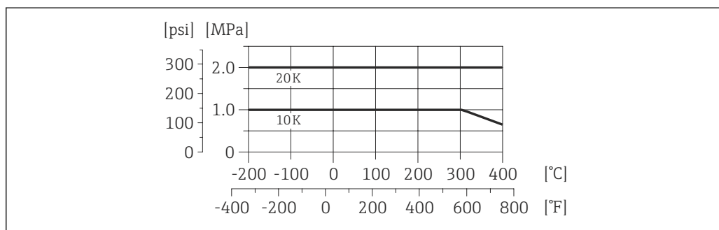
図 21 プロセス接続材質：ステンレス、複数の認証、1.4404 (SUS F316 または F316L 相当)
