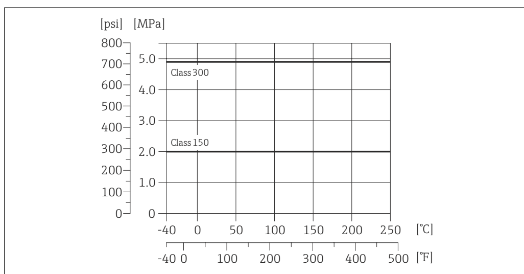
図 20 プロセス接続材質：鋳造アロイ CX2MW（アロイ C22/ 2.4602 と同等）
