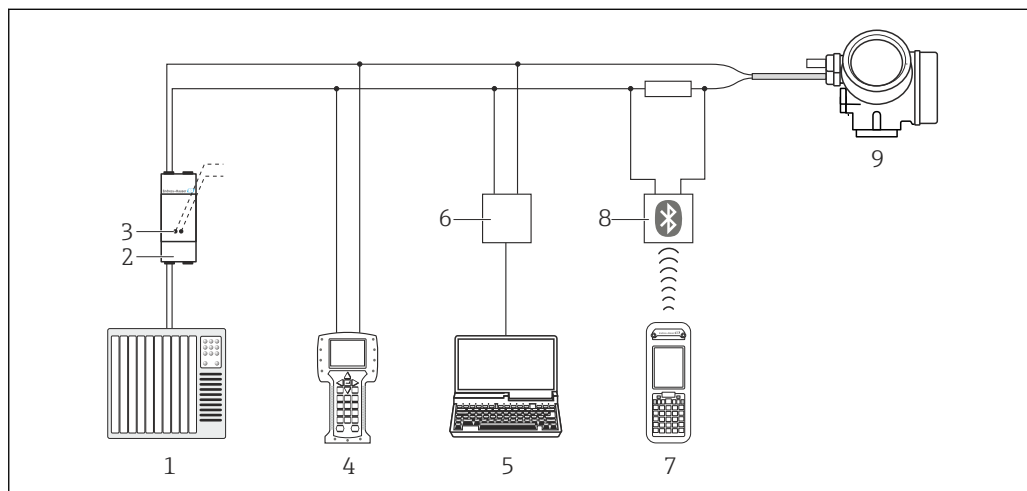
図 31 HART 経由のリモート操作用オプション
