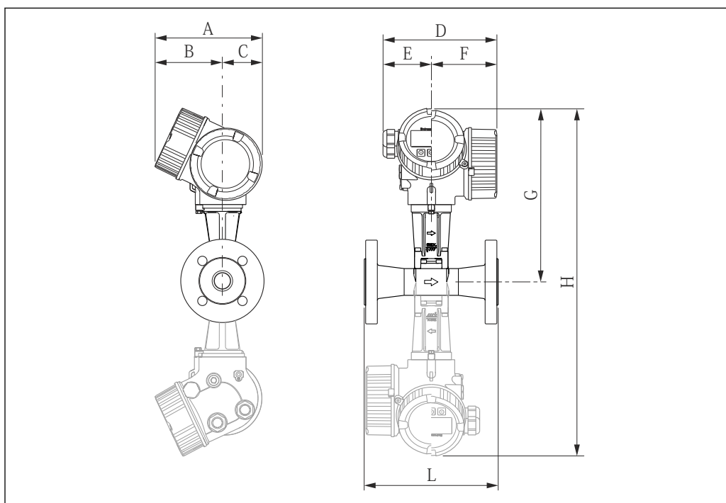
図 23 灰色破線：デュアルセンサタイプ
