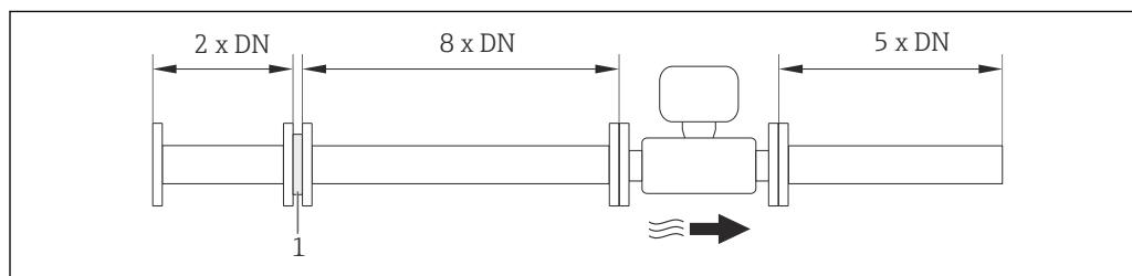
1 整流器
