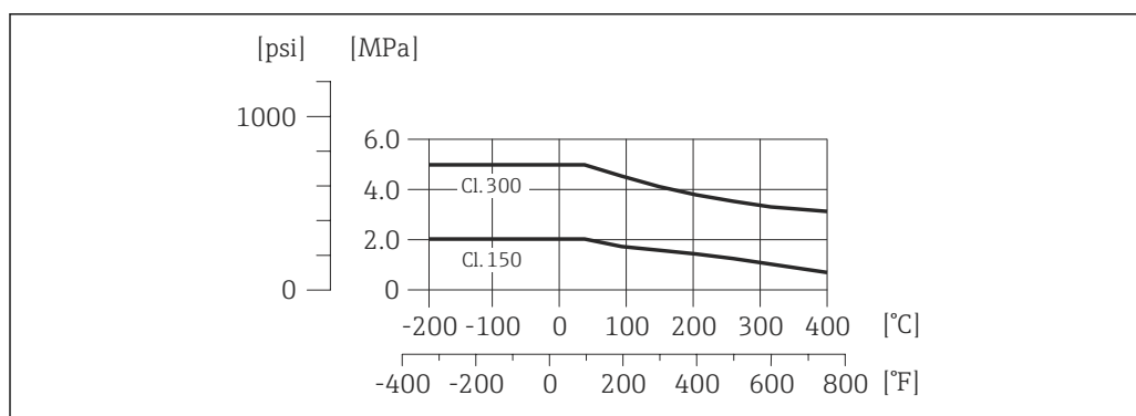
図 19 プロセス接続材質：ステンレス、複数の認証、1.4404 (SUS F316 または F316L 相当)
