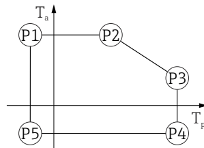
30 Custodia 316L; temperatura di processo -40 ... +80 °C (-40 ... +176 °F)
