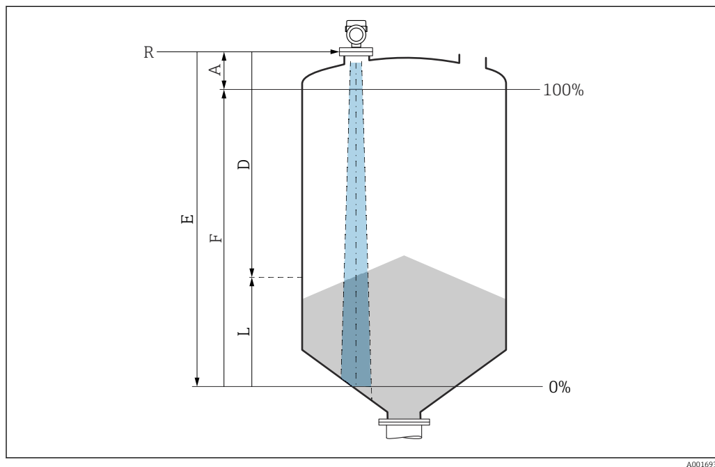
Fig. 13 Parametri di configurazione per la misura di livello nei solidi sfusi
