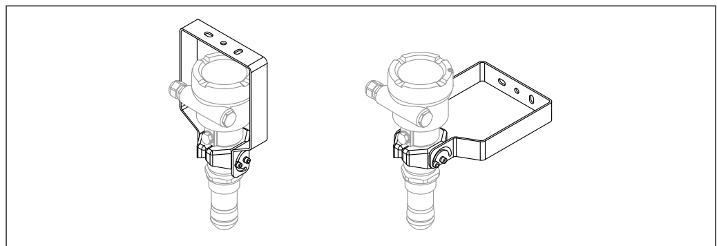
21 Staffa di montaggio regolabile FMR6xB; montaggio su soletta o a parete
