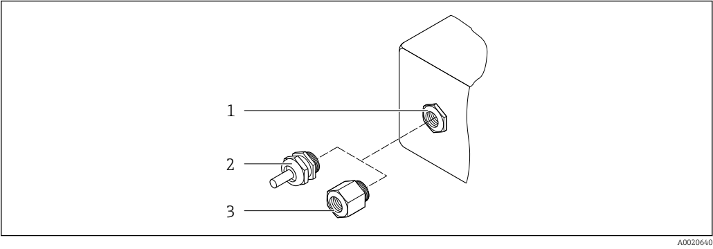
33 Entrées de câble/presse-étoupe possibles 1 Taraudage M20 × 1,5 2 Presse-étoupe M20 × 1,5 3 Adaptateur pour entrée de câble avec taraudage G ½" ou NPT ½"
