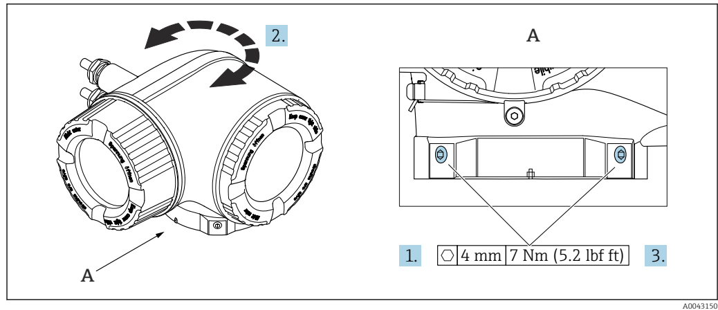
8 Boîtier Ex
