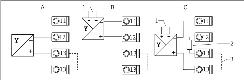
연결 예: 4~20 mA 전류 입력 또는 HART의 2선식 및 4선식 센서
