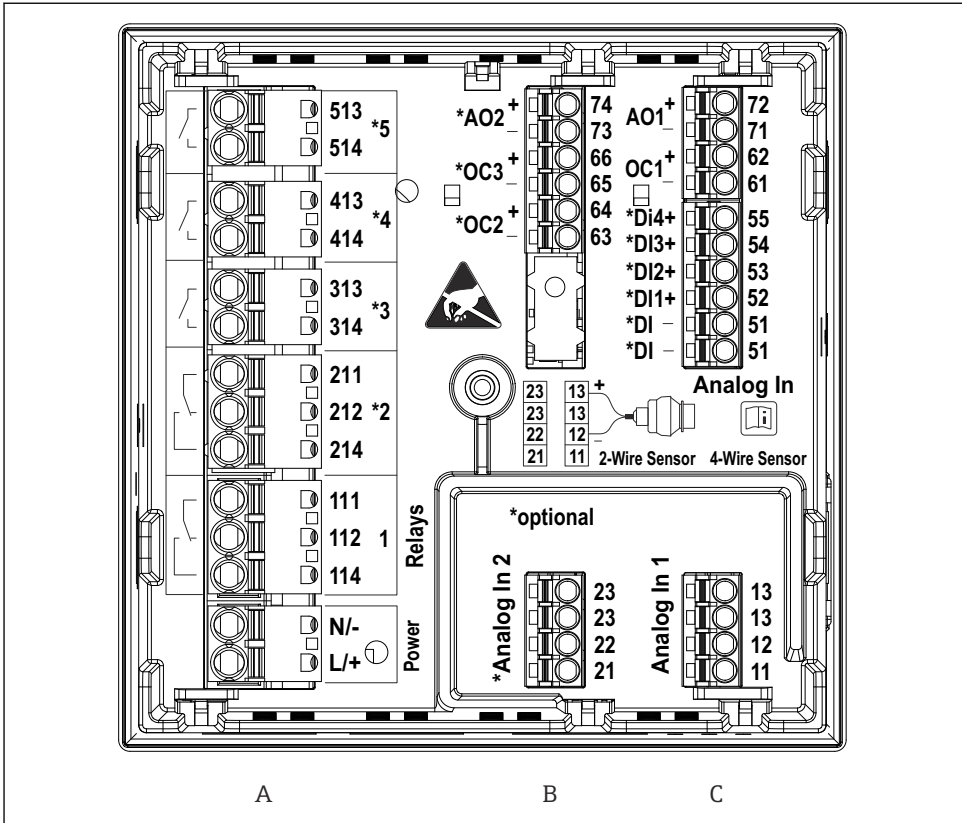
8 패널 설치 계기의 단자(계기 후면); 단자 디자인: 탈착식 푸시인 단자
