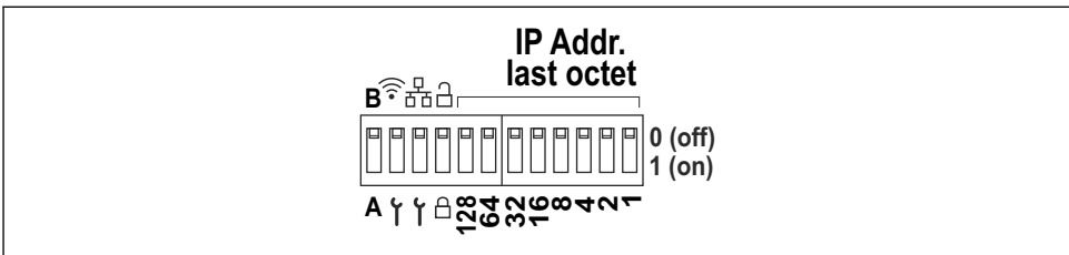
18 DIP 스위치(도면은 기본 설정 상태)
