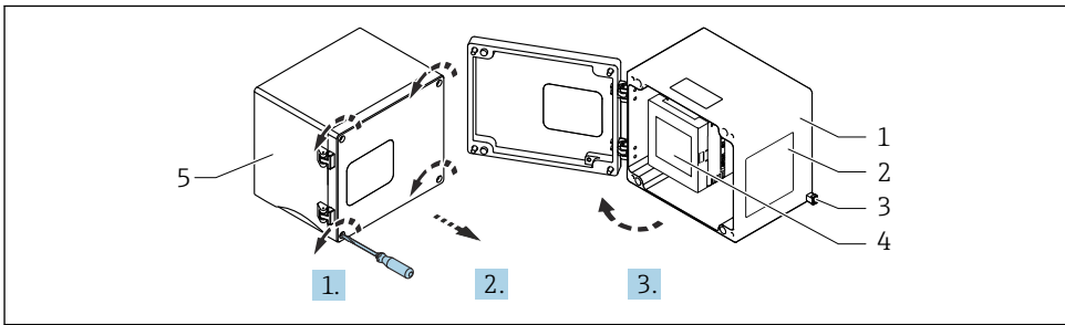
📖 6 알루미늄 필드 하우징의 단자부 액세스
