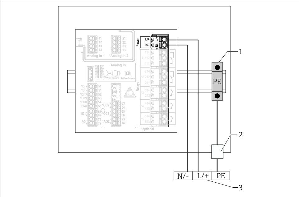
15 알루미늄 필드 하우징의 전원 공급 연결
