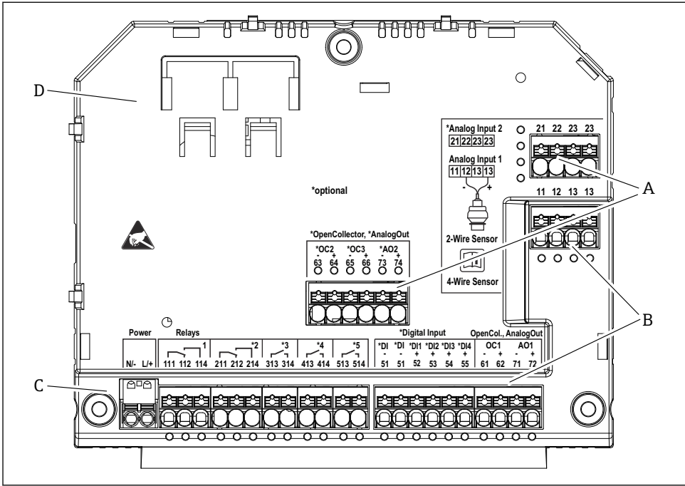
☐ 10 폴리카보네이트 필드 하우징 단자부의 단자; 단자 디자인: 푸시인 단자
