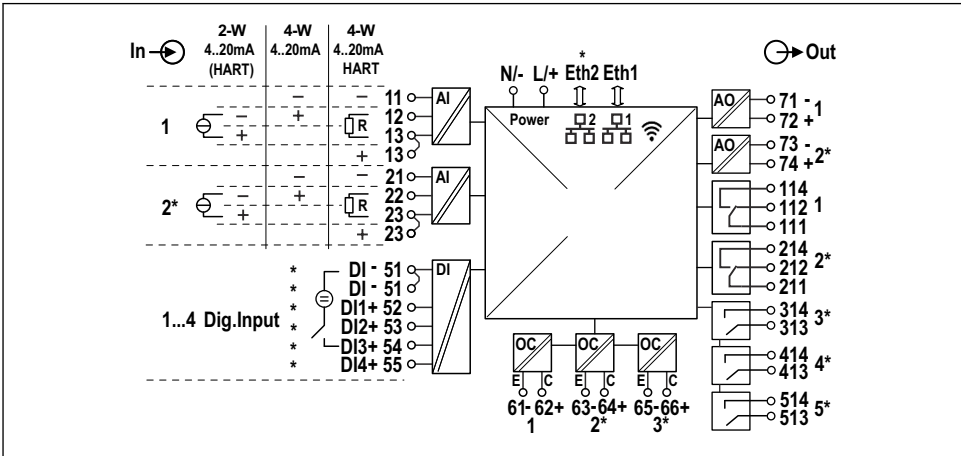
12 연결도(* 표시가 있는 단자는 옵션에 따라 다름)
