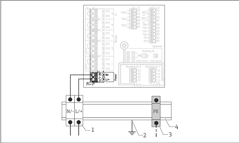
17 패널 설치 계기의 전원 공급 연결
