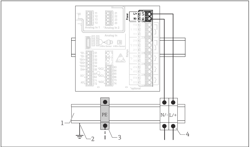
☐ 16 DIN 레일 계기의 전원 공급 연결
