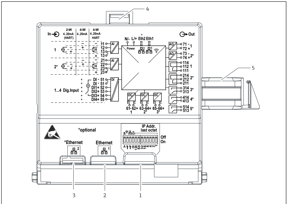
11 폴리카보네이트 필드 하우징의 디스플레이 후면에 있는 연결부
