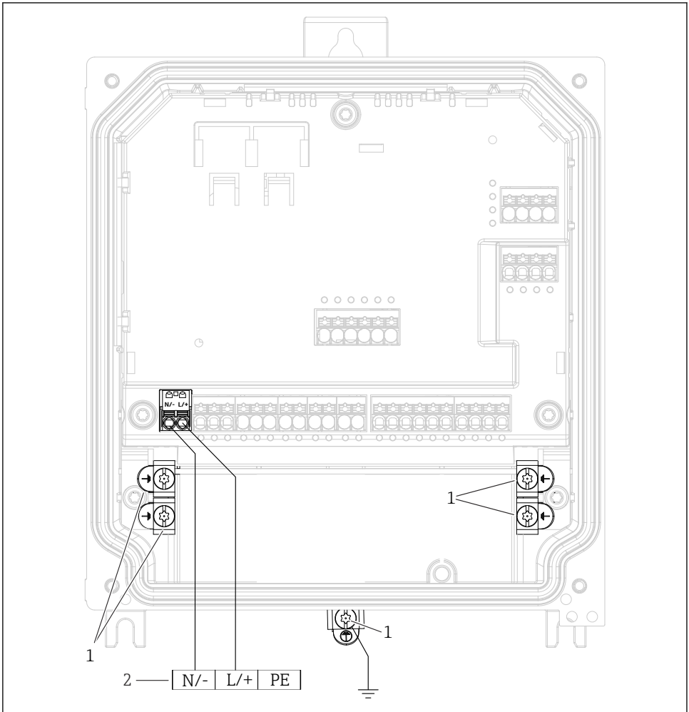
14 폴리카보네이트 필드 하우징의 전원 공급 연결
