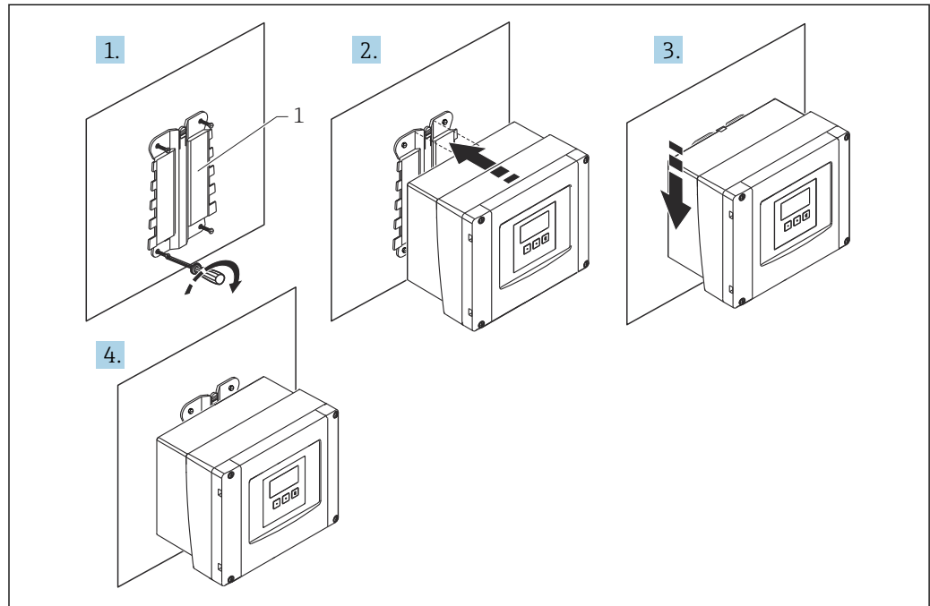
図 7 ポリカーボネート製フィールドハウジングの壁面取付け
