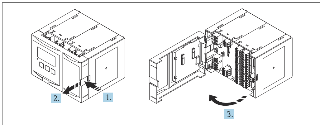
図 19 端子室へのアクセス：単体の DIN レールハウジングユニット
