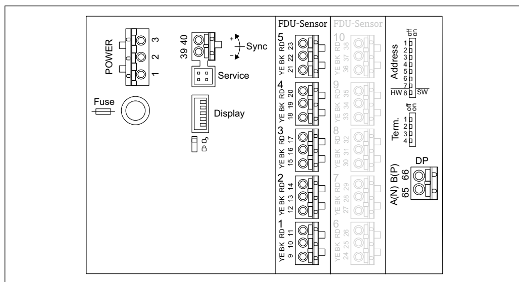
図 21 Prosonic S FMU95 の端子部
