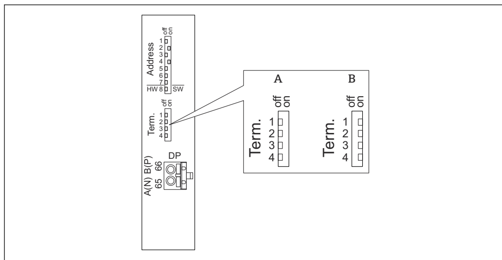
図 39 機器のバスターミネータ
