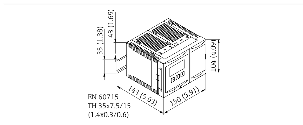
図 11 DIN レールハウジング付き Prosonic S の寸法。測定単位 mm (in)
