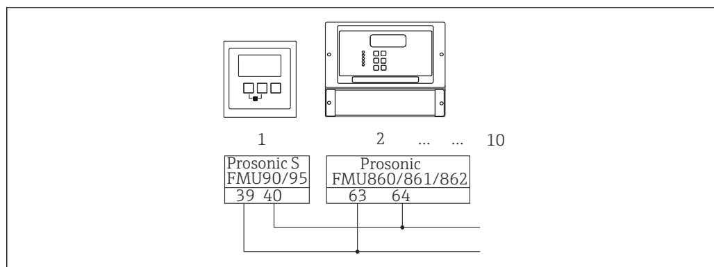
図 31 FMU90/FMU95 と FMU86x の同期
