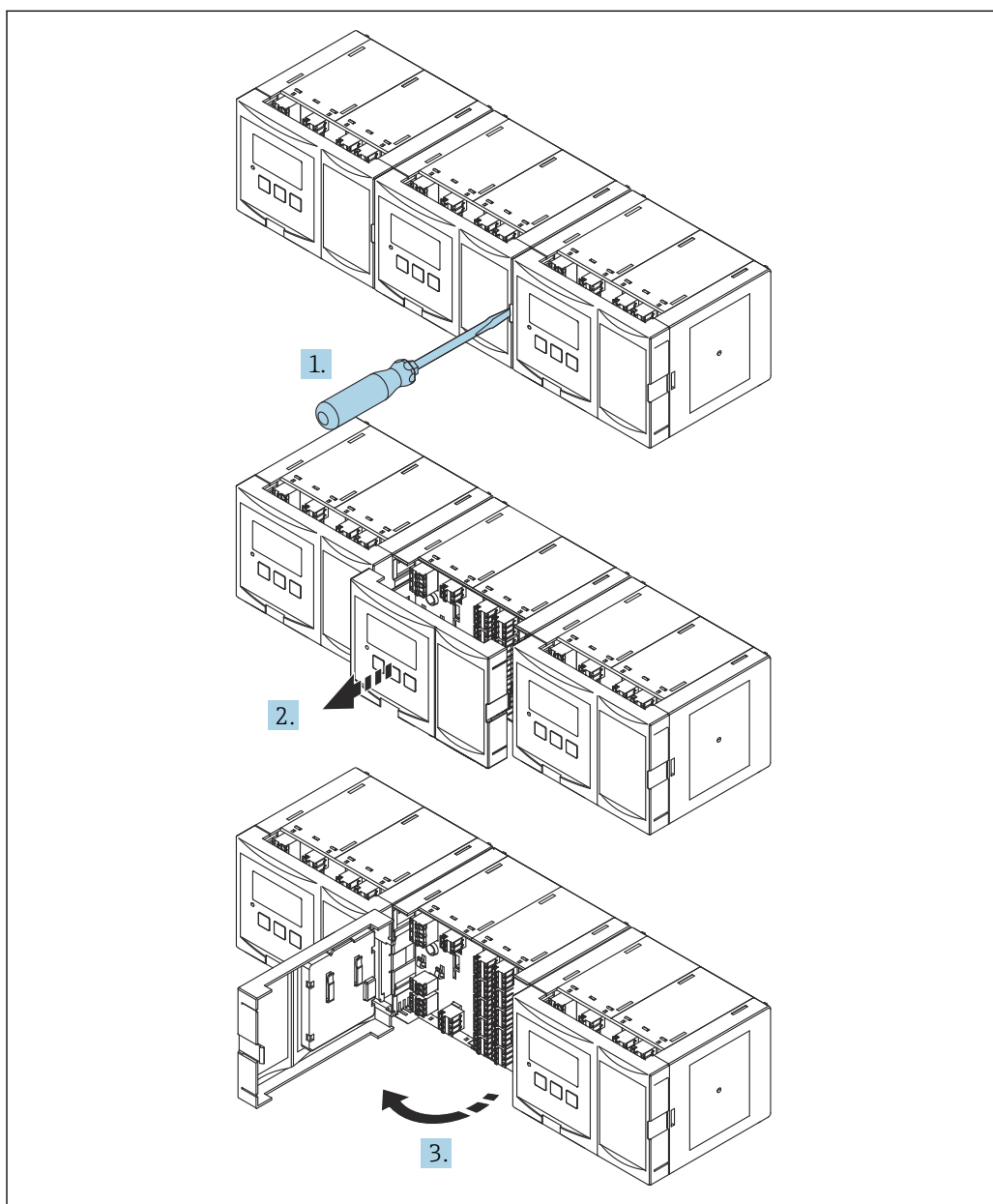
図 20 端子室へのアクセス：並んで取り付けられた複数の DIN レールハウジングユニット
