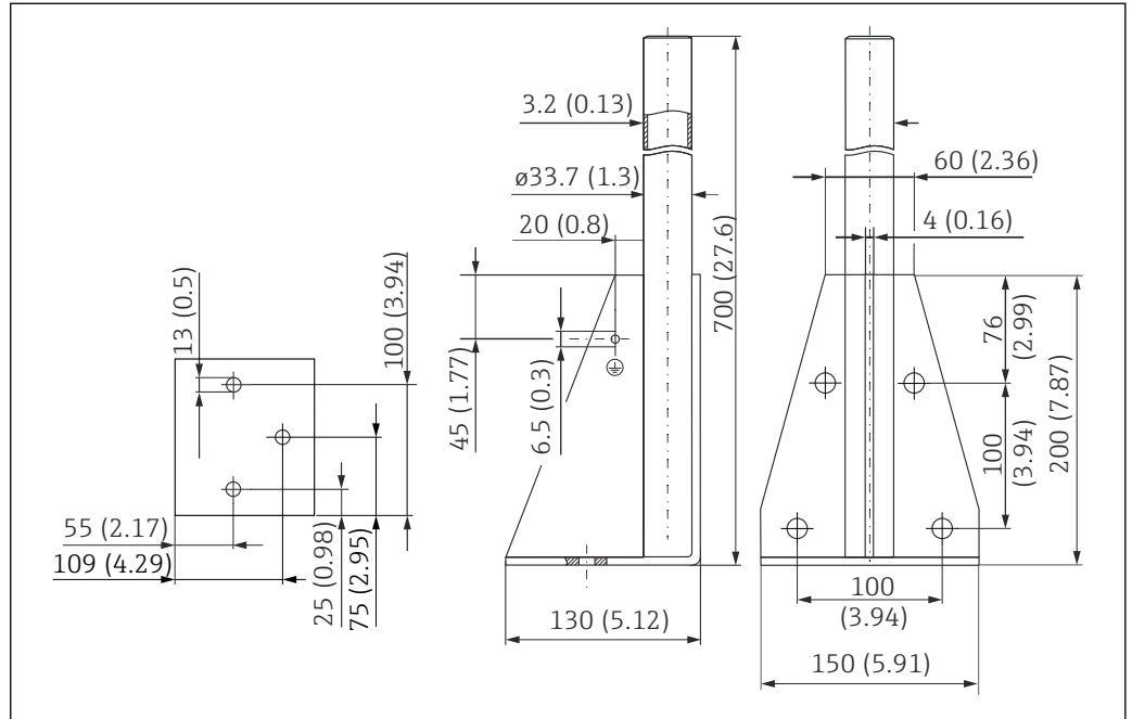
図 53 寸法。測定単位 mm (in)
