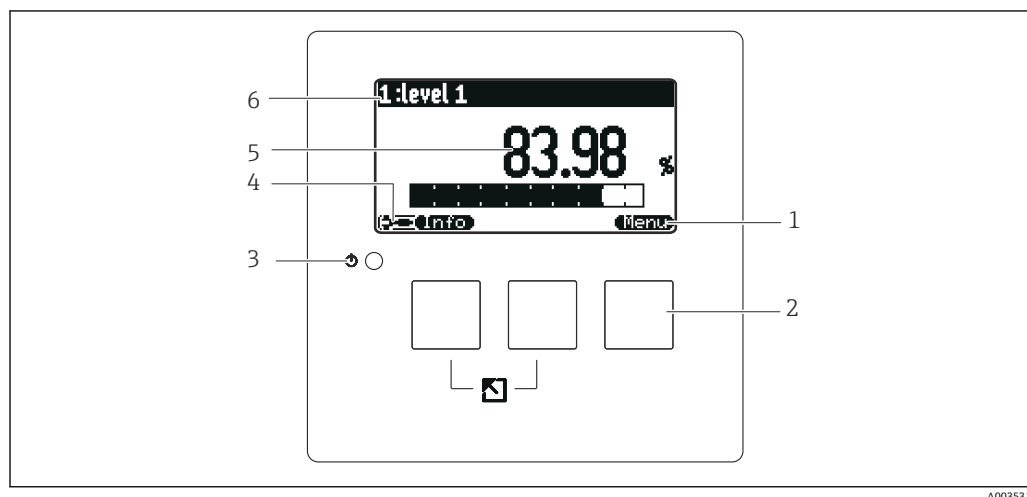
図 34 表示部および操作モジュール
