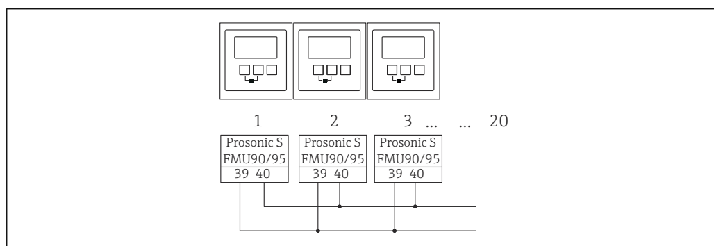
図 30 複数の FMU90/FMU95 変換器の同期
