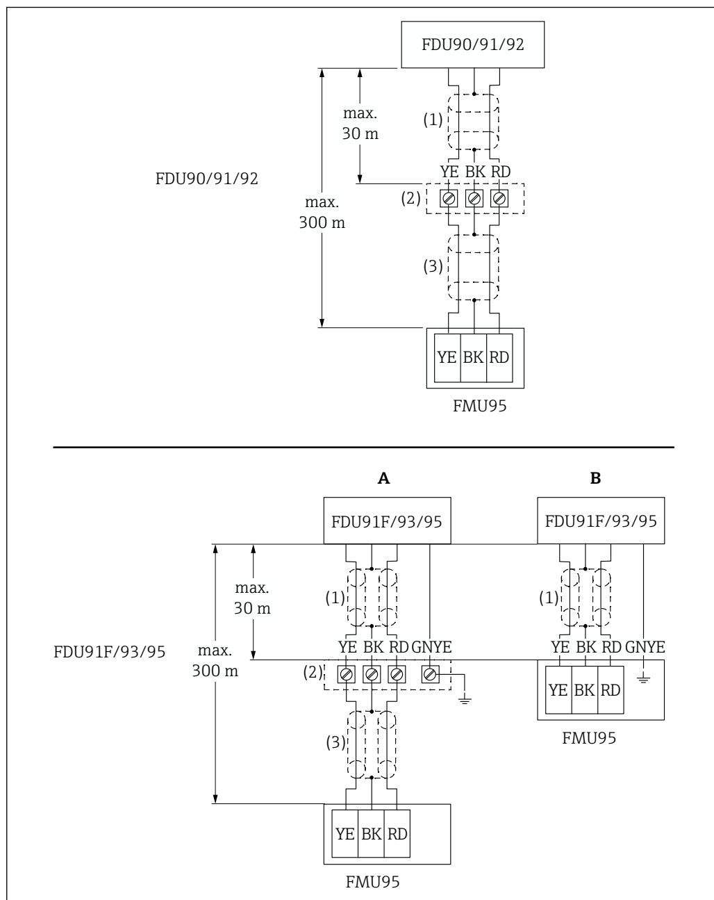
25 センサ FDU9x の接続図 ; YE : 黄色、BK : 黒色、RD : 赤色、BU : 青色、BN : 茶色、GNYE : 緑色/黄色
