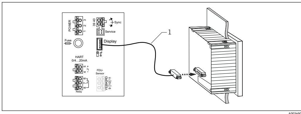
図 32 分離型ディスプレイと操作モジュールの接続
