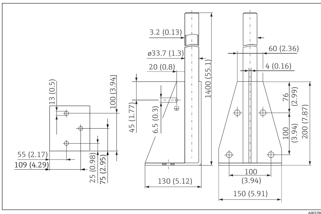
図 54 寸法。測定単位 mm (in)
