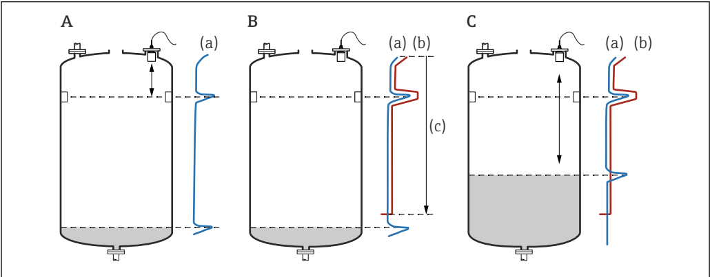
図 43 不要反射の抑制（マッピング）機能の動作原理
