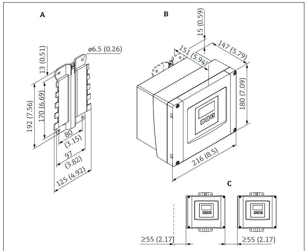
図 6 ポリカーボネート製フィールドハウジング付き Prosonic S の寸法。測定単位 mm (in)
