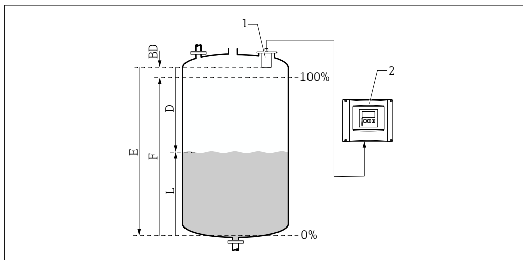
図 41 レベル測定のための空/満量校正
