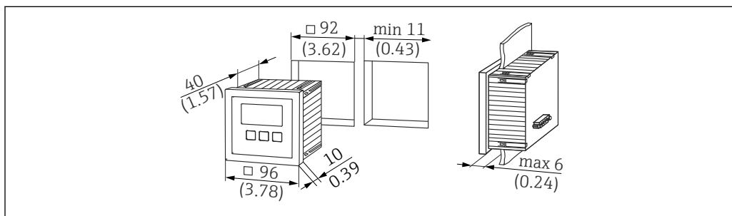
図 13 分離型ディスプレイと操作モジュール用の開口部。測定単位 mm (in)
