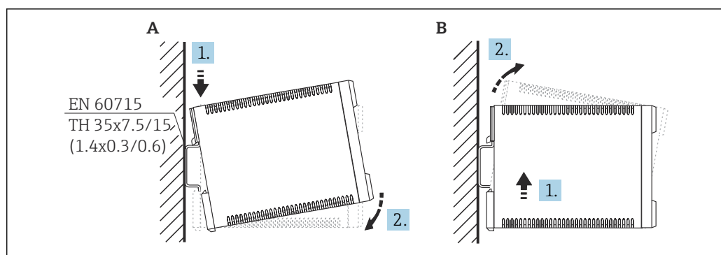
図 12 DIN レールハウジングの取付け/取外し。測定単位 mm (in)
