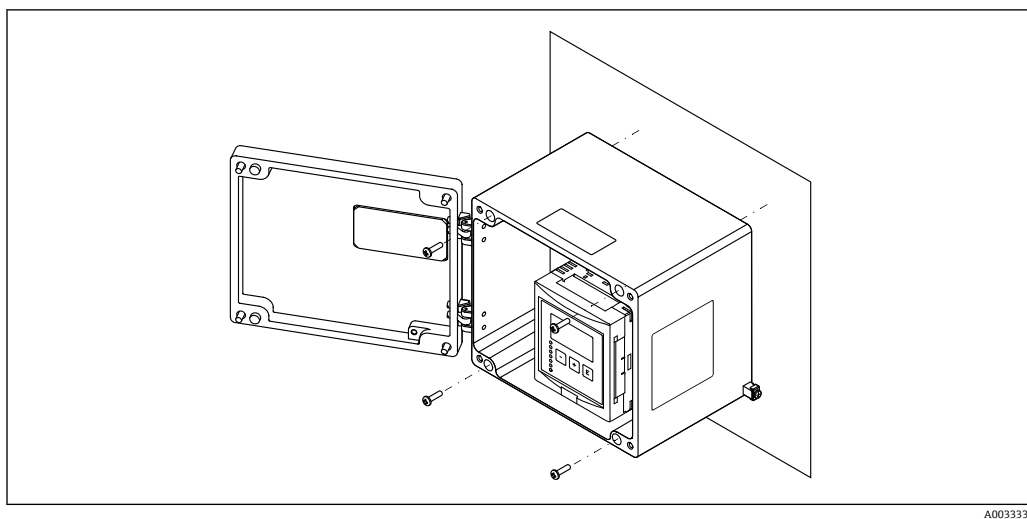
■ 10 アルミニウム製フィールドハウジングの壁面取付け
