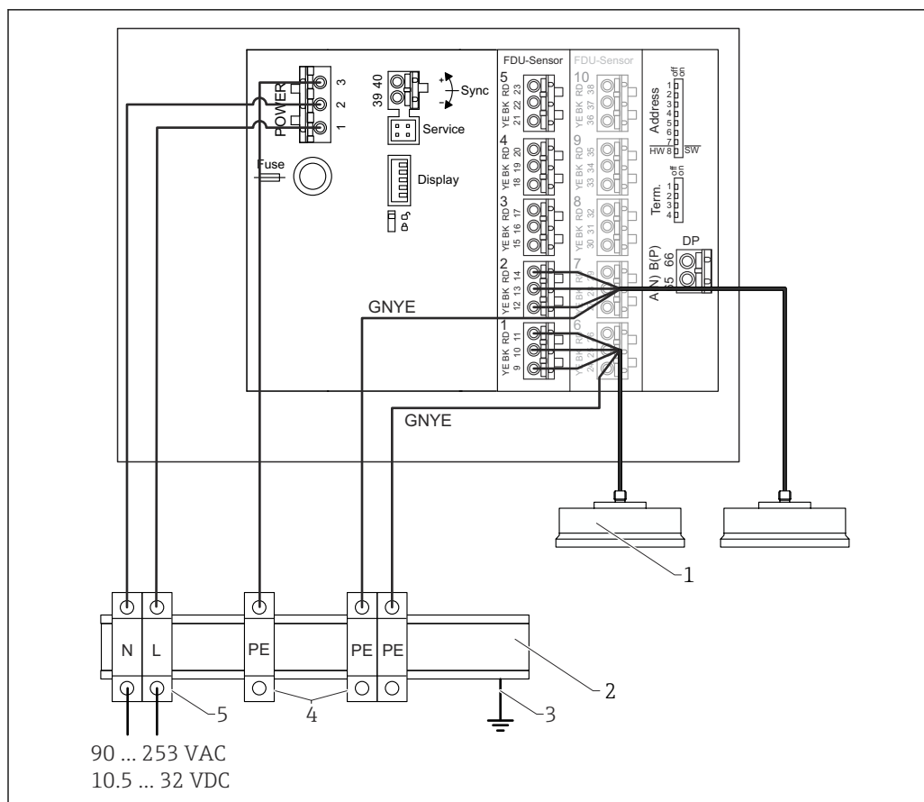
図 28 DIN レールハウジング内の金属製センサの電位平衡
