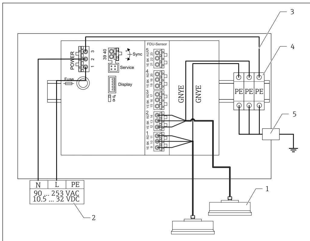
図 27 アルミニウム製フィールドハウジング内の金属製センサの電位平衡
