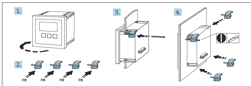
図 15 リモートディスプレイと操作モジュールの取付け
