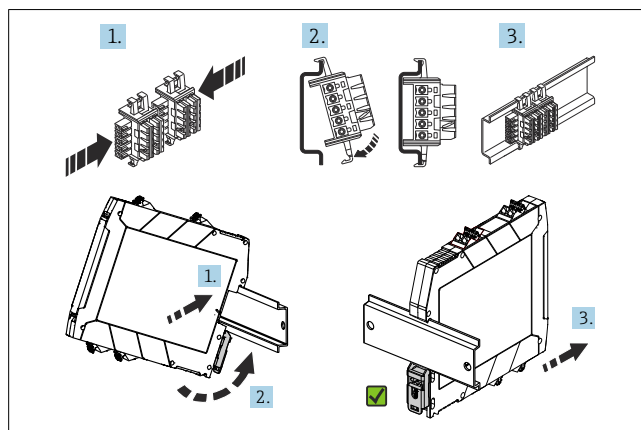
1 Namestitev konektorja za napajanje iz DIN-letve 12,5 mm (0,5 in) (zgoraj) in namestitev na DIN-letev (spodaj)
