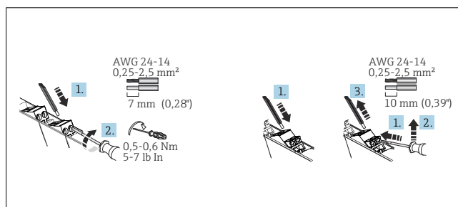
2 Električna priključitev z vijajnimi (levo) in potisnimi sponkami (desno)
