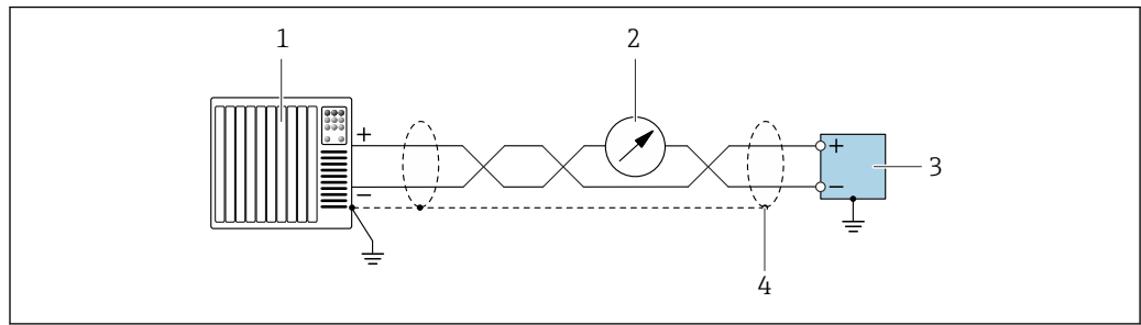
27 Exemplo de conexão para saída em corrente 4 para 20 mA com HART (ativa)
