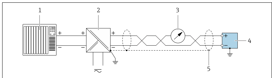
28 Exemplo de conexão para saída em corrente 4 para 20 mA com HART (passiva)
