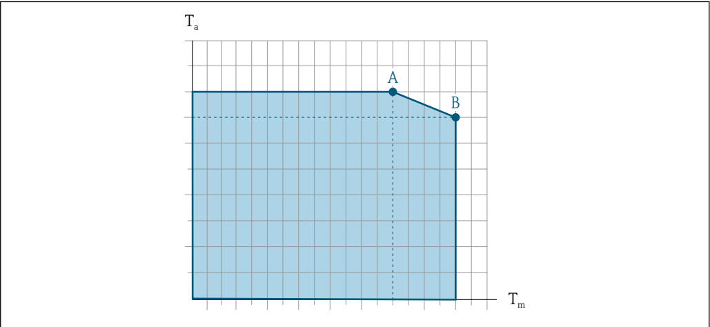
46 Representação exemplar, valores na tabela abaixo. T_a Temperatura ambiente T_m Temperatura do meio A Temperatura máxima permitida do meio T_m a T_a\text{ máx.} = 60\text{ °C (140 °F)} ; temperaturas do meio mais altas T_m requerem uma redução na temperatura ambiente T_a B Temperatura ambiente T_a máxima permitida para a temperatura média T_m máxima especificada do sensor
