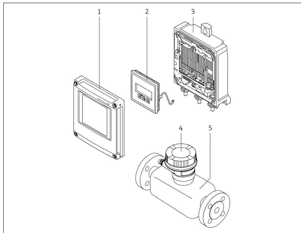
1 Componentes importantes de um medidor
