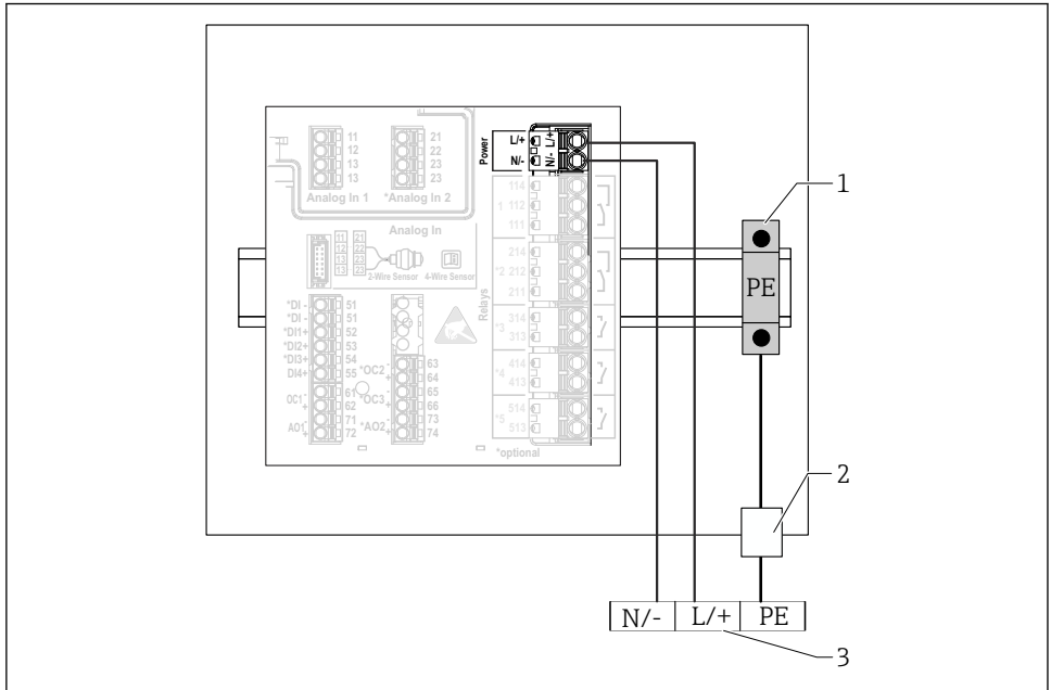
16 A tápellátás csatlakoztatása az alumínium terepi burkolatban
