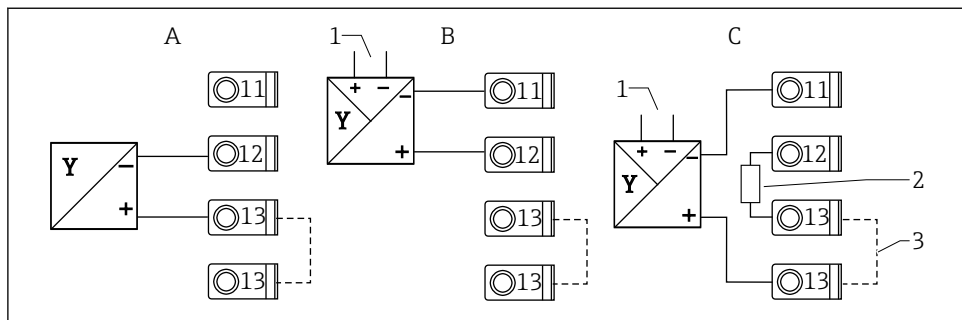
14 Csatlakozási példák: 2- és 4-vezetékes érzékelő 4–20 mA árambemenetre vagy HART-ra
