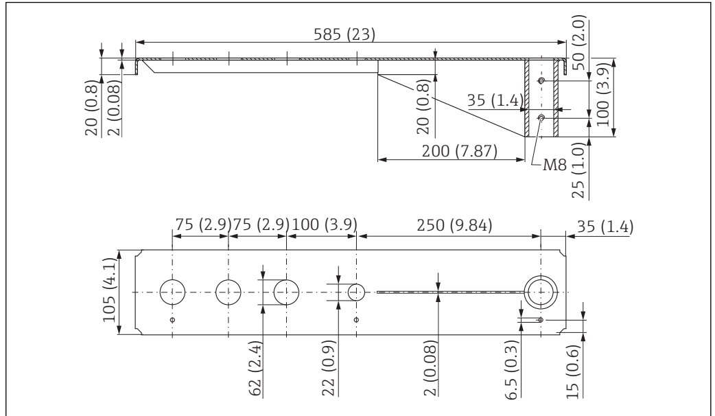
51 Abmessungen Ausleger (kurz) schwenkbar für Sensor Prozessanschluss Vorderseite G 2", Maßeinheit: mm (in)
