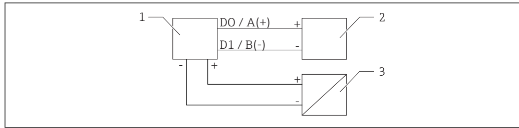
6 Blockschaltbild Modbus RS485 Anschluss
