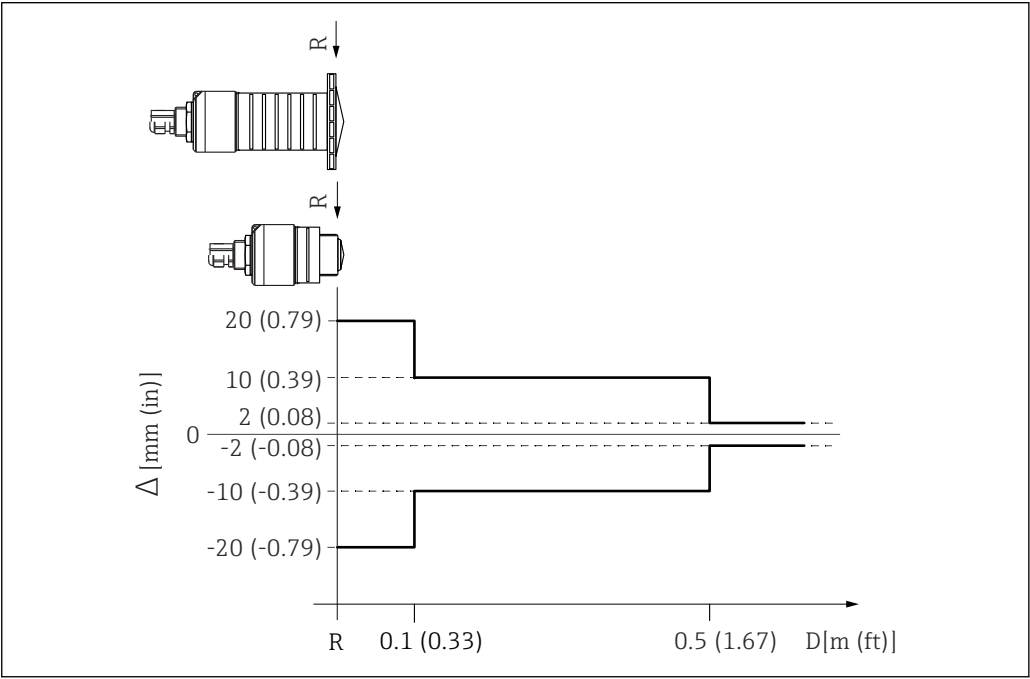
9 Maximale Messabweichung im Nahbereich; Werte für die Standard-Ausführung
