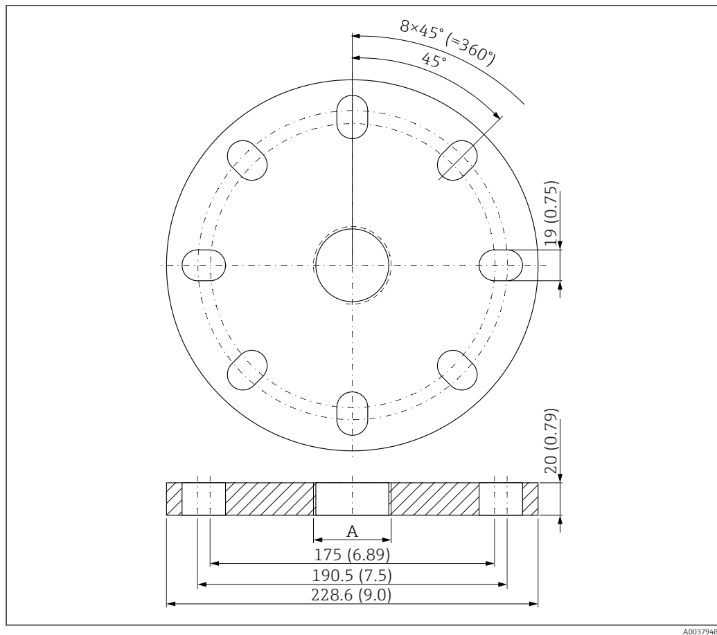
43 Abmessungen UNI Flansch 4"/DN100/100, Maßeinheit: mm (in)
