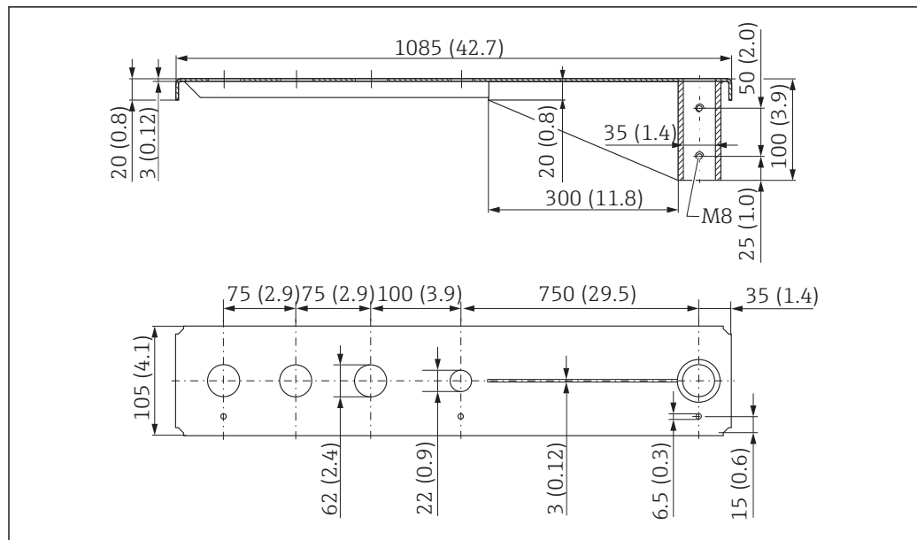
52 Abmessungen Ausleger (lang) schwenkbar für Sensor Prozessanschluss Vorderseite G 1-½", Maßeinheit: mm (in)
