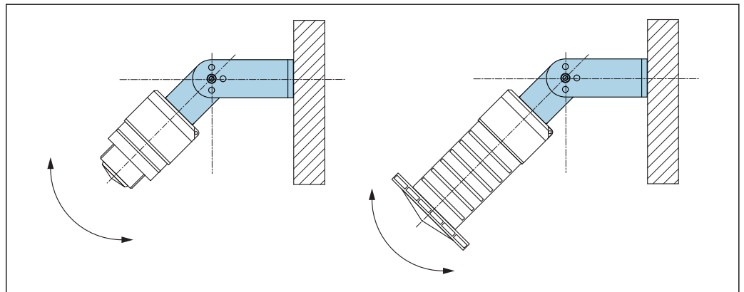
18 Einbau mit Montagebügel ausrichtbar
