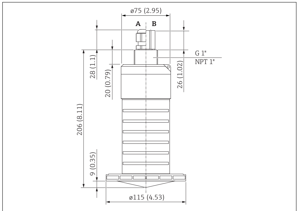
26 Abmessungen 80 mm (3 in) Antenne; Maßeinheit: mm (in)
