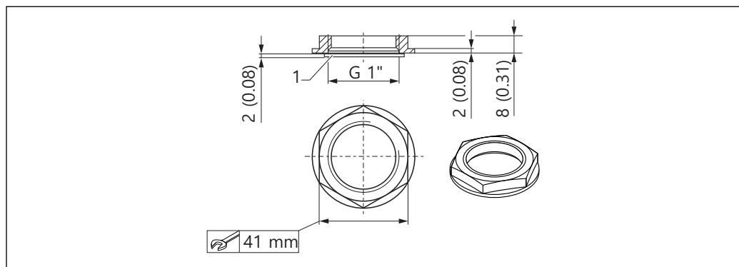
31 Abmessungen Gegenmutter Prozessanschluss Rückseite, Maßeinheit: mm (in)
