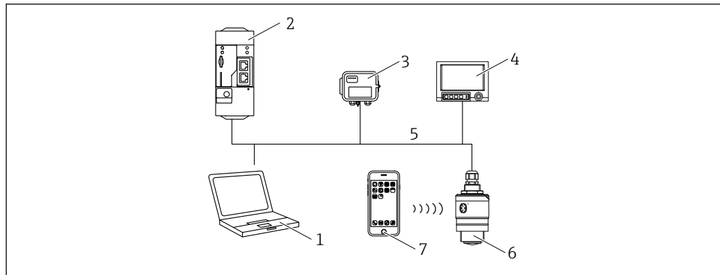
34 Möglichkeiten der Fernbedienung via Modbus-Protokoll
