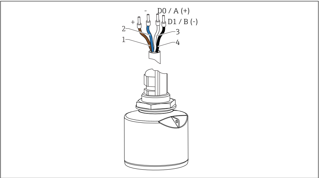
2 Kabelbelegung FMR20, Modbus
