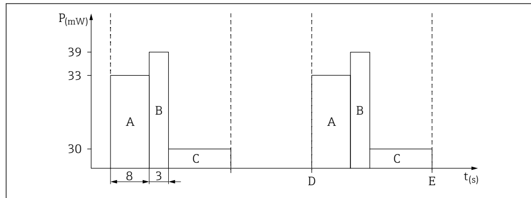
3 Leistungsaufnahme Einzelmessmodus ein-/ausgeschaltet via RTU
