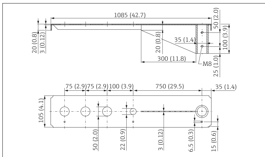
50 Abmessungen Ausleger (lang) schwenkbar für Sensor Prozessanschluss Vorderseite G 1-½", Maßeinheit: mm (in)
