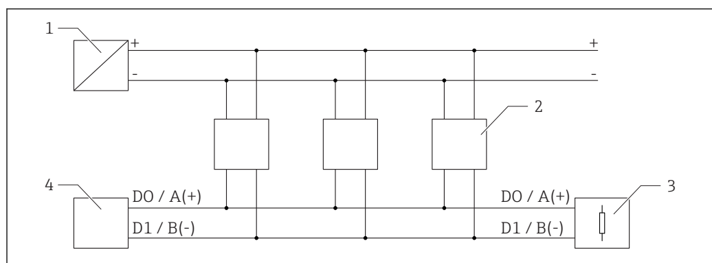
7 Blockschaltbild Modbus RS485 Anschluss, mehrere Teilnehmer
