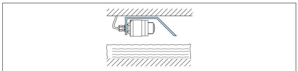
20 Montage horizontal mit Reflexionsblech
