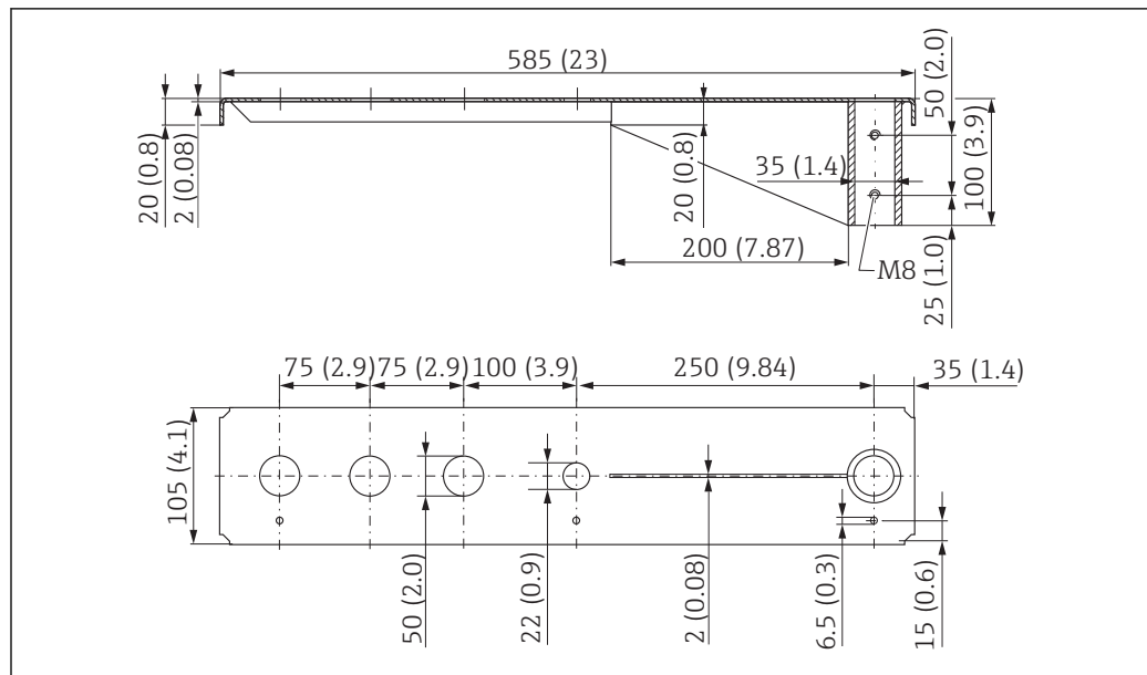
49 Abmessungen Ausleger (kurz) schwenkbar für Sensor Prozessanschluss Vorderseite G 1-½", Maßeinheit: mm (in)
