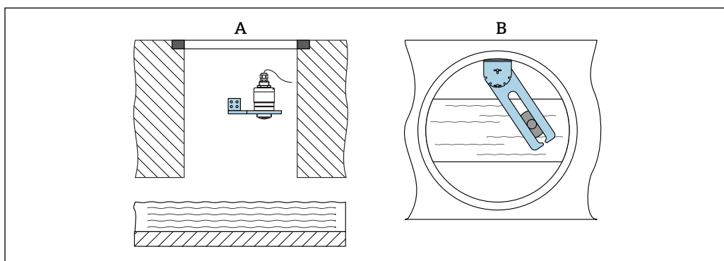
21 Montage im Schacht, schwenk- und verschiebbar
