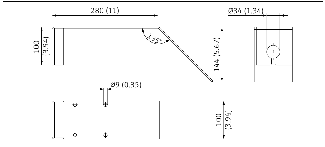
58 Abmessungen Reflexionsblech, Maßeinheit: mm (in)
