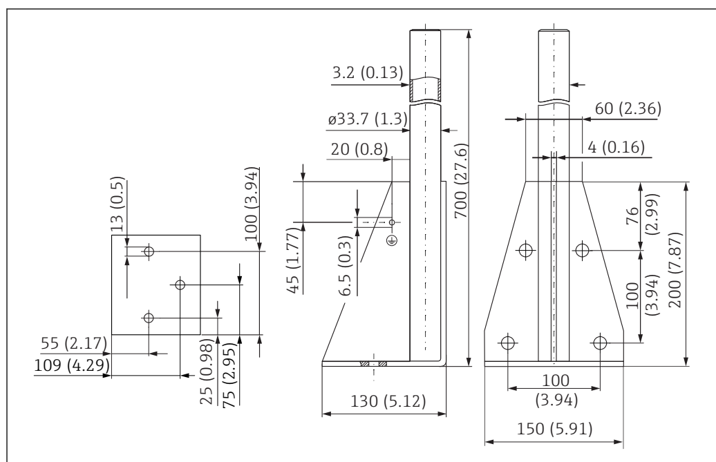
53 Abmessungen Montagegeständer (kurz), Maßeinheit: mm (in)
