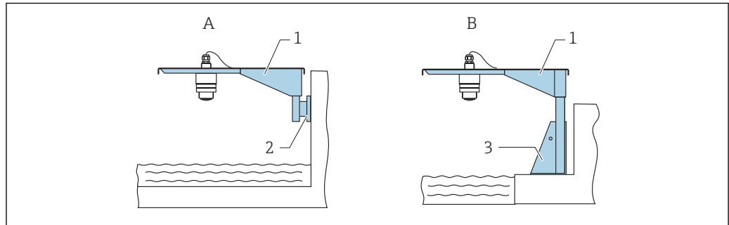
45 Montageart Sensor Prozessanschluss Rückseite
