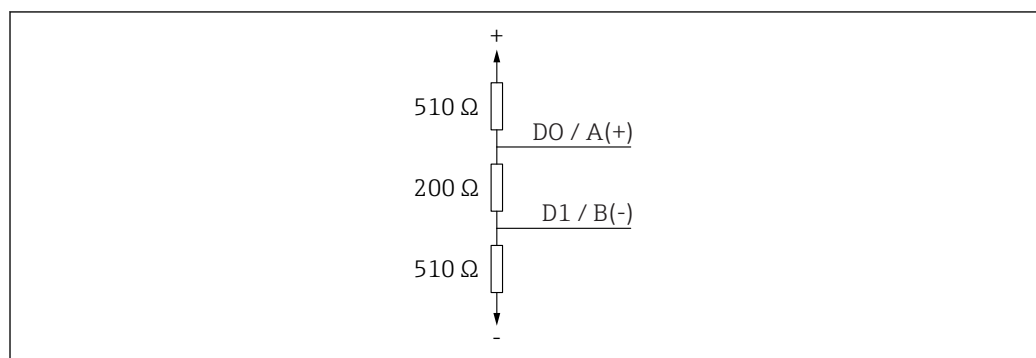
8 Darstellung Busabschlusswiderstand gemäss RS485-IS Spezifikation
