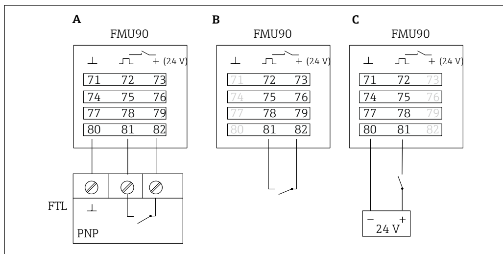
35 Conexão de seletoras externas
