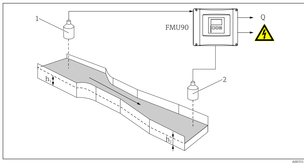
Fig. 49 Detecção de retorno com dois sensores ultrassônicos
