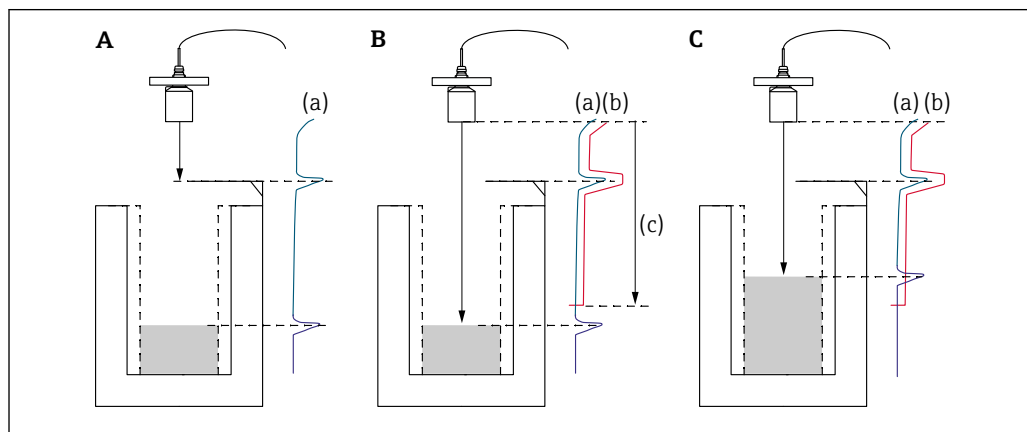
48 Princípio de operação da função de supressão de ecos de interferência (mapeamento)
