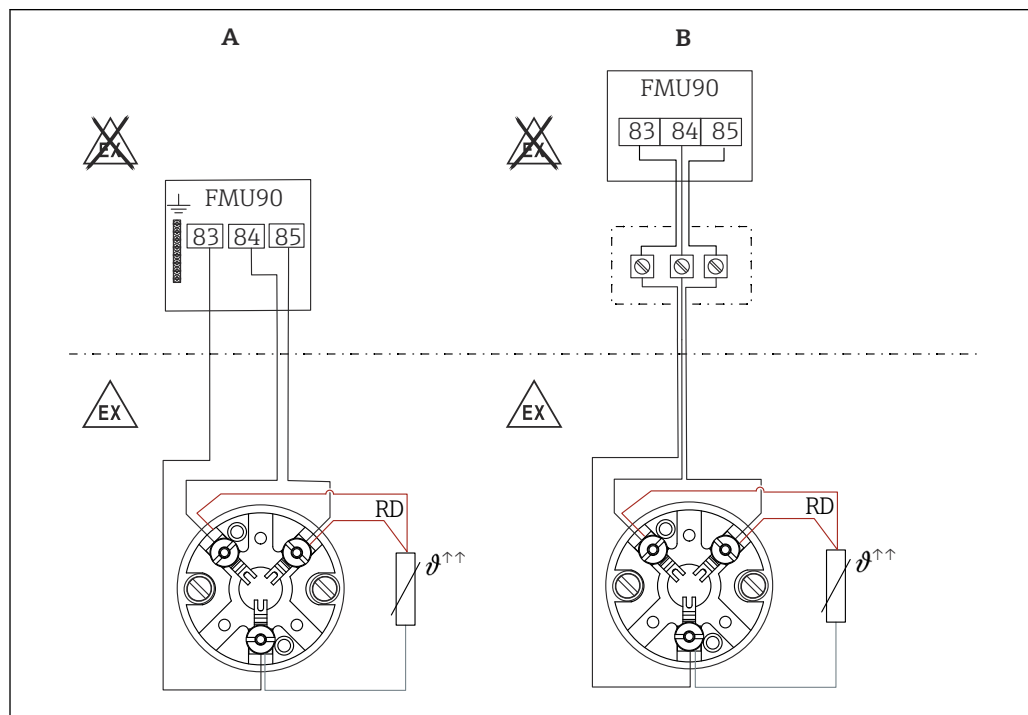
38 Conexão do Omnigrad S TR61 em áreas classificadas
