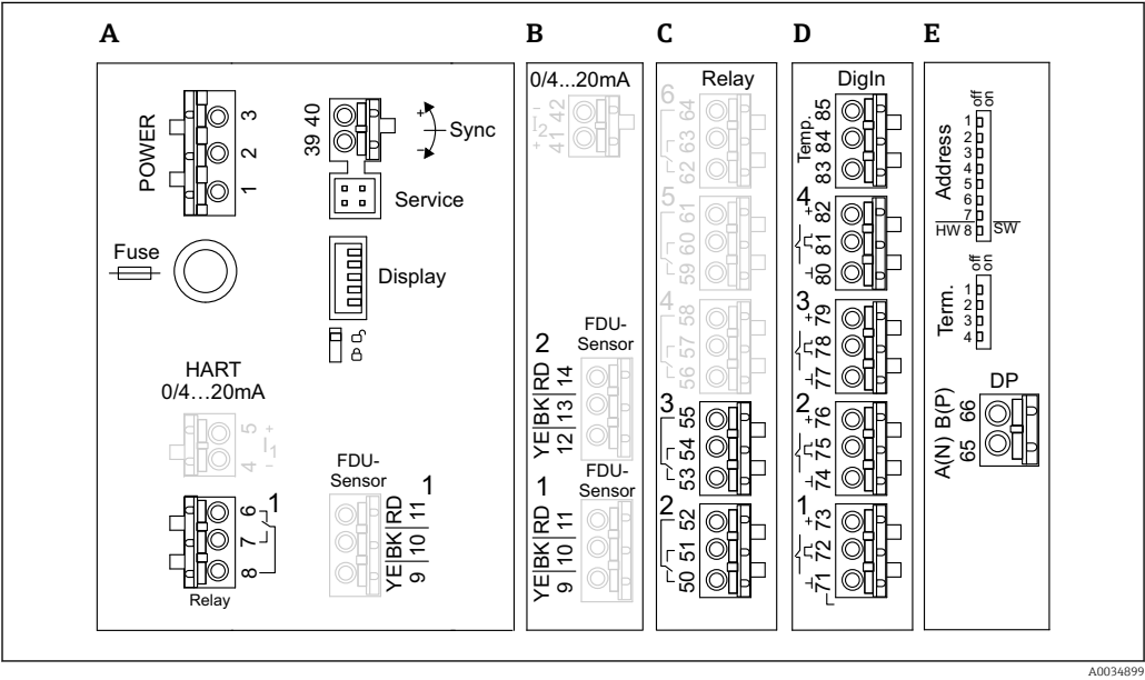
21 Terminal do Prosonic S (os terminais mostrados em cinza não estão disponíveis em todas as versões do equipamento)
