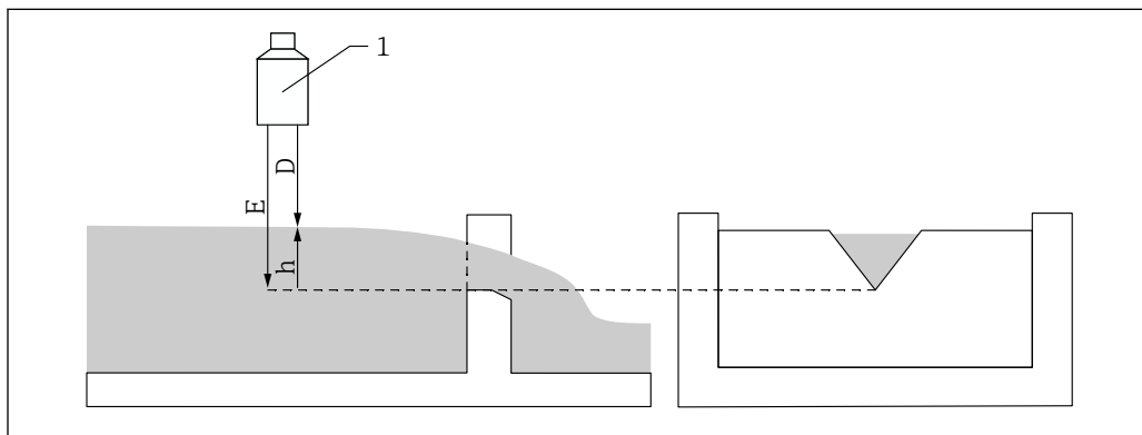
47 Calibração do vazio para canais
