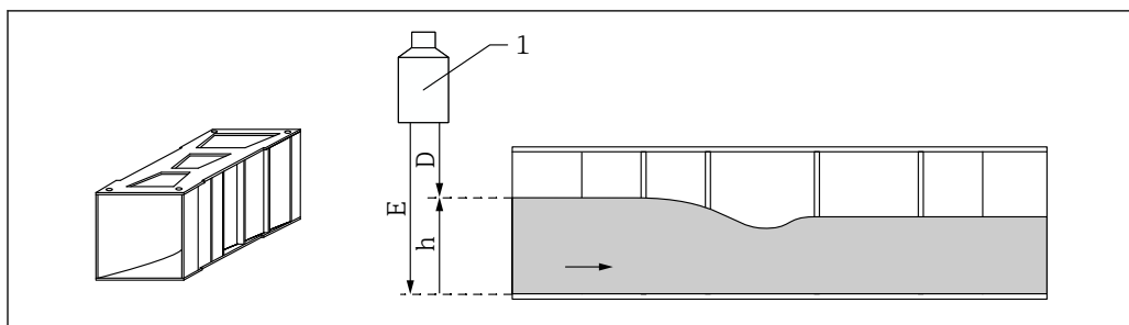
46 Calibração do vazio para calhas
