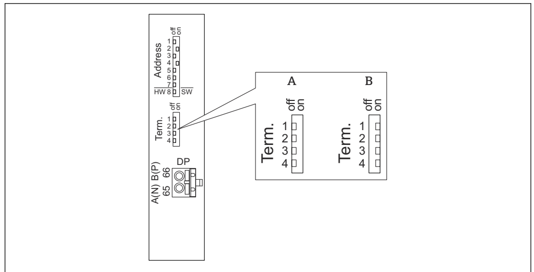
45 Terminação de barramento no equipamento
