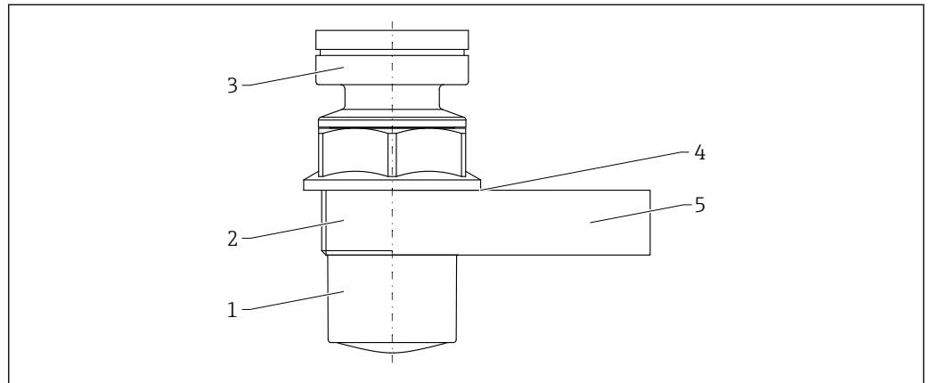
图 35 PVDF 全密封天线（40 mm (1.5 in) 口径）的材质
