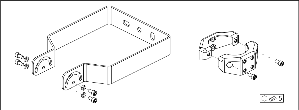
图 43 供货清单; FMR6xB 的安装架 (可调节)
