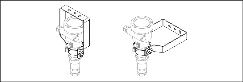
41 FMR6xB 的安装架（可调节）；安装在罐顶或墙壁上
