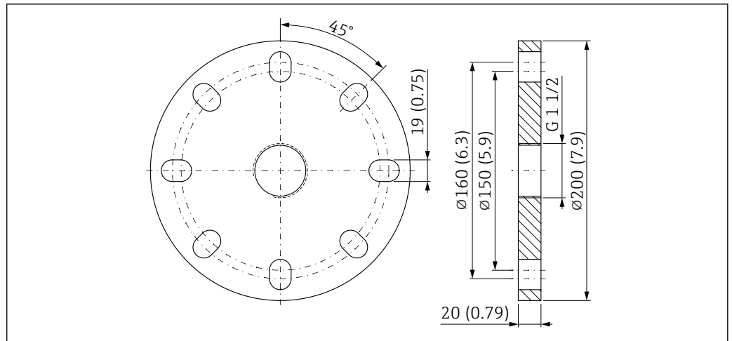
图 32 UNI 3"/DN80/80A 法兰的外形尺寸示意图。测量单位 mm (in)
