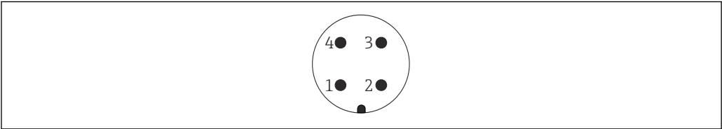
图 6 仪表连接插头示意图
