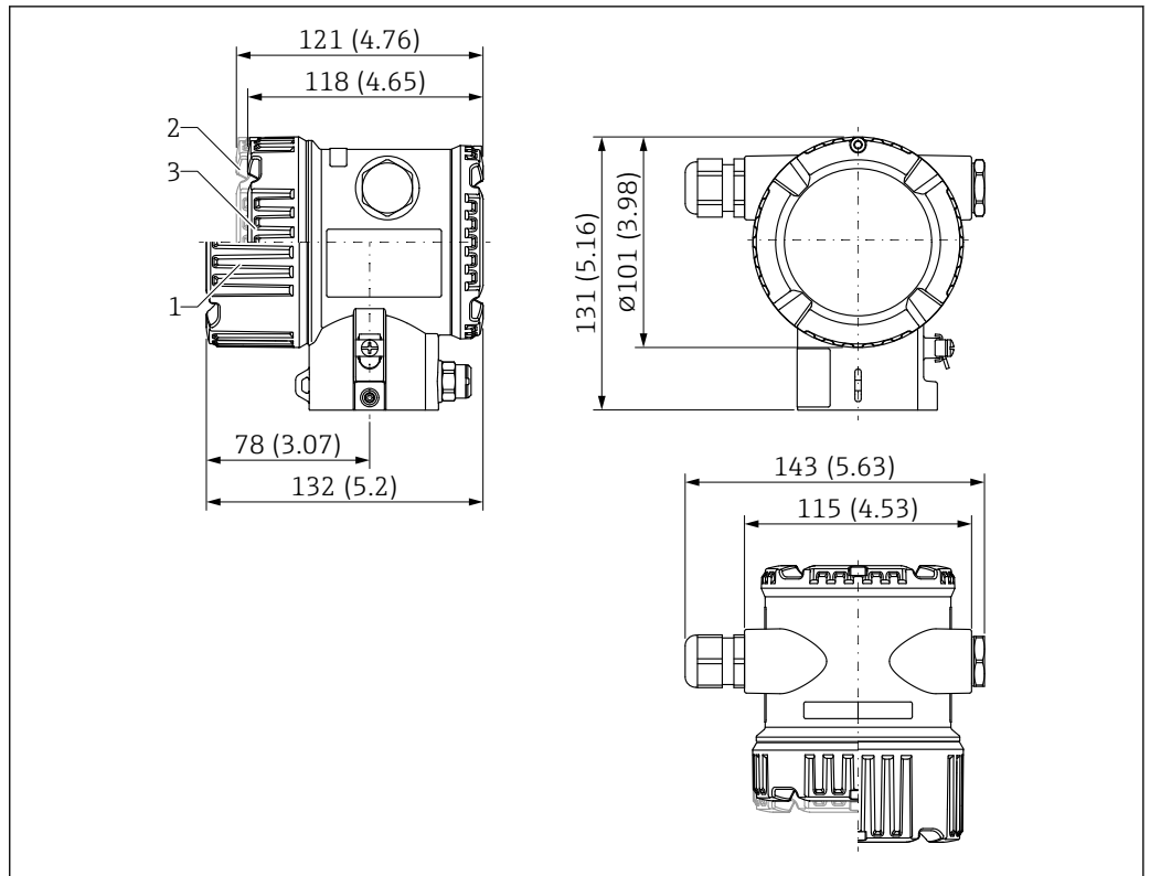
图 22 双腔室铝外壳（带涂层）的外形尺寸示意图；包括 M20 接头和塑料插头。测量单位 mm (in)
