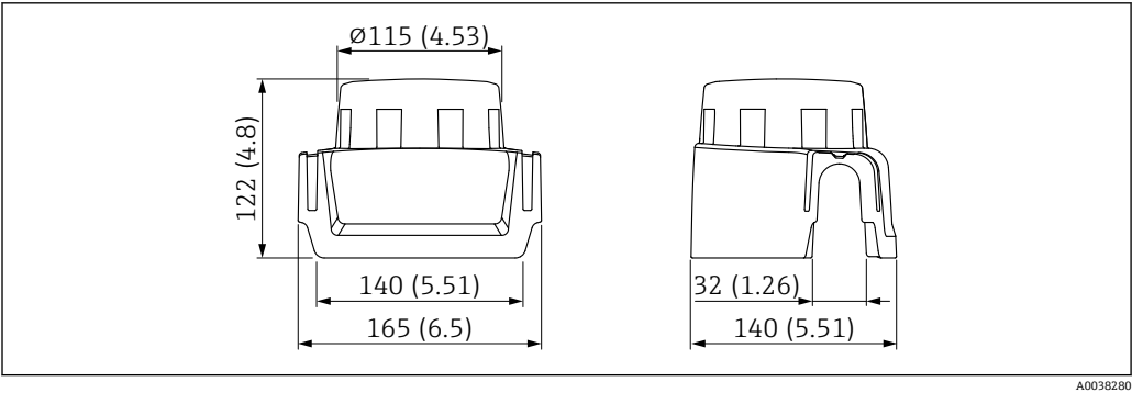
图 40 塑料防护罩 XW111 的外形尺寸示意图。测量单位 mm (in)
