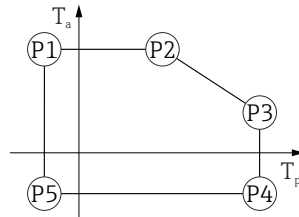
图 15 316L 外壳; 过程温度范围: -40 \dots +80 \text{ }^{\circ}\text{C} ( -40 \dots +176 \text{ }^{\circ}\text{F} )
