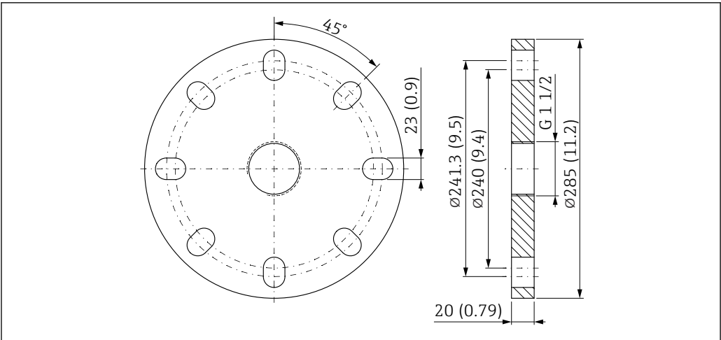
图 34 UNI 6"/DN150/150A 法兰的外形尺寸示意图。测量单位 mm (in)
