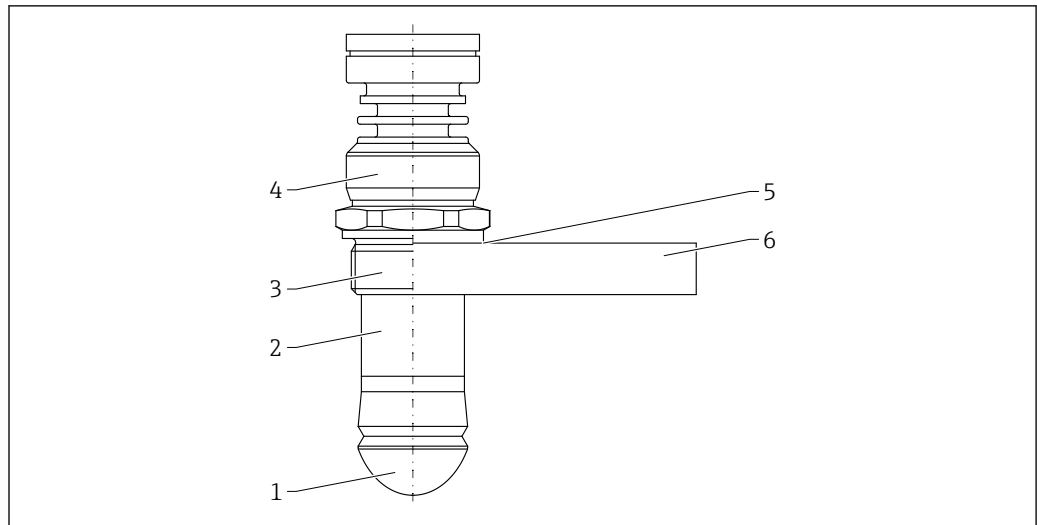
图 36 水滴型天线 (50 mm (2 in) 口径) 的材质
