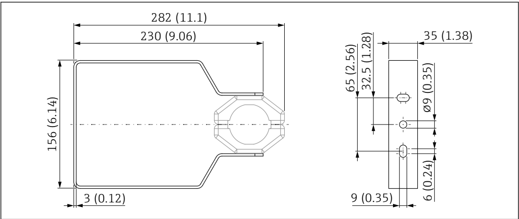
42 外形尺寸示意图；FMR6xB 的安装架（可调节）。测量单位 mm (in)
