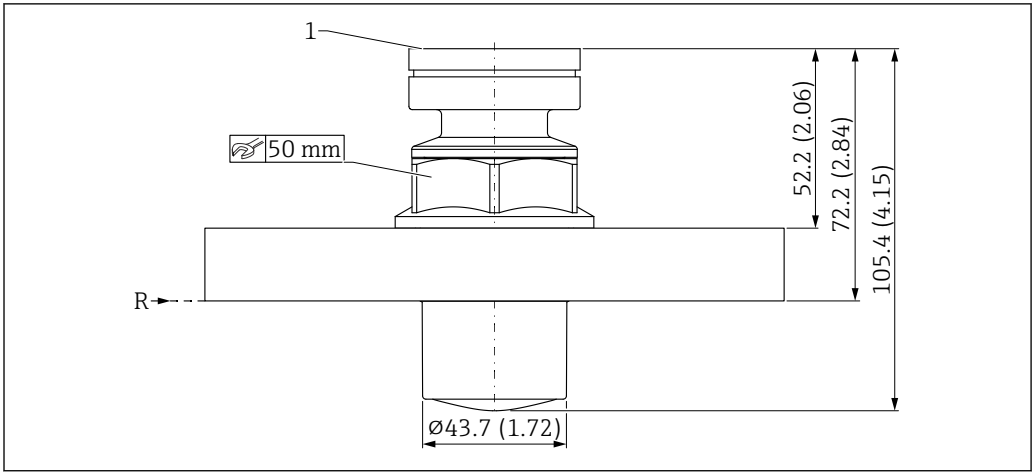
图 26 PVDF 全密封天线（40 mm (1.5 in) 口径）的外形尺寸示意图；UNI 法兰过程连接。测量单位 mm (in)
