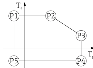
图 13 铝外壳, 带涂层; 过程温度范围: -40 ... +80 °C (-40 ... +176 °F)
