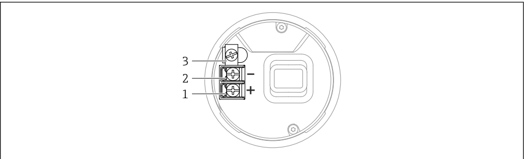
图 3 接线腔内的接线端子和接地端，单腔室外壳
