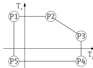
图 14 铝外壳, 带涂层; 过程温度范围: -40 ... +130 °C (-40 ... +266 °F)
