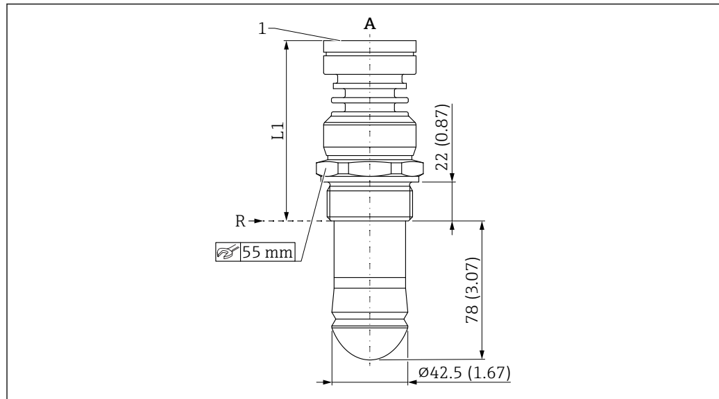
图 30 水滴型天线 (50 mm (2 in) 口径) 的外形尺寸示意图，螺纹过程连接
