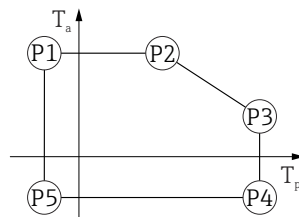
图 11 塑料外壳; 过程温度范围: -40 \dots +130 \text{ }^{\circ}\text{C} ( -40 \dots +266 \text{ }^{\circ}\text{F} )
