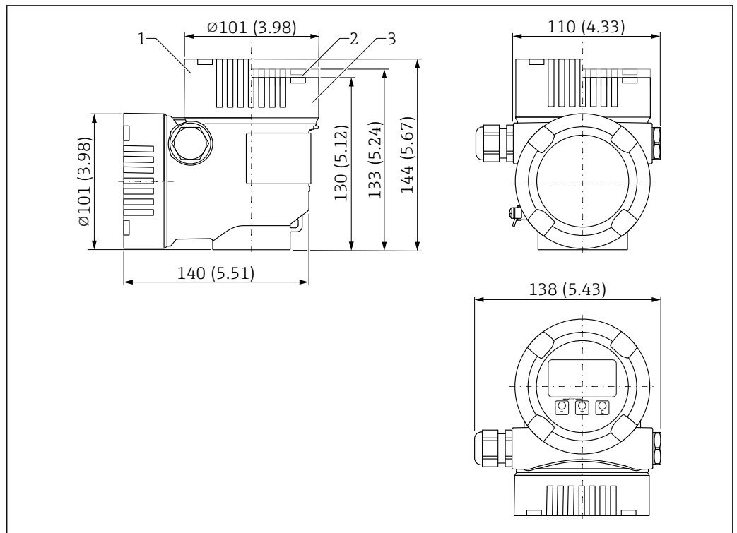
图 24 L 型双腔室 316L 外壳的外形尺寸示意图；包括 M20 接头和塑料插头。测量单位 mm (in)
