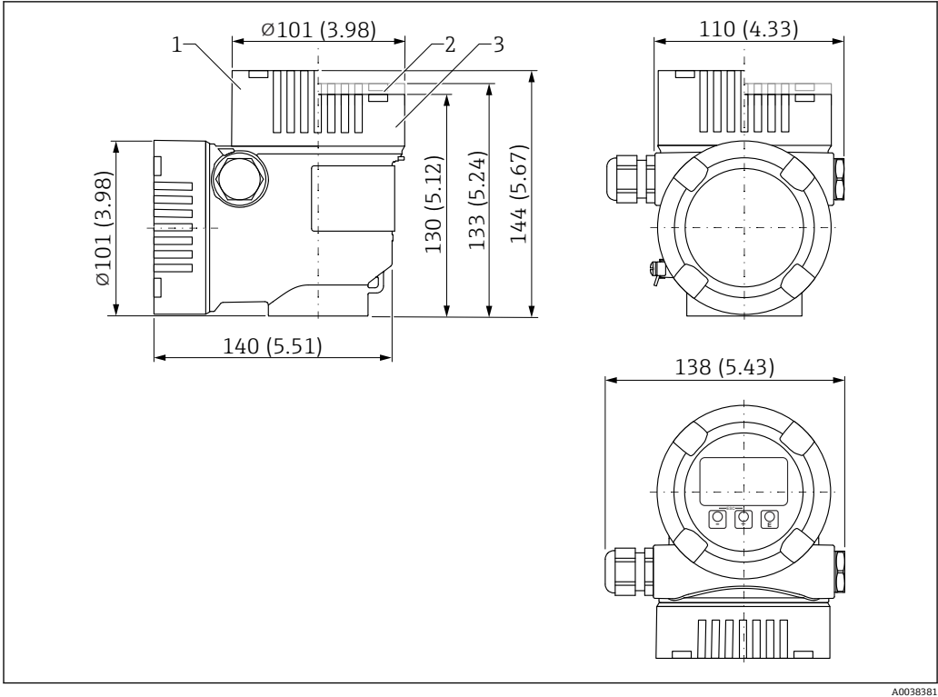
图 23 L 型双腔室铝外壳（带涂层）的外形尺寸示意图；包括 M20 接头和塑料插头。测量单位 mm (in)
