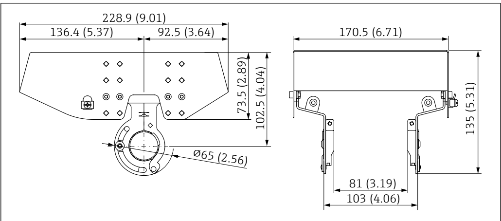
图 39 316L 防护罩 XW112 的外形尺寸示意图。测量单位 mm (in)
