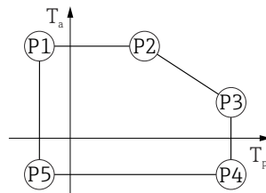
图 17 316L 外壳, 卫生型; 过程温度范围: -40 \dots +80 \text{ }^{\circ}\text{C} ( -40 \dots +176 \text{ }^{\circ}\text{F} )
