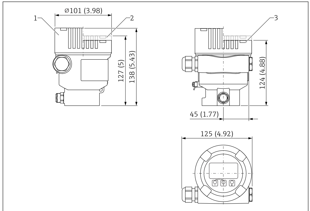
图 20 单腔室铝外壳（带涂层）的外形尺寸示意图；包括 M20 接头和塑料插头。测量单位 mm (in)
