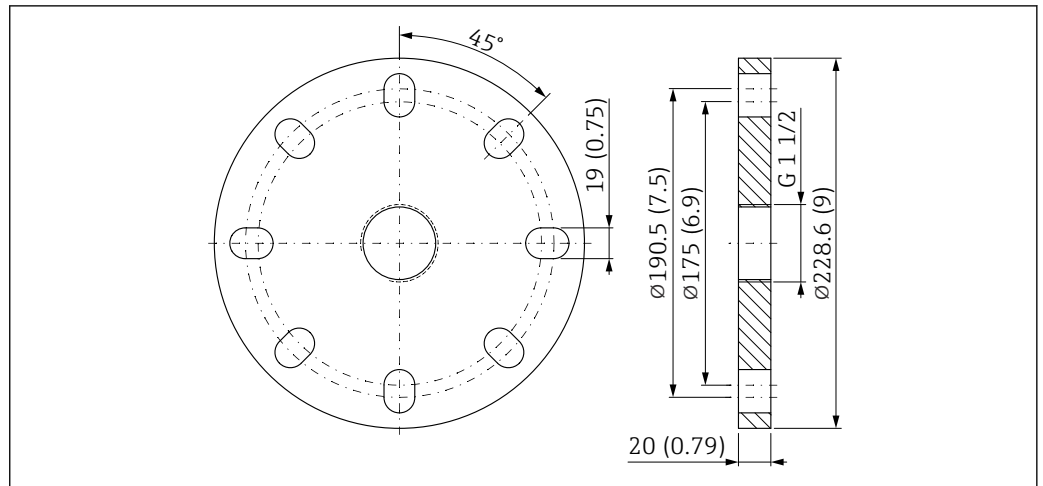
图 28 UNI 4"/DN100/100A 法兰的外形尺寸示意图。测量单位 mm (in)
