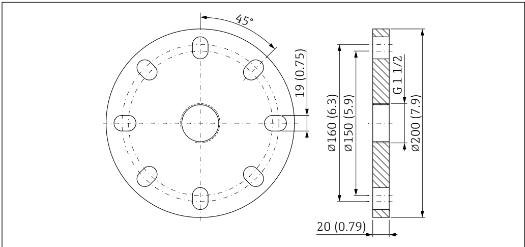
图 27 UNI 3"/DN80/80A 法兰的外形尺寸示意图。测量单位 mm (in)
