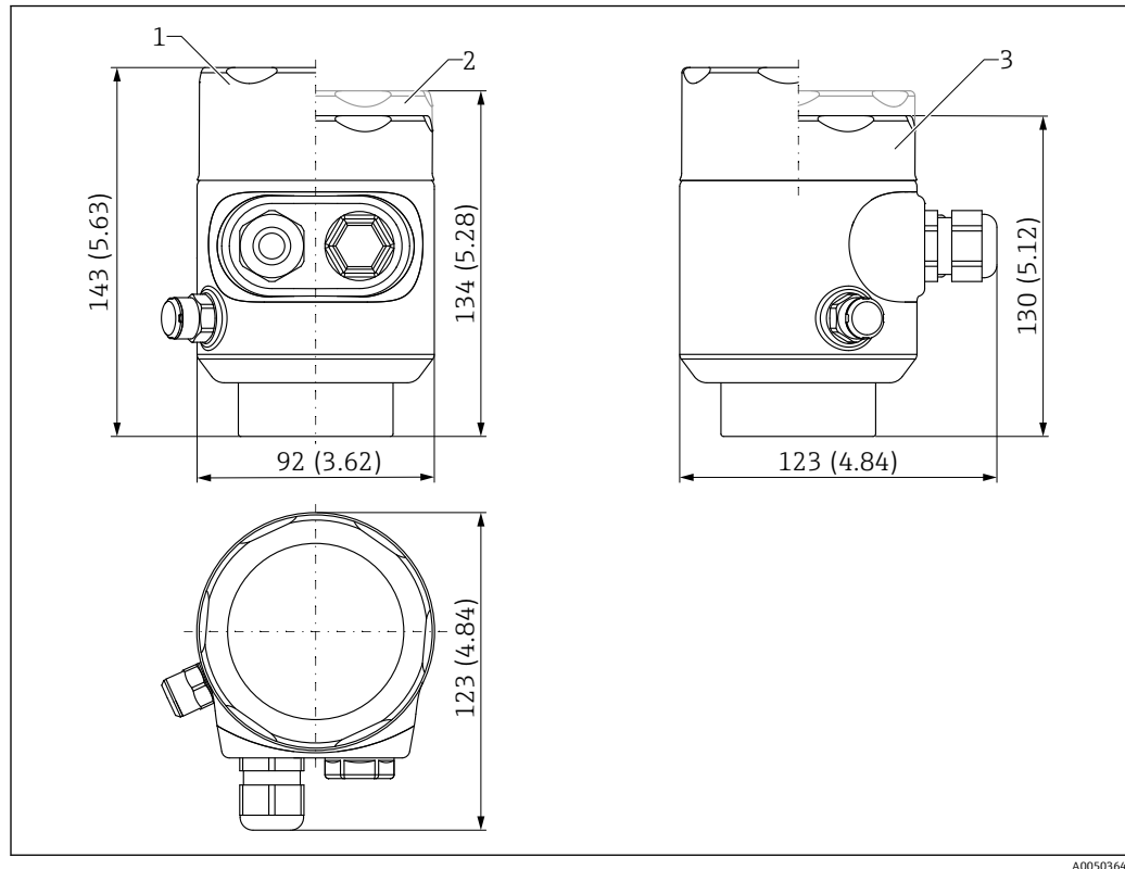
图 21 316L 单腔室外壳（卫生型）的外形尺寸示意图；包括 M20 接头和塑料插头。测量单位 mm (in)
