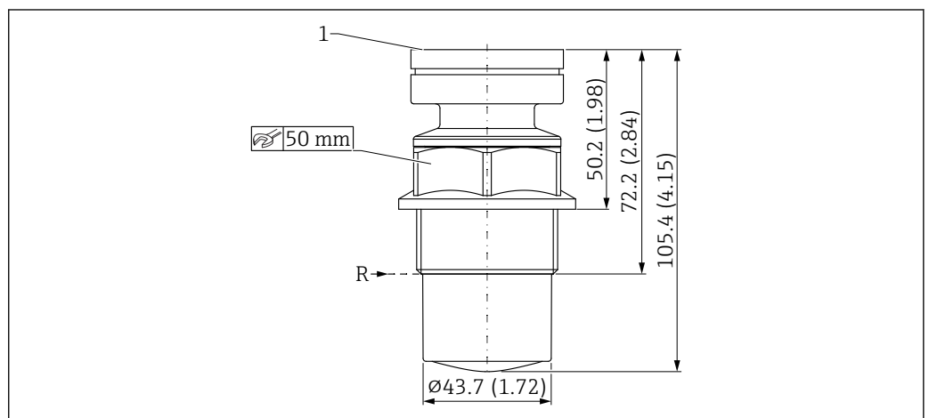
图 25 PVDF 全密封天线 (40 mm (1.5 in) 口径) 的外形尺寸示意图。测量单位 mm (in)
