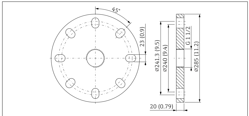
图 29 UNI 6"/DN150/150A 法兰的外形尺寸示意图。测量单位 mm (in)
