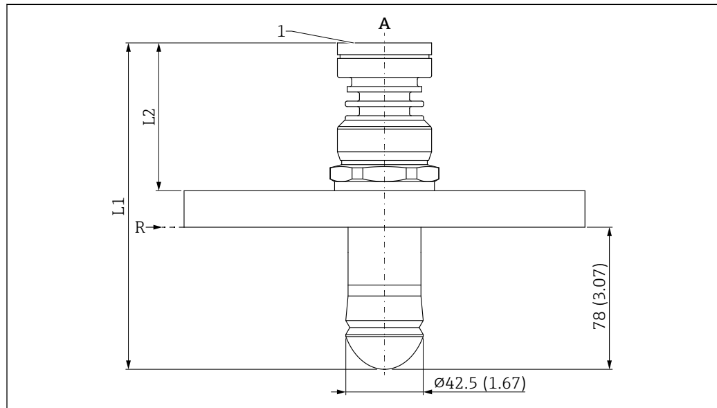
图 31 水滴型天线 (50 mm (2 in) 口径) 的外形尺寸示意图；UNI 法兰过程连接。测量单位 mm (in)
