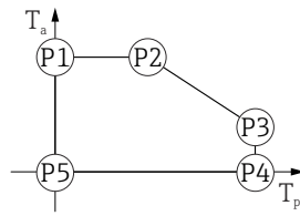
图 12 塑料外壳; 过程温度范围: 0 ... +130 °C (+32 ... +266 °F), 适用 CSA C/US 认证型仪表
