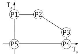
图 10 塑料外壳; 过程温度范围: 0 \dots +80 \text{ }^{\circ}\text{C} ( +32 \dots +176 \text{ }^{\circ}\text{F} ), 适用 CSA C/US 认证型仪表
