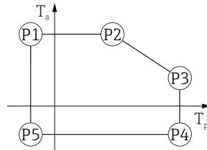
图 16 316L 外壳; 过程温度范围: -40 \dots +130 \text{ }^{\circ}\text{C} ( -40 \dots +266 \text{ }^{\circ}\text{F} )
