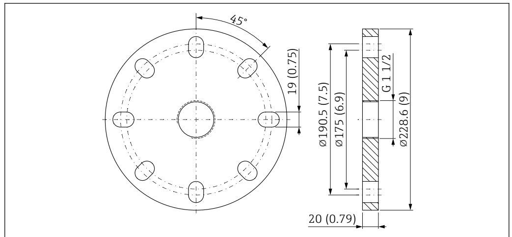
图 33 UNI 4"/DN100/100A 法兰的外形尺寸示意图。测量单位 mm (in)
