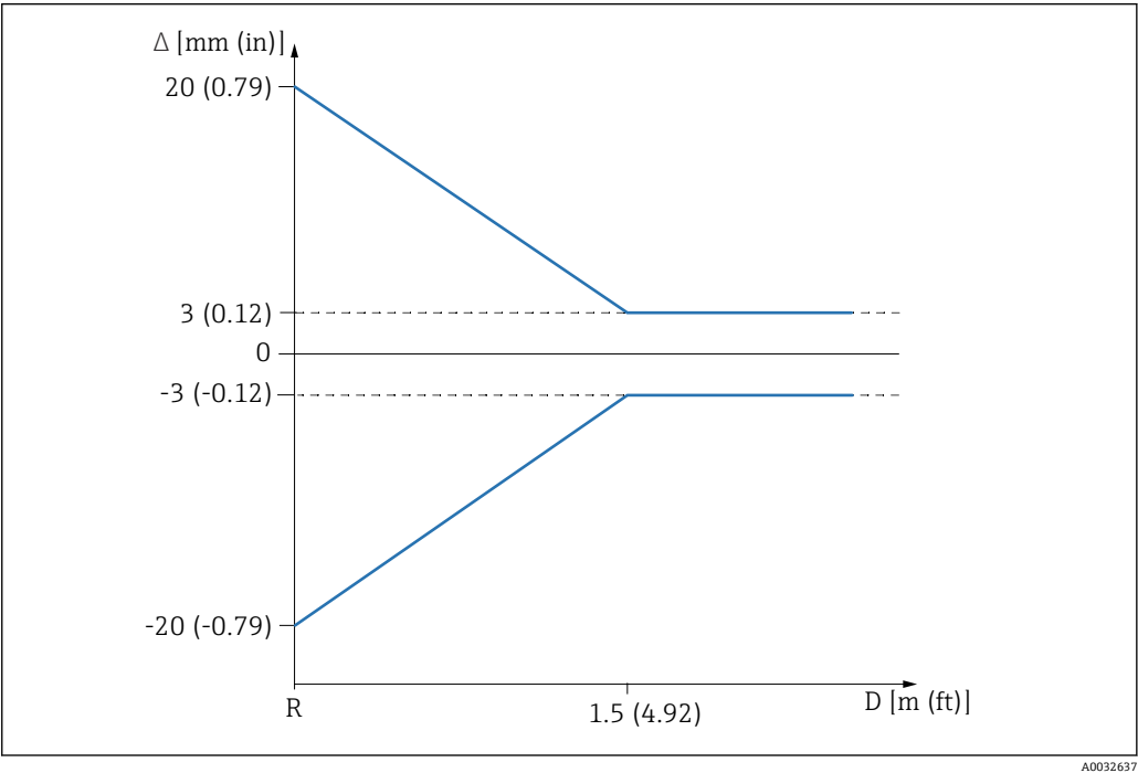
图 7 近距离测量时的最大测量误差
