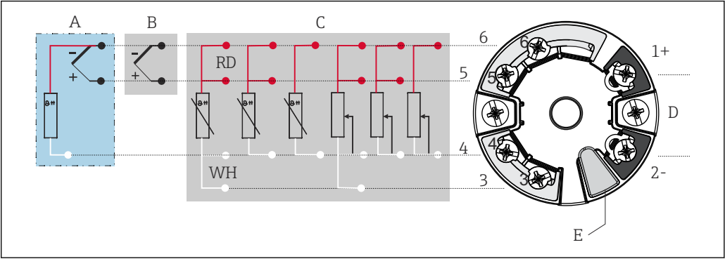
图 3 模块化温度变送器的接线端子分配
