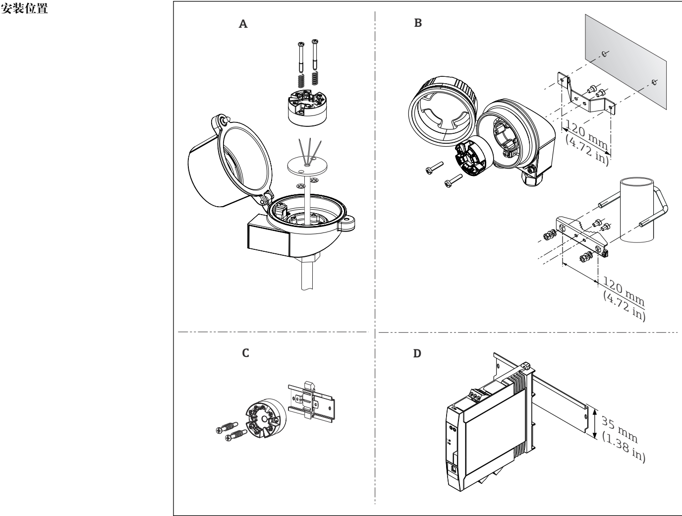
5 变送器安装位置 A 安装在符合 DIN EN 50446 标准的 B 类接线盒中，直接固定在带电缆入口的铠装芯子上（中心孔径：7 mm (0.28 in)） B 分体式安装在现场型外壳中，允许墙装或管装 C 使用导轨夹安装在 DIN 导轨上，TH35 导轨符合 IEC 60715 标准 D DIN 导轨式温度变送器，安装在符合 IEC 60715 标准的 DIN 导轨上（TH35）
