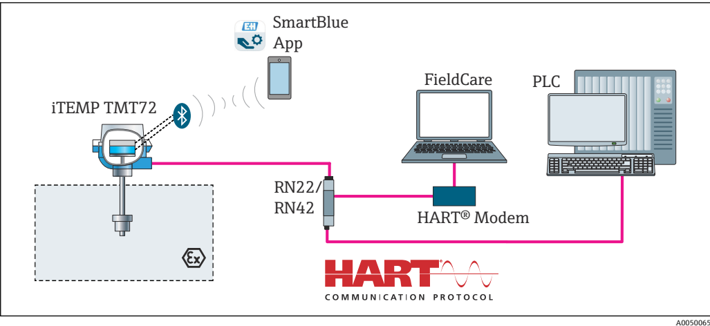
HART 通信的设备架构
