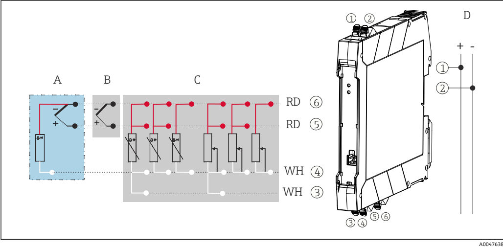
图 4 DIN 导轨式温度变送器的接线端子分配示意图 A 传感器输入，热电偶 (TC) 和电压 (mV) 信号，外部冷端 (CJ)，Pt100 B 传感器输入，热电偶 (TC) 和电压 (mV) 信号，内部冷端 (CJ) C 传感器输入，热电阻 (RTD) 和电阻 (Ω) 信号，四线制、三线制和两线制连接 D 总线终端电阻和 4 ... 20 mA 电源
