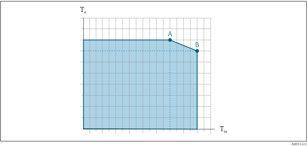
43 Representación ejemplar, valores en la tabla siguiente. T_a Temperatura ambiente T_m Temperatura del producto A Máxima temperatura admisible del producto T_m a T_{a\,máx} = 60\text{ °C} (140 °F); las temperaturas de producto superiores T_m requieren una reducción en la temperatura ambiente T_a B Temperatura ambiente máxima admisible T_a para la temperatura máxima del producto especificada T_m del sensor
