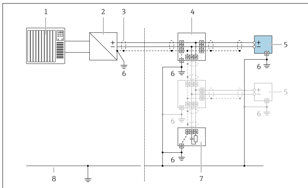
Fig. 16 Ejemplo de conexión para FOUNDATION Fieldbus
