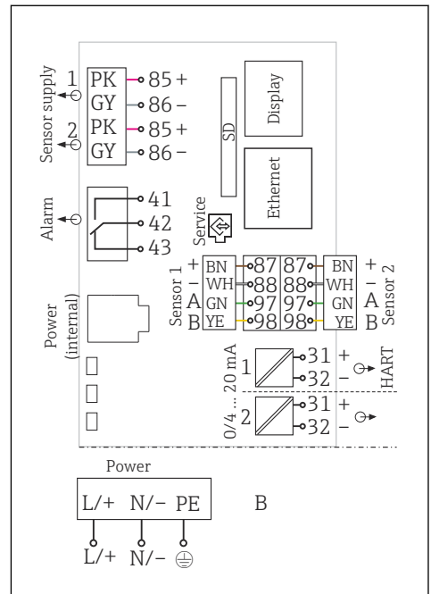
9 Diagrama de conexionado completo con el ejemplo del BASE2-E y fuente de alimentación externa (B)
