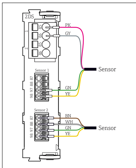
13 Sensores con y sin tensión de alimentación adicional en el módulo del sensor 2DS
