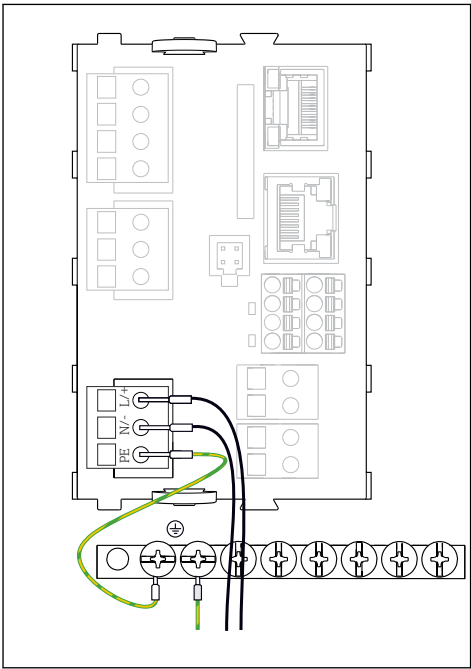
6 Conexión de la fuente de alimentación mediante el ejemplo del BASE2-H o -L
