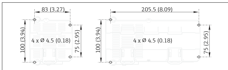
2 Esquema de taladros para montaje en pared en mm (pulgadas)
