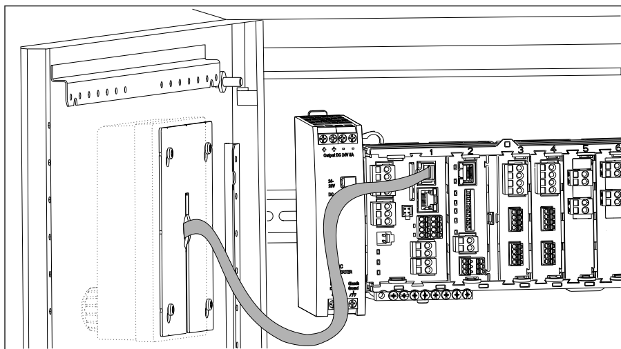
5 Indicador montado
