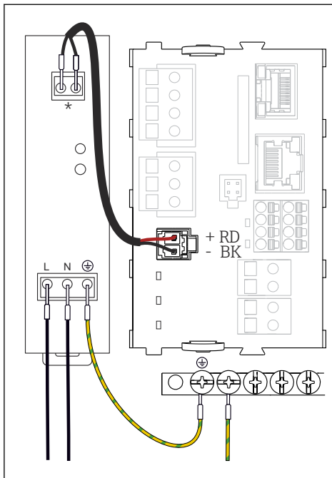
8 Conexión de la fuente de alimentación con el ejemplo del BASE2-E
