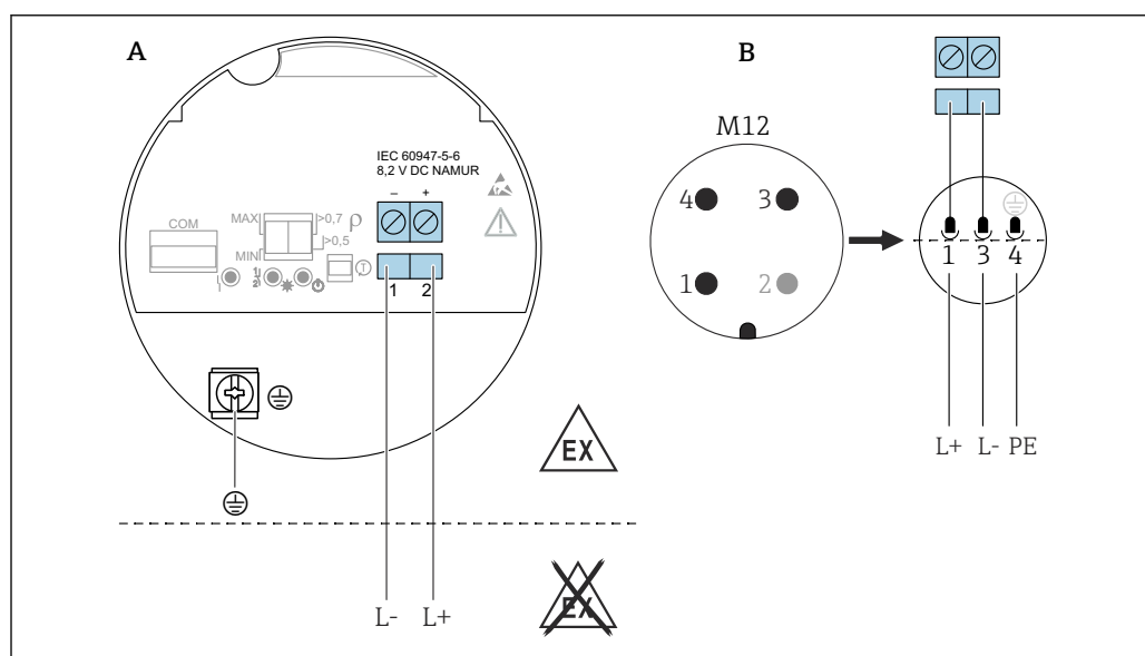
図 29 2 線式 NAMUR \geq 2.2 \text{ mA} / \leq 1.0 \text{ mA} 、エレクトロニックインサート FEL68
