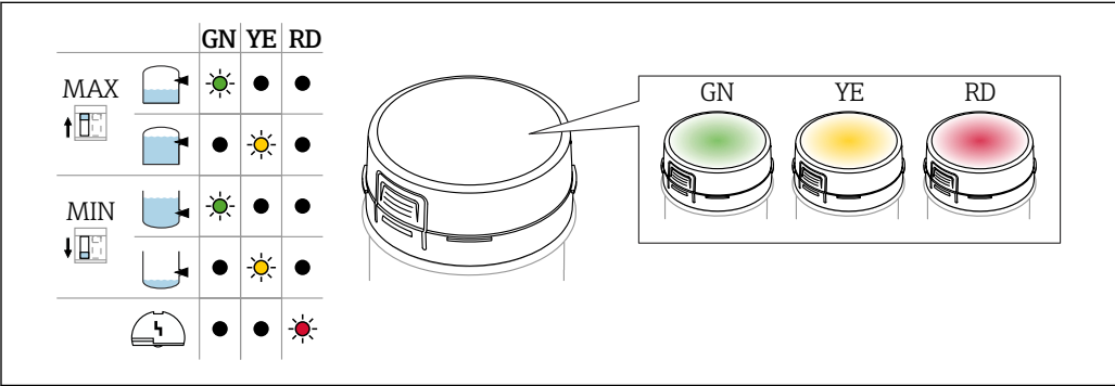
図 31 LED モジュール：LED は緑色（GN）、黄色（YE）または赤色（RD）に点灯します。
