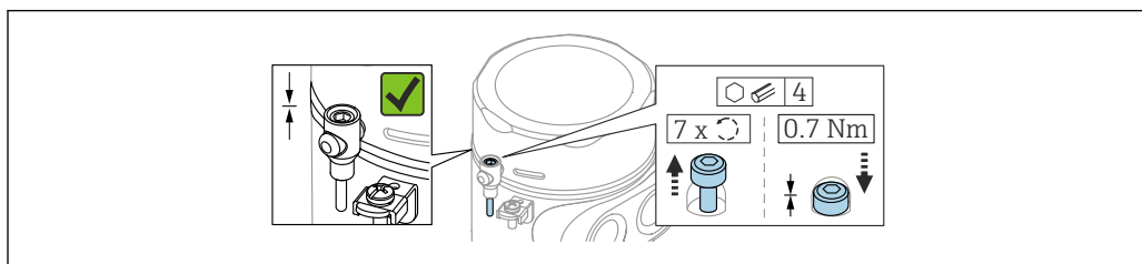
図 17 固定ねじ付きカバー；サニタリハウジング（粉塵防爆仕様のみ）
