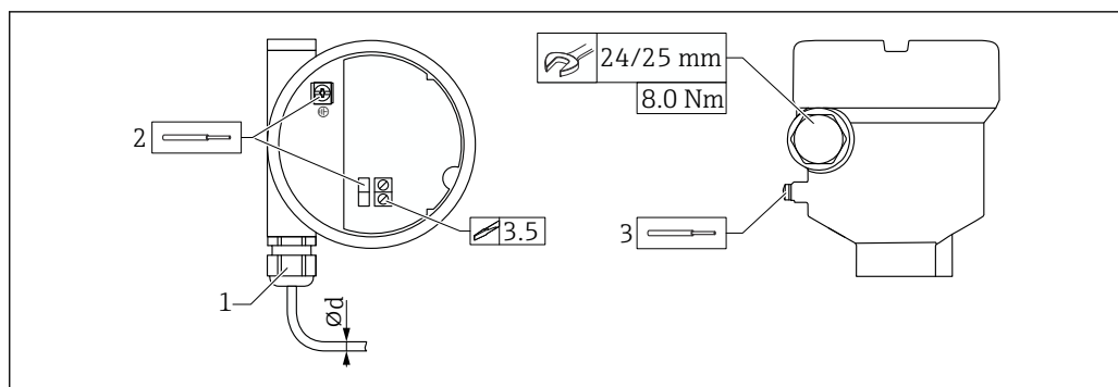
図 33 カップリングの例（電線口、エレクトロニックインサートと端子）
