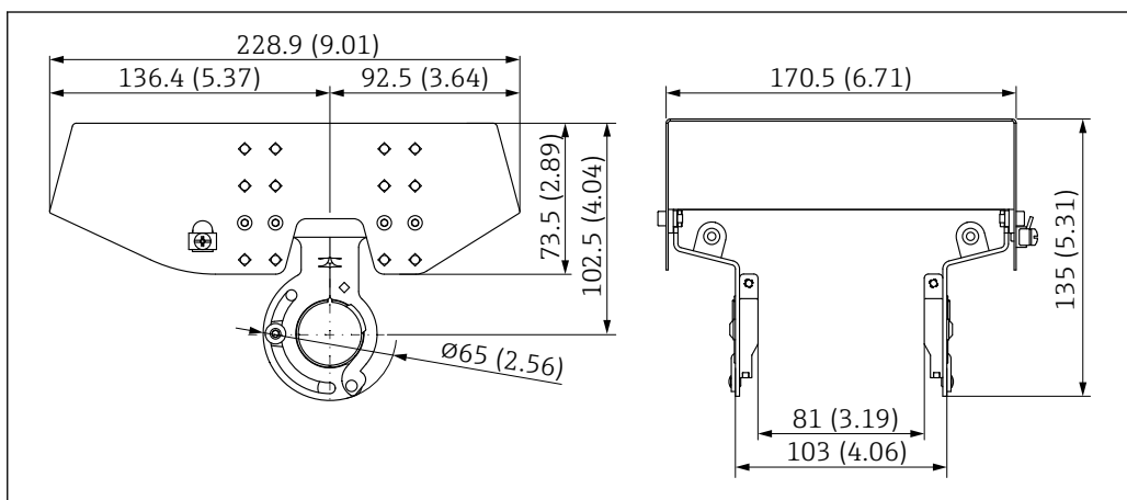
47 保護カバー、SUS 316L 相当、XW112 の寸法。測定単位 mm (in)
