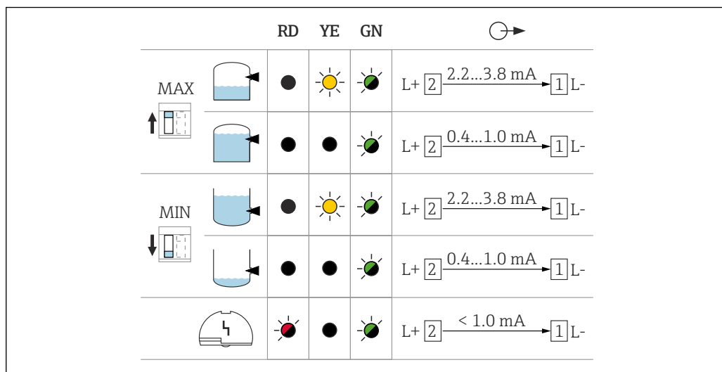
図 30 スwitch出力および信号伝達の動作、エレクトロニクスインサート FEL68
