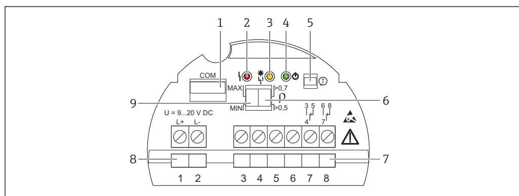
図 34 エレクトロニックインサート FEL64DC の例
