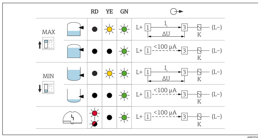
22 スイッチ出力および信号伝達の動作、エレクトロニックインサート FEL62
