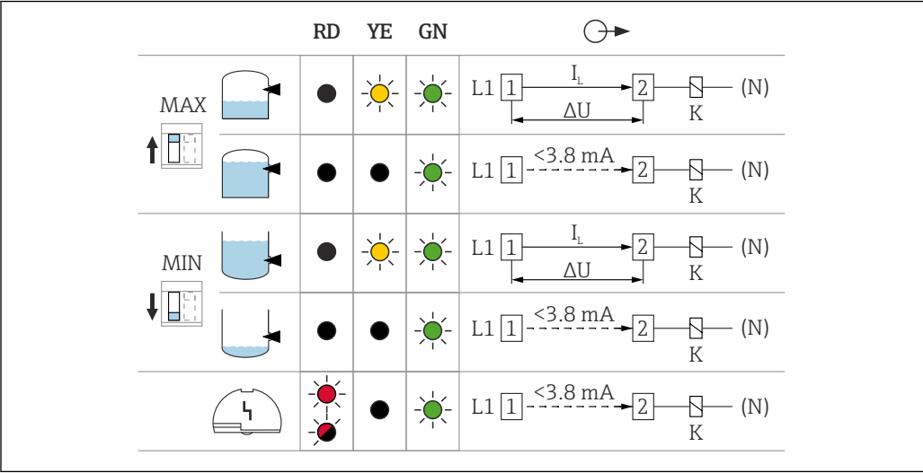
図 19 スwitch出力および信号伝達の動作、エレクトロニックインサート FEL61
