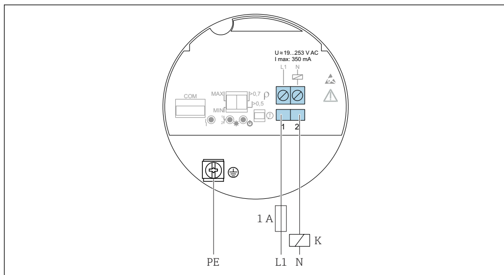
18 2 線式 AC、エレクトロニックインサート FEL61
