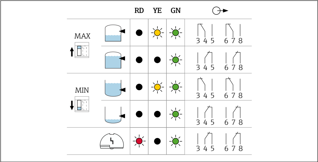
図 24 スイッチ出力および信号伝達の動作、エレクトロニックインサート FEL64
