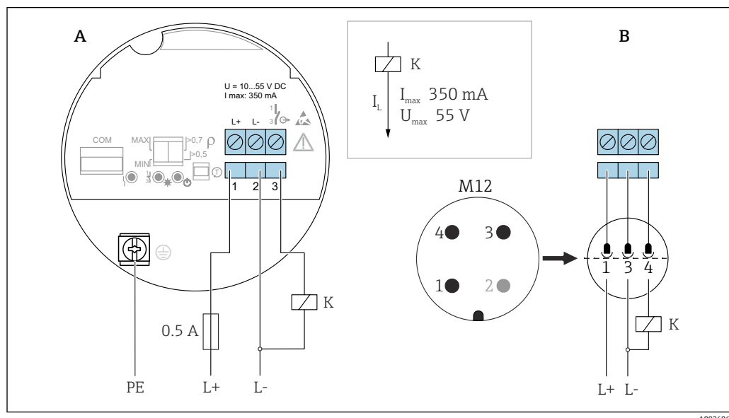
21 3線式DC-PNP、エレクトロニックインサート FEL62
