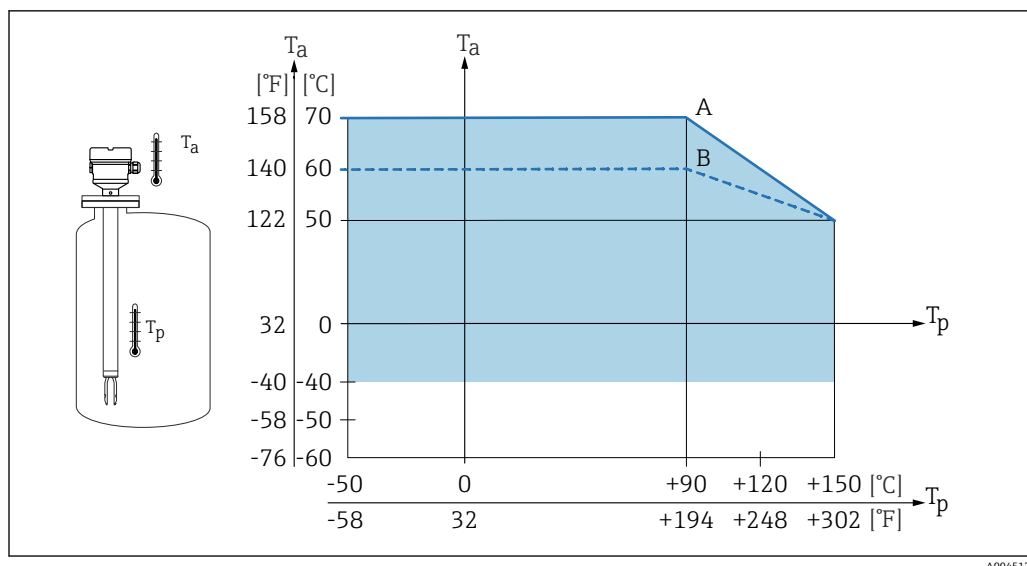
図 51 容器内のプロセス温度 T_p に応じたハウジングの許容周囲温度 T_a
