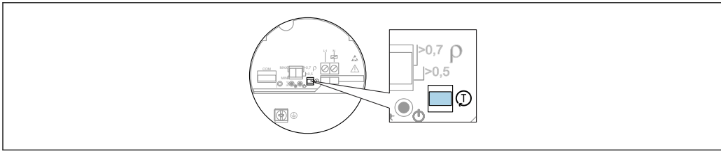
図 36 機能テスト用のボタン (エレクトロニックインサート FEL61/62/64/64DC/67/68)
