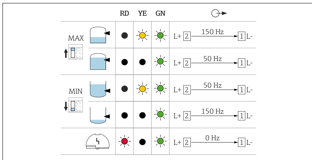
図 28 スイッチング動作および信号伝達、エレクトロニックインサート FEL67
