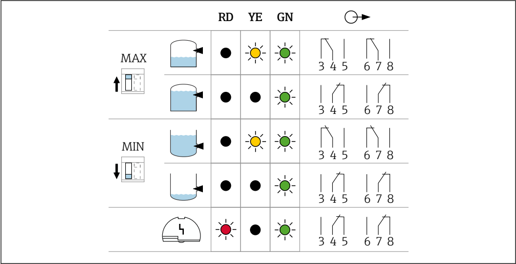
図 26 スwitch出力および信号伝達の動作、エレクトロニックインサート FEL64 DC
