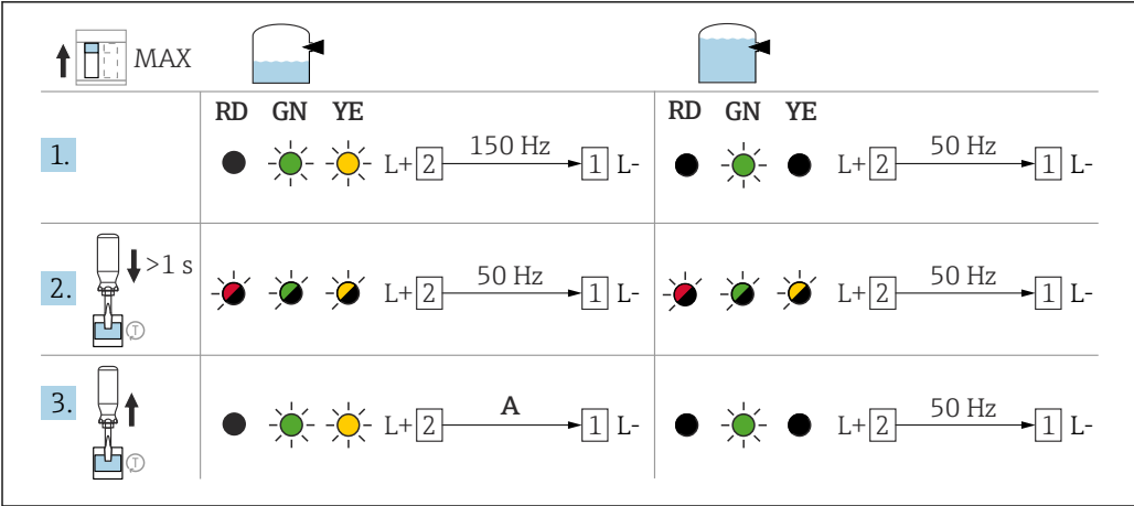
40 FEL67 上限 (MAX) スイッチング動作および信号伝達
