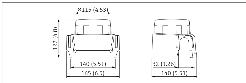
図 48 日除けカバー、プラスチック、XW111 の寸法。測定単位 mm (in)
