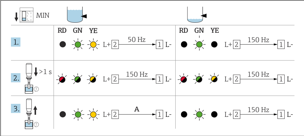
41 FEL67 下限 (MIN) スイッチング動作および信号伝達
