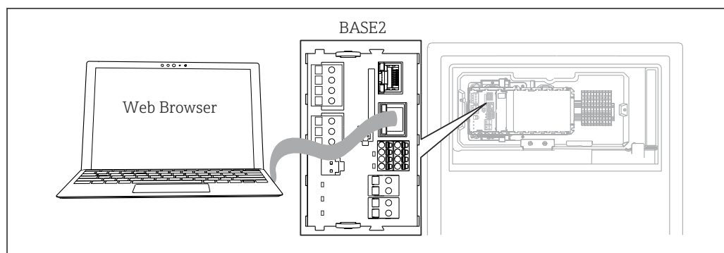
📄 49 Веб-сервер/Ethernet-соединение
