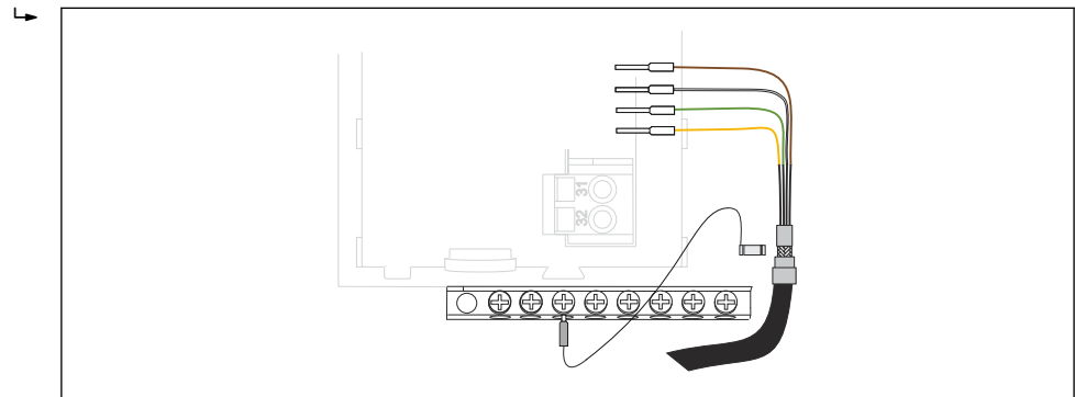
26 Клеммная колодка
