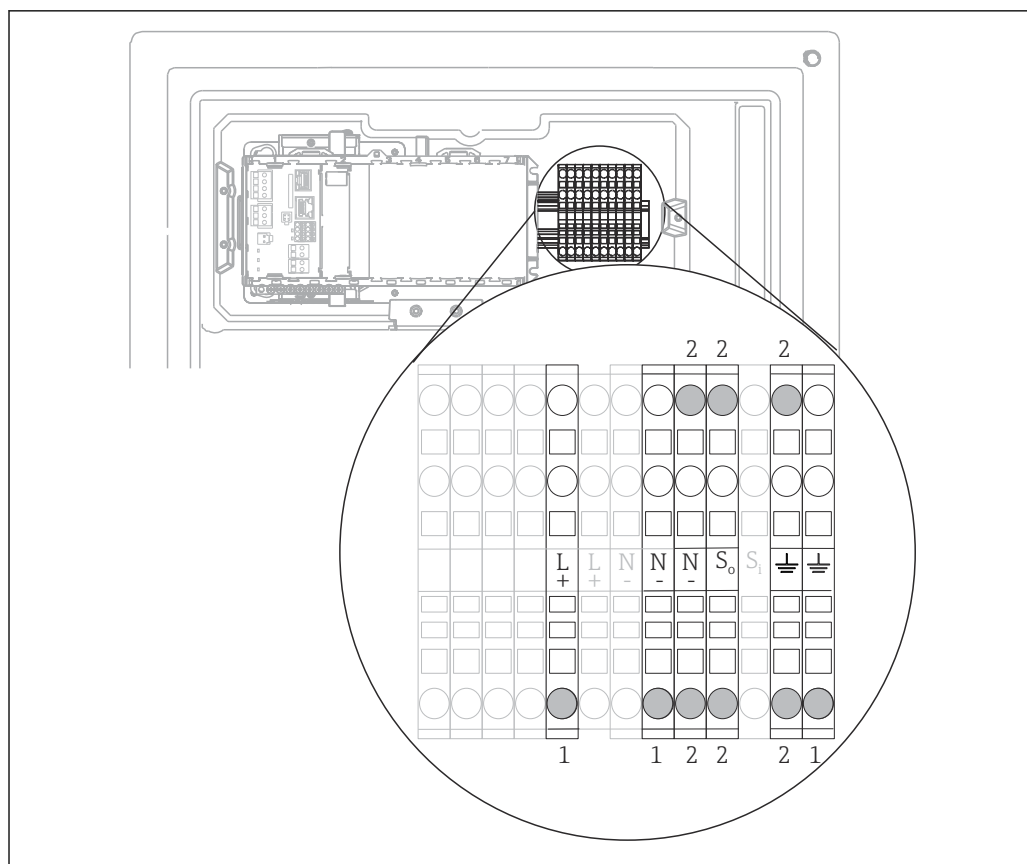
22 Назначение клемм в исполнении, предназначенном для установки вне помещений
