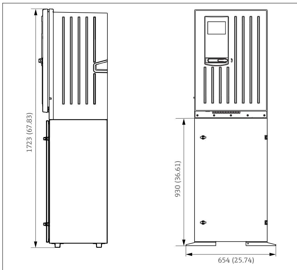
10 С базой. Единица измерения мм (дюйм)
