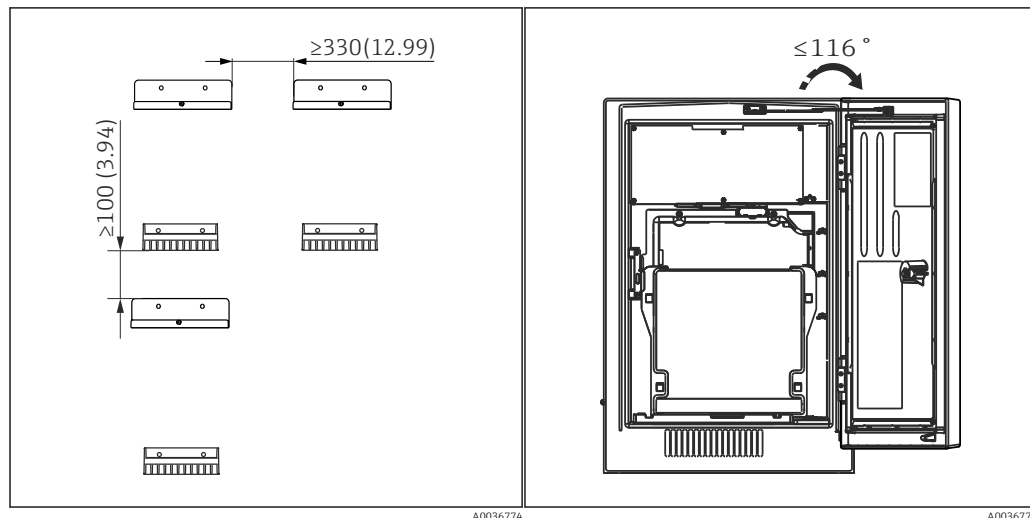
13 Минимальный зазор для монтажа. Единица измерения мм (дюйм) 14 Максимальный угол раскрытия
