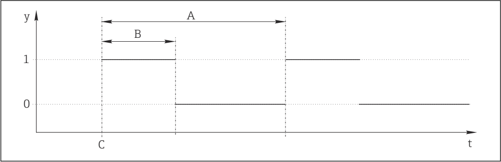
65 Схема сигнала реле времени t Временная шкала y Уровень сигнала (1 – вкл., 0 – выкл.) A Период B Длительность сигнала C Время начала (Дата запуска, Время зап.)
