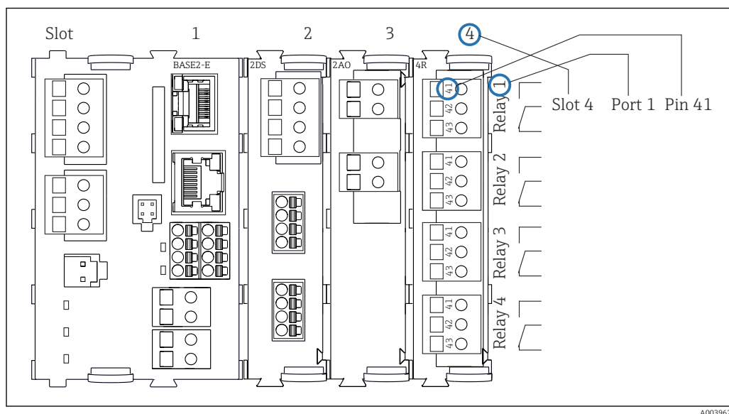
7 Создание схемы контактного вывода на примере нормально разомкнутого контакта (вывод 41) реле
