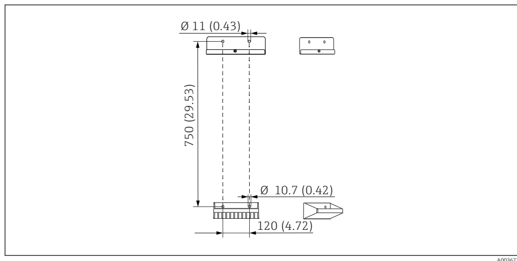
15 Размеры держателя. Единица измерения мм (дюйм)
