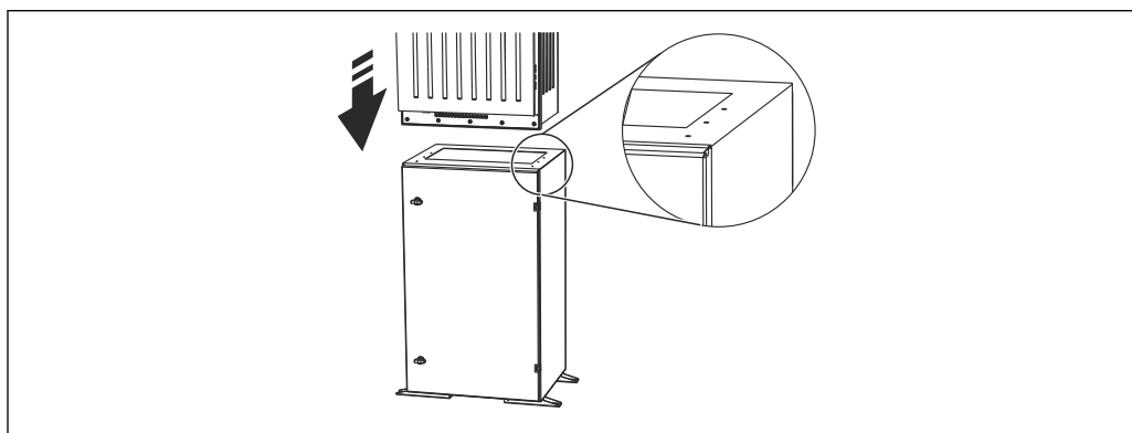
17 Закрепление опоры
