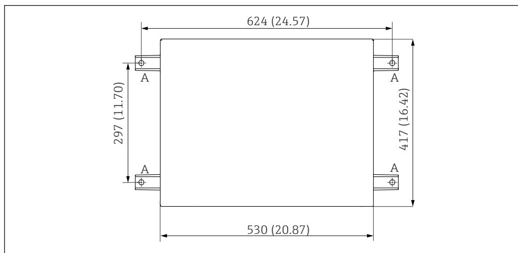
16 План фундамента. Единица измерения мм (дюйм)
