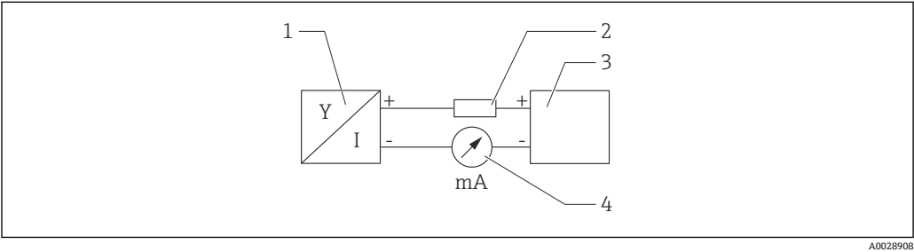
图 4 HART 接线框图
