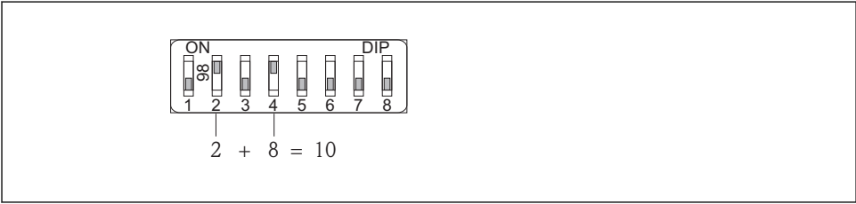
17 Exemplo de endereçamento de hardware: a seletora 8 está na posição "OFF"; as seletoras 1 a 7 definem o endereço.
