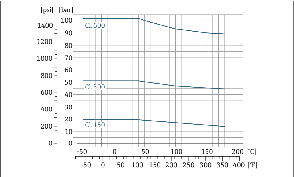
18 法兰材质: 1.4404 (316/316L)
