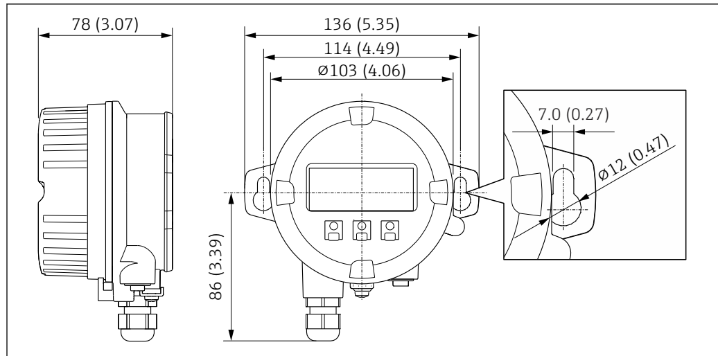
图 23 单位: mm (in)
