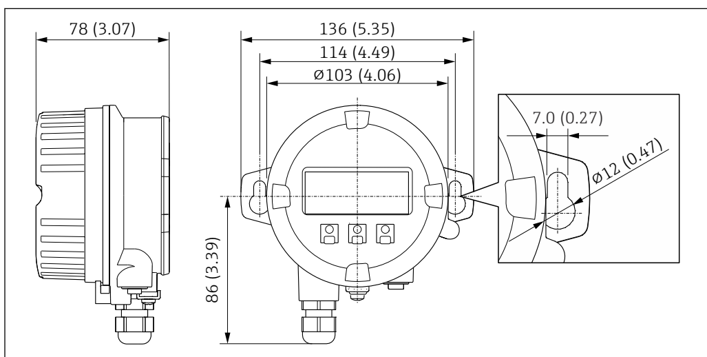
图 29 单位: mm (in)
