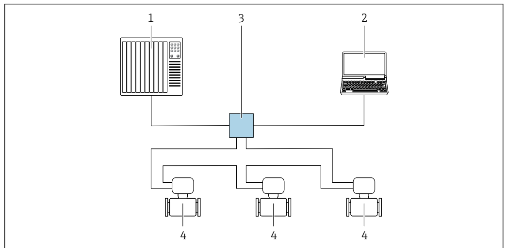
图 46 通过 PROFINET 网络进行远程操作：环形拓扑结构
