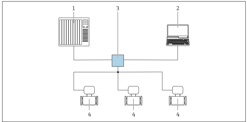
图 45 通过 PROFINET 网络进行远程操作：星形拓扑结构
