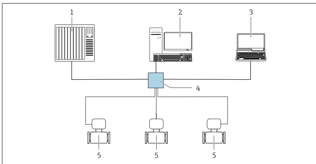
图 43 通过 EtherNet/IP 网络进行远程操作：星形拓扑结构
