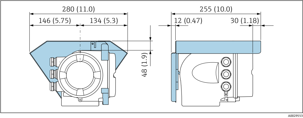
图 15 单位: mm (in)
