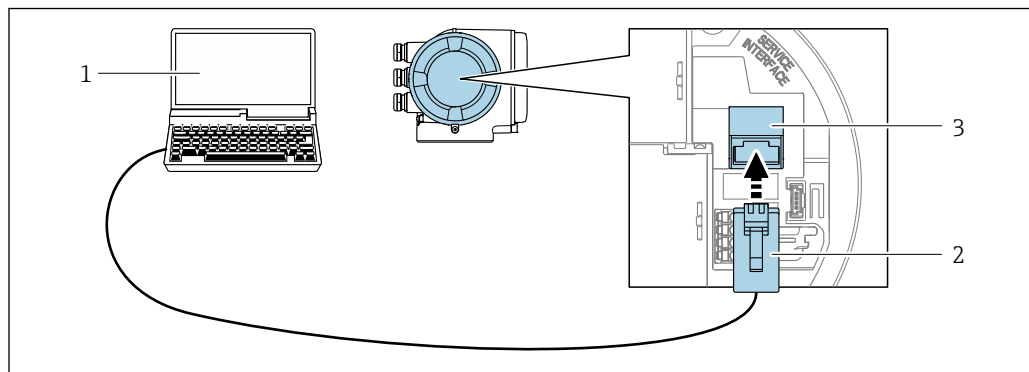
图 47 通过服务接口 (CDI-RJ45) 连接
