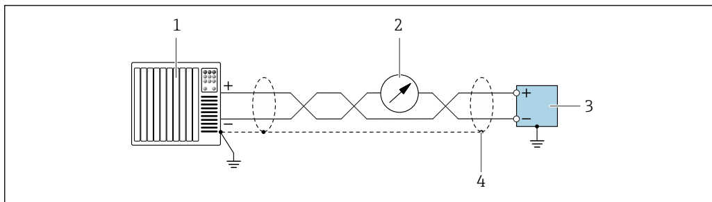
图 9 接线实例：4 ... 20 mA HART 电流输出（有源）
