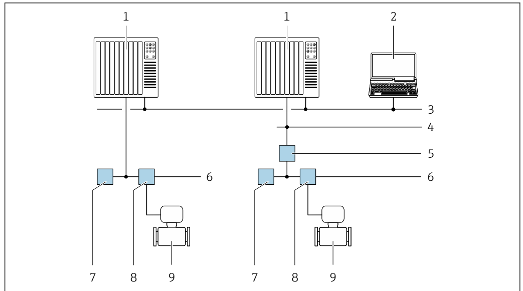
37 通过 FOUNDATION Fieldbus 网络进行远程操作
