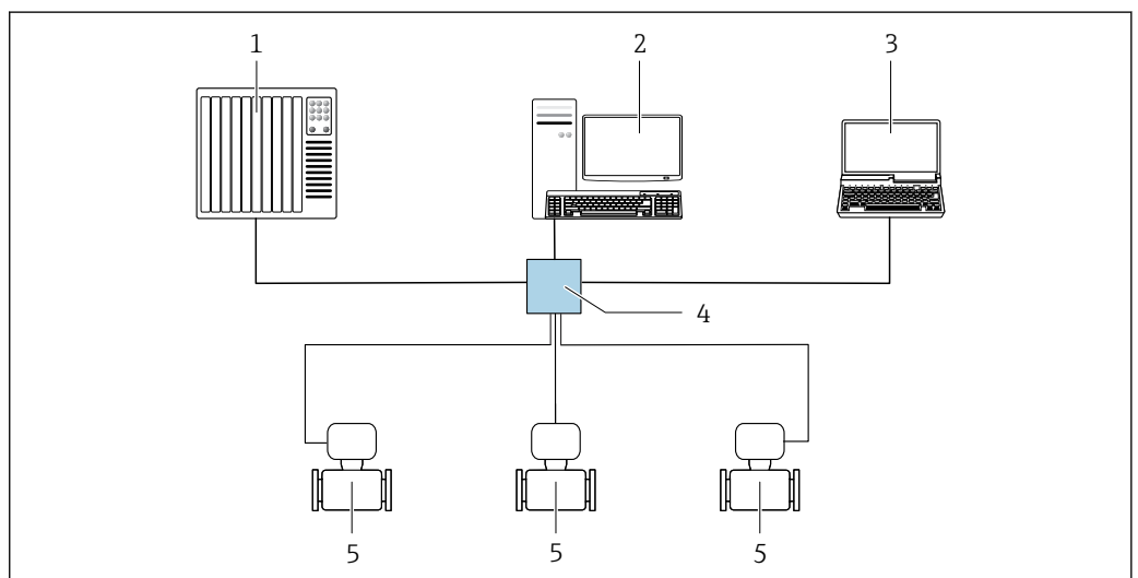
图 42 通过 Modbus TCP + Ethernet 进行远程操作 - 100 Mbit/s: 星形拓扑结构
