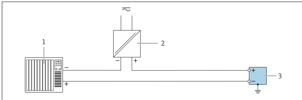
図 25 リレー出力の接続例
