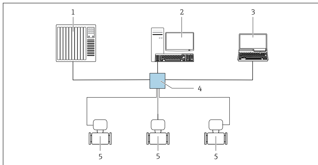
図 32 EtherNet/IP ネットワーク経由のリモート操作用オプション：スター型トポロジー
