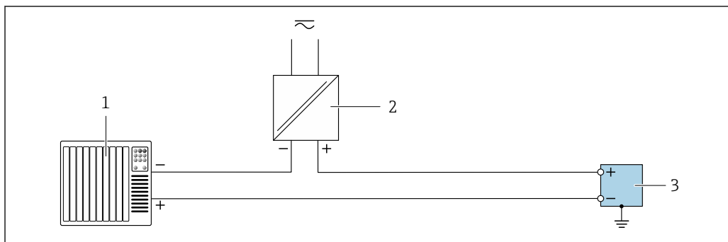
図 24 パルス出力/周波数出力/スイッチ出力（パッシブ）の接続例
