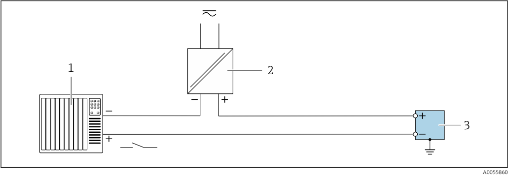
16 Exemple de raccordement pour l'entrée état 1 Système d'automatisation avec sortie tout ou rien passive p. ex. API) 2 Alimentation électrique 3 Transmetteur avec entrée d'état
