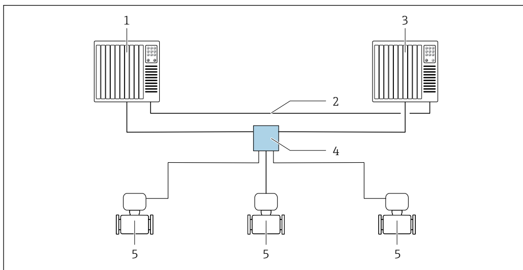
■ 27 Пример компоновки резервируемой системы (S2): топология «звезда»
