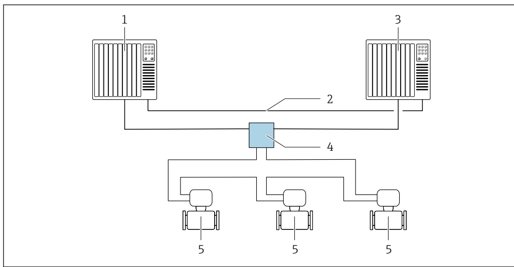
■ 26 Пример компоновки резервируемой системы (S2): кольцевая топология
