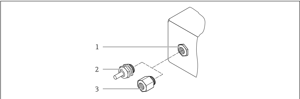
34 Entrées de câble/presse-étoupe possibles 1 Taraudage M20 × 1,5 2 Presse-étoupe M20 × 1,5 3 Adaptateur pour entrée de câble avec taraudage G ½" ou NPT ½"
