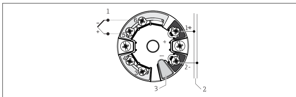
図 6 ヘッド組込型伝送器 iTEMP TMT7x または iTEMP TMT31 (1 センサ入力)
