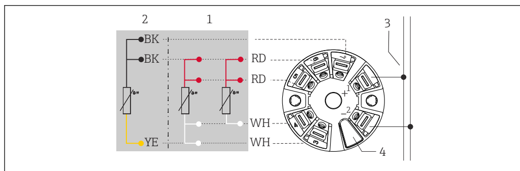
図 4 iTEMP TMT8x ヘッド組込型伝送器 (2 センサ入力)
