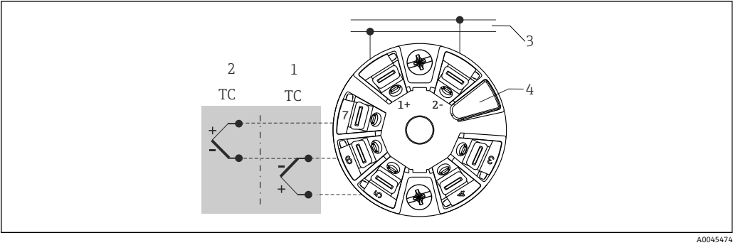
7 iTEMP TMT8x ヘッド組込型伝送器 (2 センサ入力)
