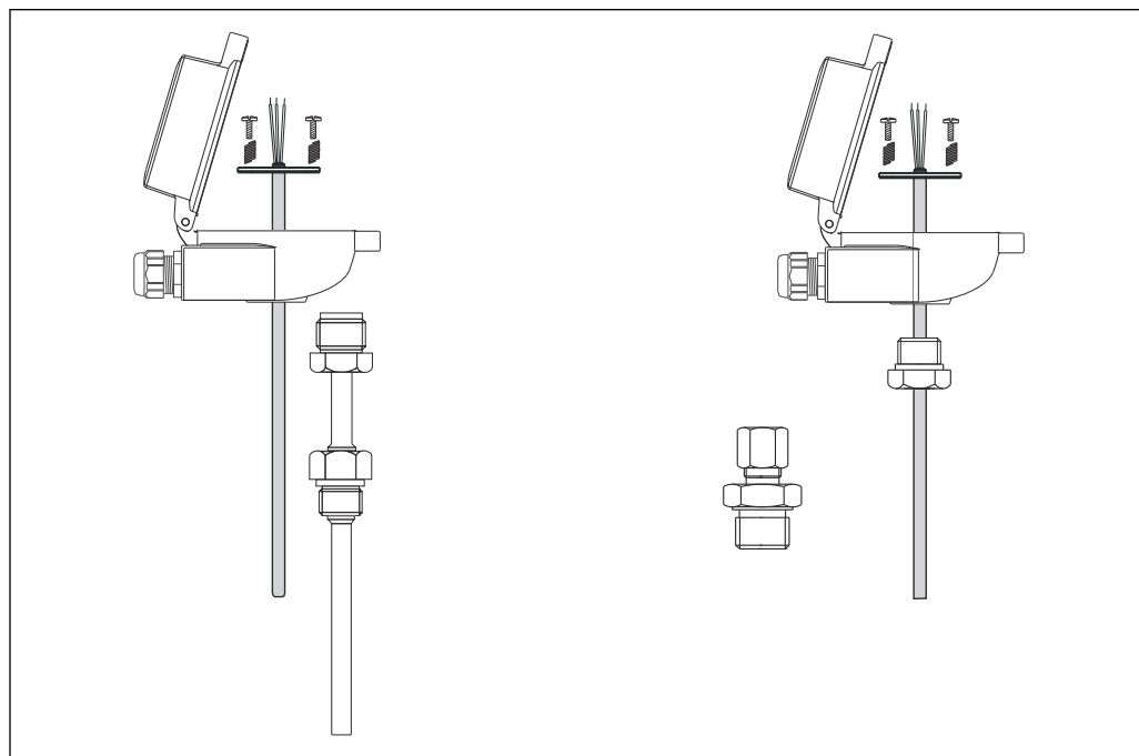
図 9 一般的な設置オプション：サーモウェル（左）、直接測定（右）のアセンブリ
