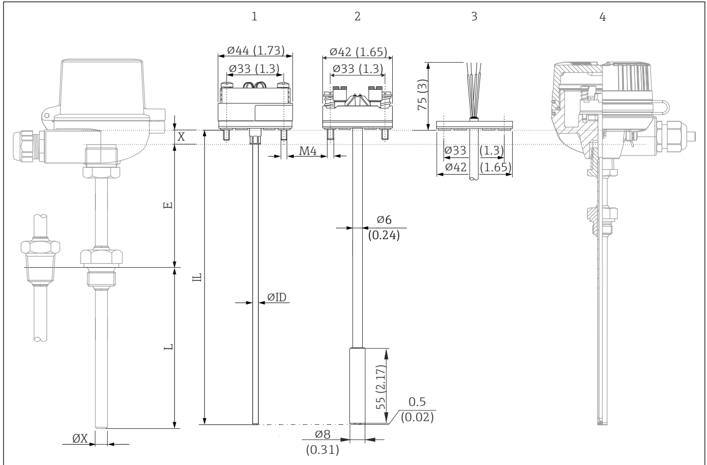
図 10 全寸法単位は mm (in) です。
