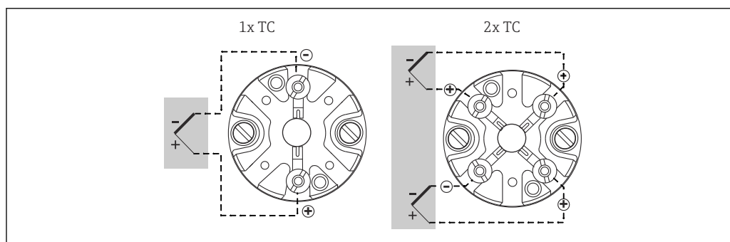
図 5 熱電対用のセラミック端子台
