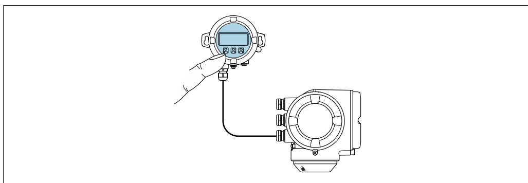
33 Управление с помощью блока выносного дисплея DKX001
