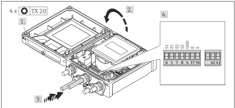
8 Messumformer: Hauptelektronikmodul mit Anschlussklemmen
