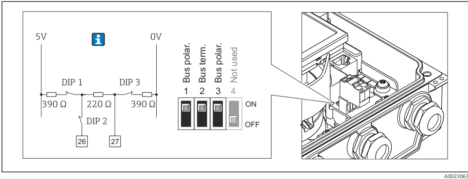
12 Terminierung mit Hilfe von DIP-Schaltern auf dem I/O-Elektronikmodul einstellen (bei Baudraten < 1,5 Mbaud)
