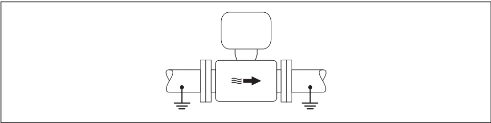
10 Potenzialausgleich über Messrohr
