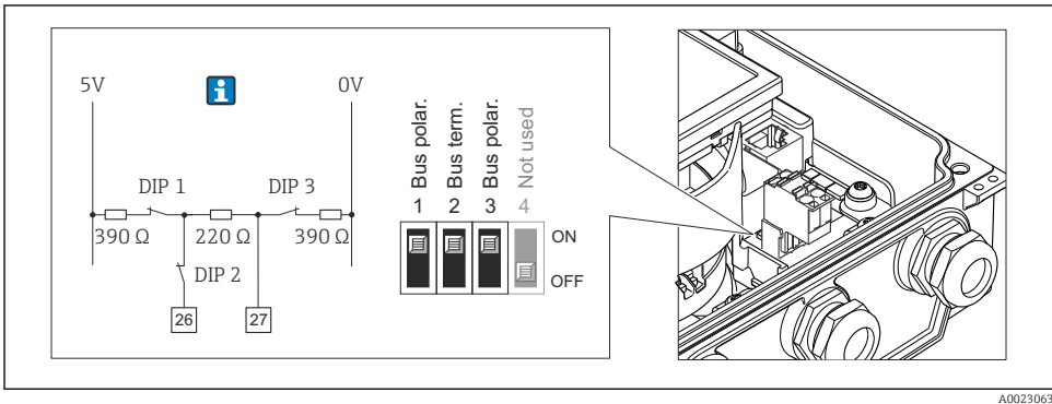
13 Abschlusswiderstand über DIP-Schalter auf Hauptelektronikmodul aktivierbar
