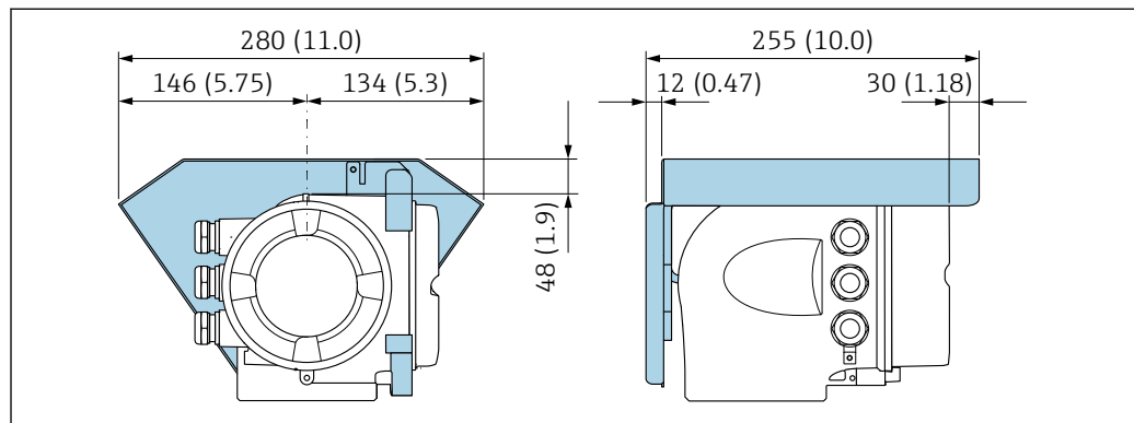
40 Tettuccio di protezione dalle intemperie per Proline 500 – unità ingegneristica mm (in)
