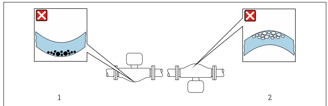
☒ 14 Orientamento del sensore con tubo di misura curvo
