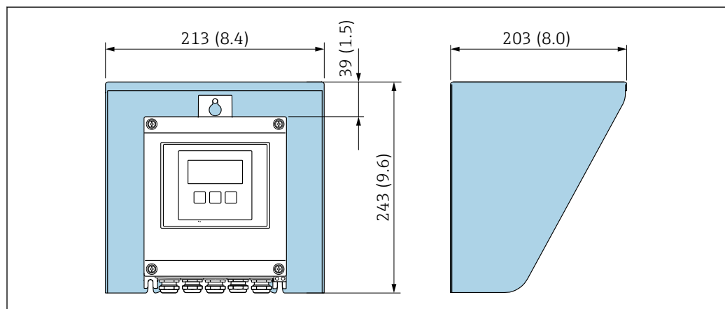
39 Tettuccio di protezione dalle intemperie per Proline 500 – digital; unità ingegneristica mm (in)
