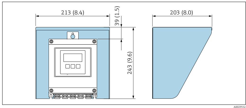
32 Tettuccio di protezione dalle intemperie per Proline 500 – digital; unità ingegneristica mm (in)
