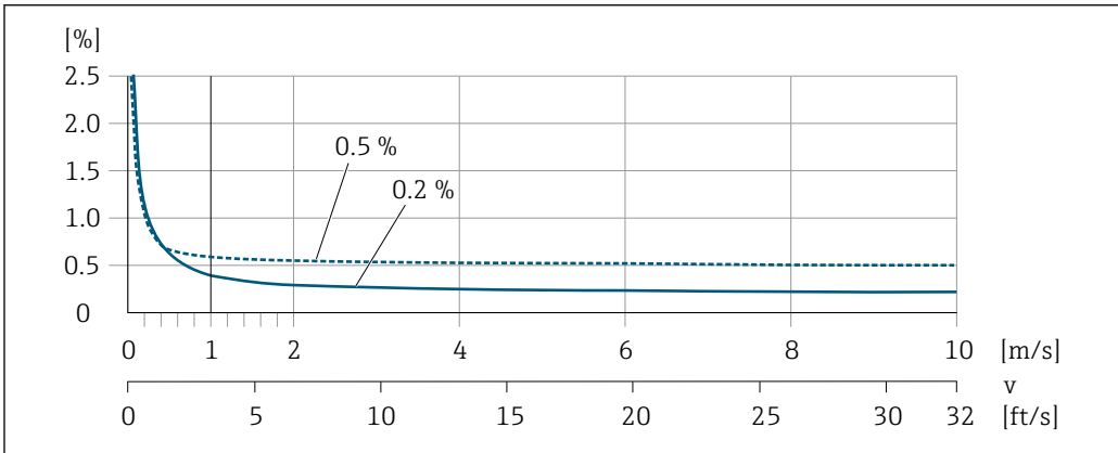
图 35 最大测量误差 (% o.r.)
