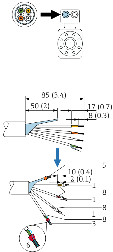
电极电缆
