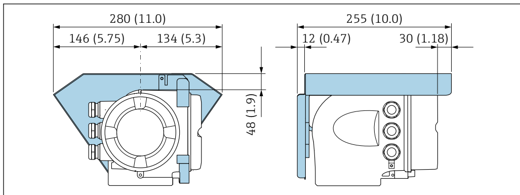
图 8 防护罩 (Proline 500) ; 单位: mm (in)
