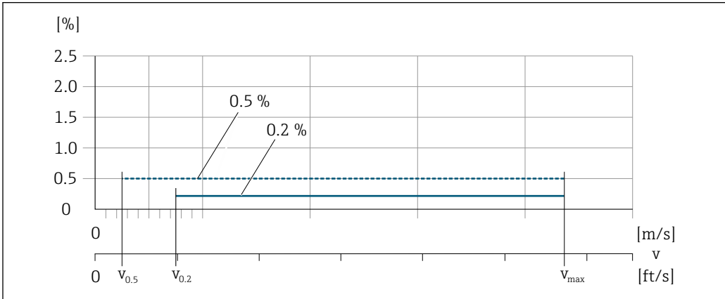
图 36 设计测量精度 (% o.r.)
