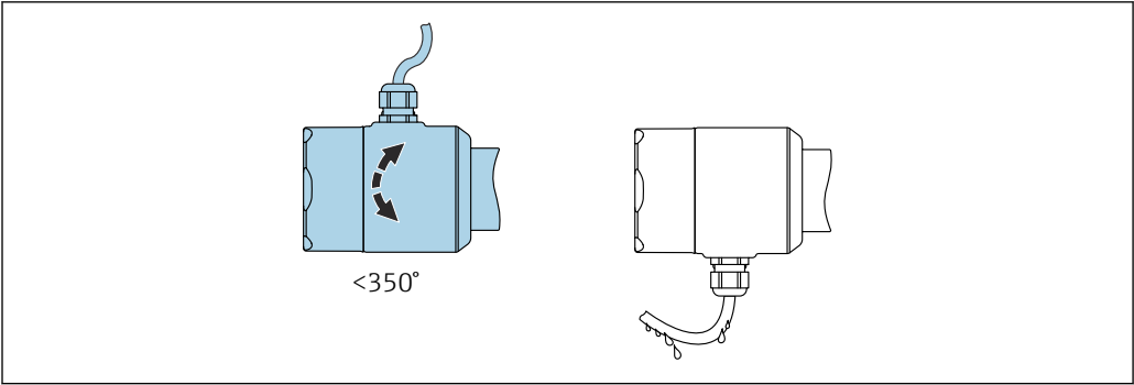
图 17 外壳不带固定螺丝；在电缆上建立排水回路。
