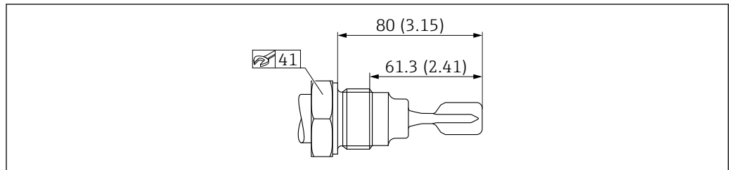
36 ISO228 G 1 螺纹。测量单位 mm (in)
