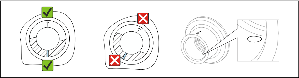
图 21 焊座，带泄漏检测孔
