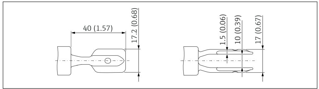
图 33 叉体。测量单位 mm (in)
