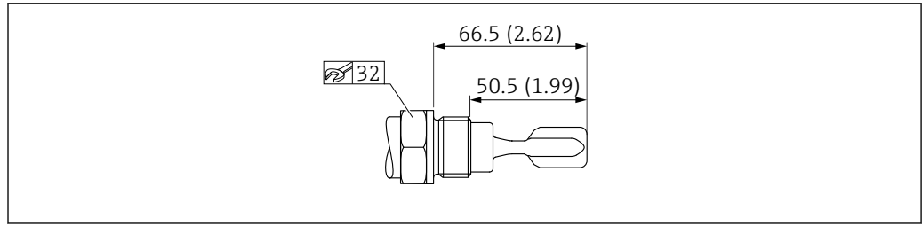
35 ISO228 G 3/4 螺纹。测量单位 mm (in)
