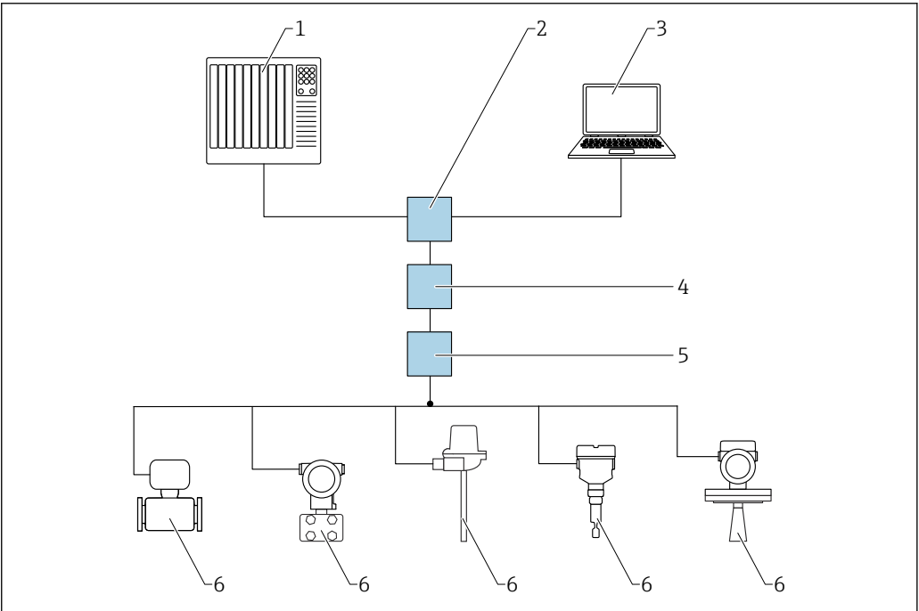
47 通过 PROFINET + Ethernet-APL 网络实现远程操作: 星形拓扑结构
