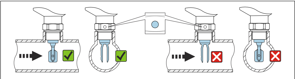
16 安装在管道中（注意叉体安装位置和标记）
