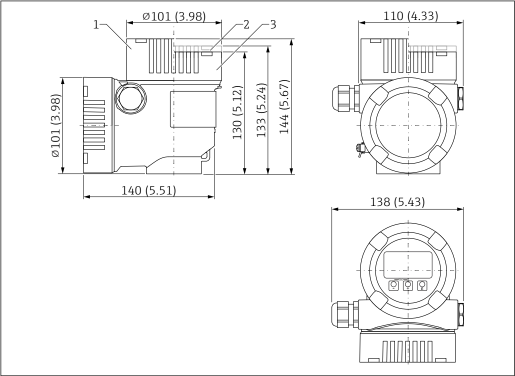
图 29 双腔体 L 型铝外壳（带涂层）的外形尺寸示意图。测量单位 mm (in)
