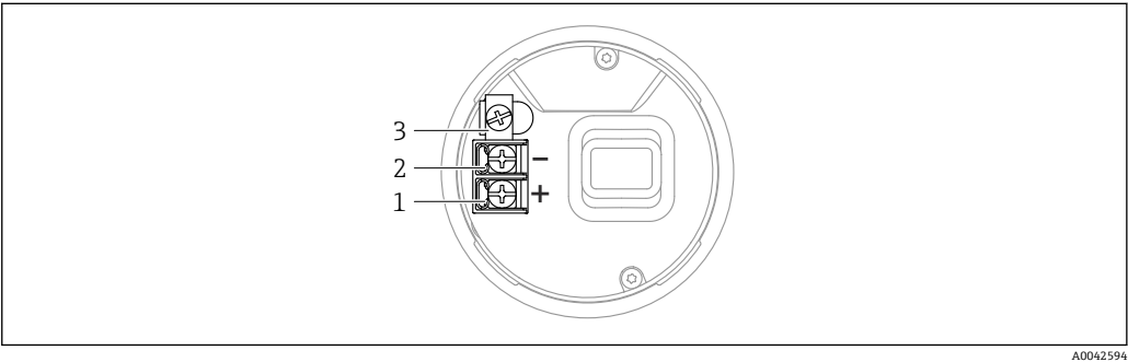
图 2 接线腔内的接线端子和接地端，单腔室外壳
