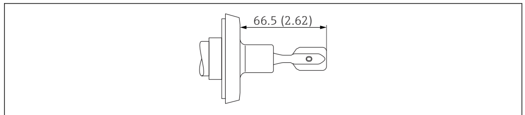
39 DIN11851 管接头。测量单位 mm (in)
