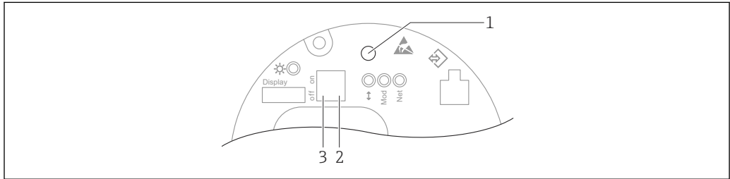
图 44 Ethernet-APL 通信型电子插件（FEL60P）上的操作按键和 DIP 开关
