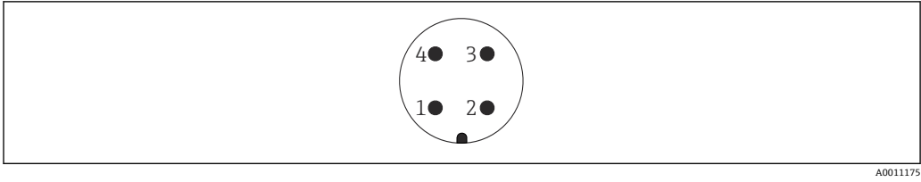
图 4 设备接线示意图
