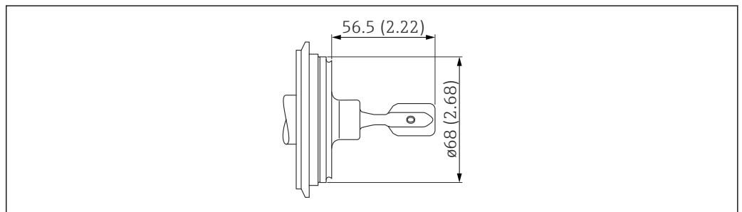
40 Varivent N 型接头, DN65-162 PN25 配合管道。测量单位 mm (in)
