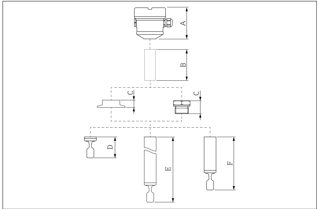
图 25 计算设备高度所需考虑的部件
