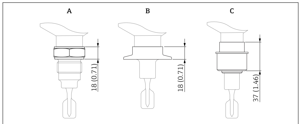
图 34 过程连接的最大高度规格。测量单位 mm (in)
