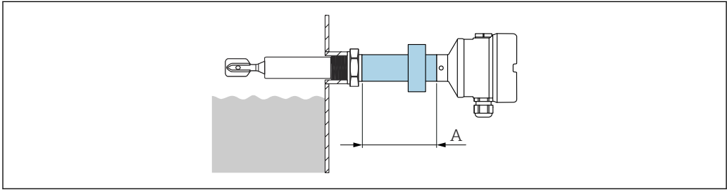
图 30 隔爆玻璃馈通（搭配延长管使用）
