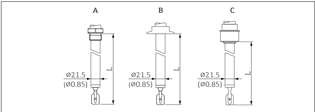
图 32 探头类型：延长管型、短管型（传感器长度 L）。测量单位 mm (in)
